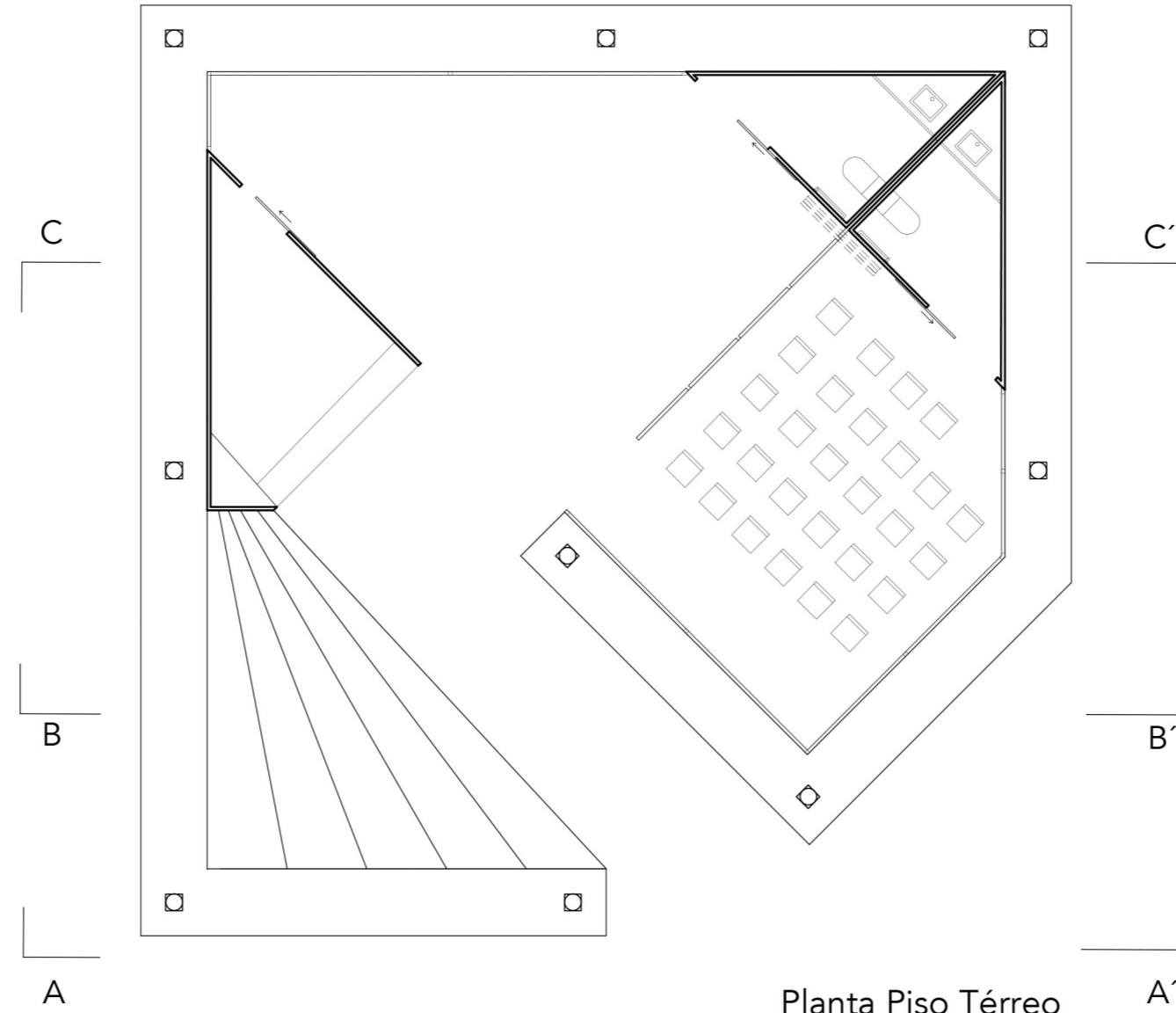
Planta Piso Térreo Esc. 1/100
