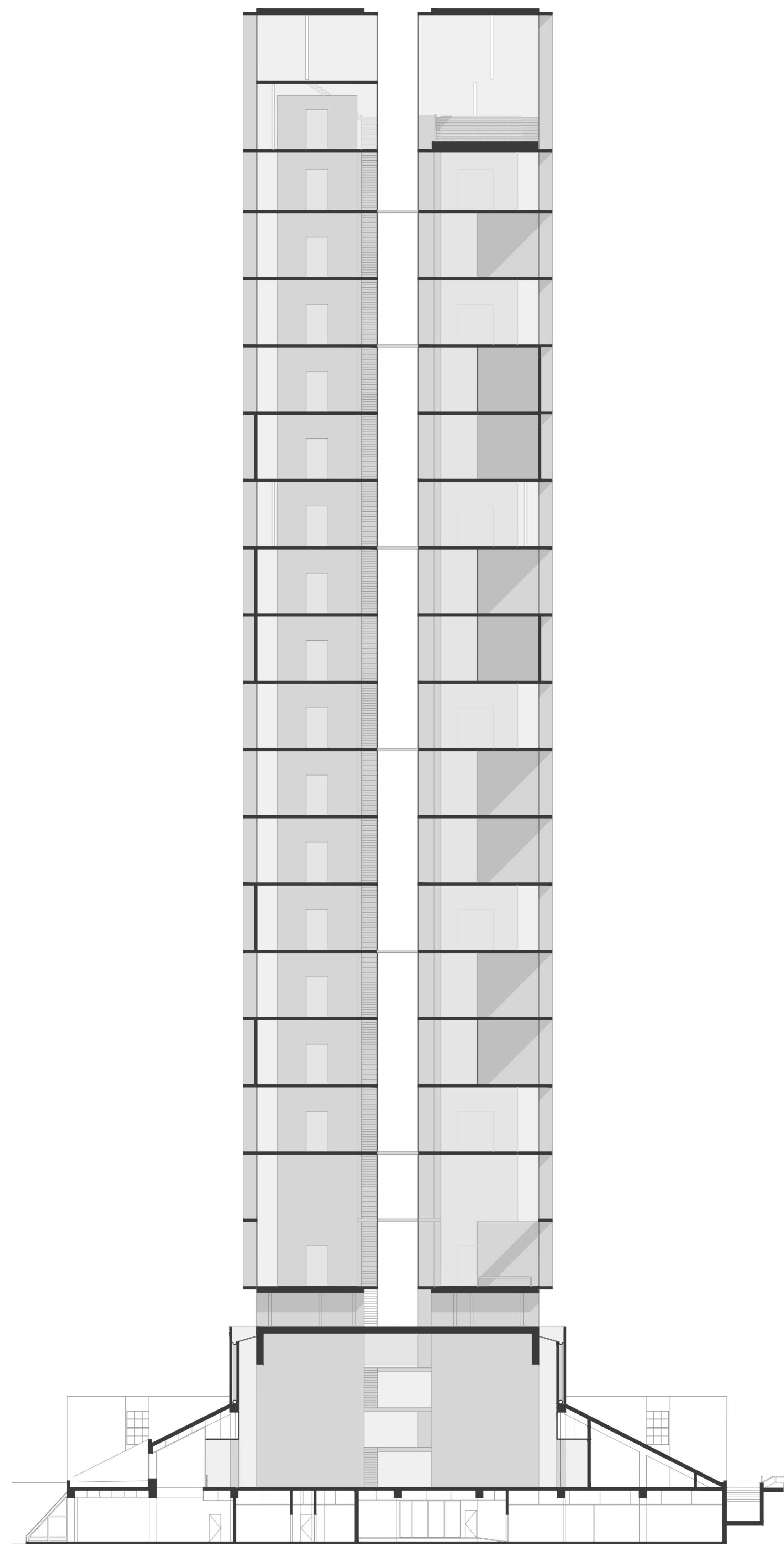
Corte Vertical (Nascente-Poente)
