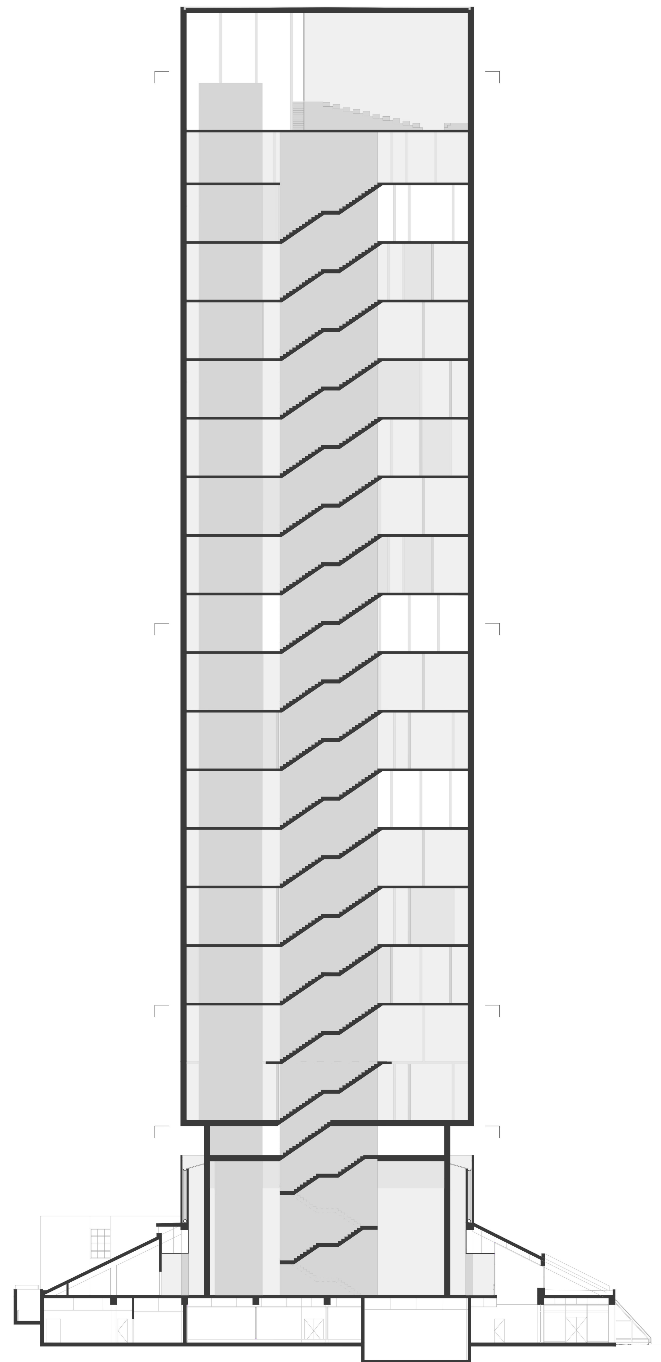
Corte Vertical (Norte-Sul)
