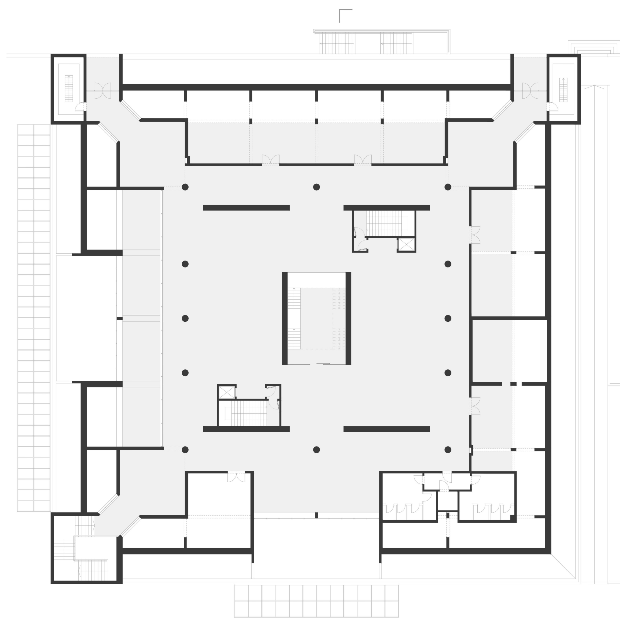
planta de piso térreo (átrio de entrada)
