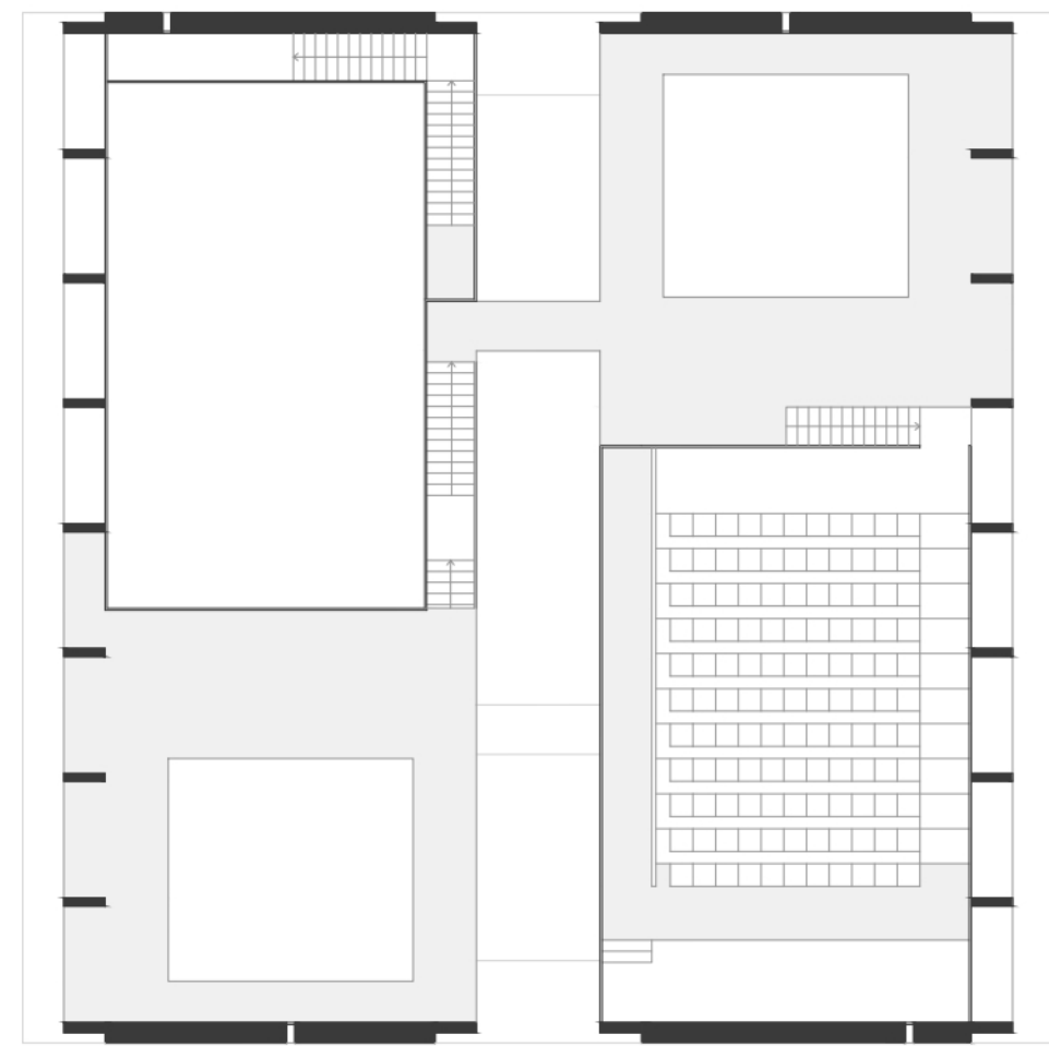
auditório e sala de exposições
