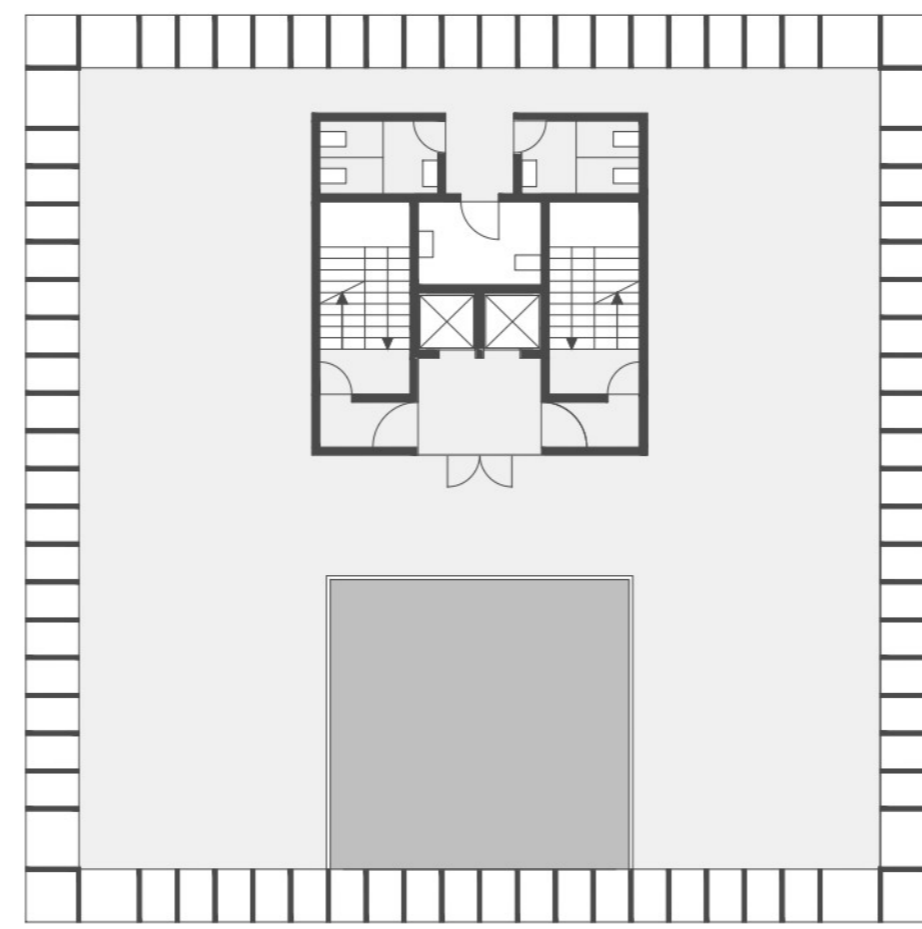
último piso | terraço
