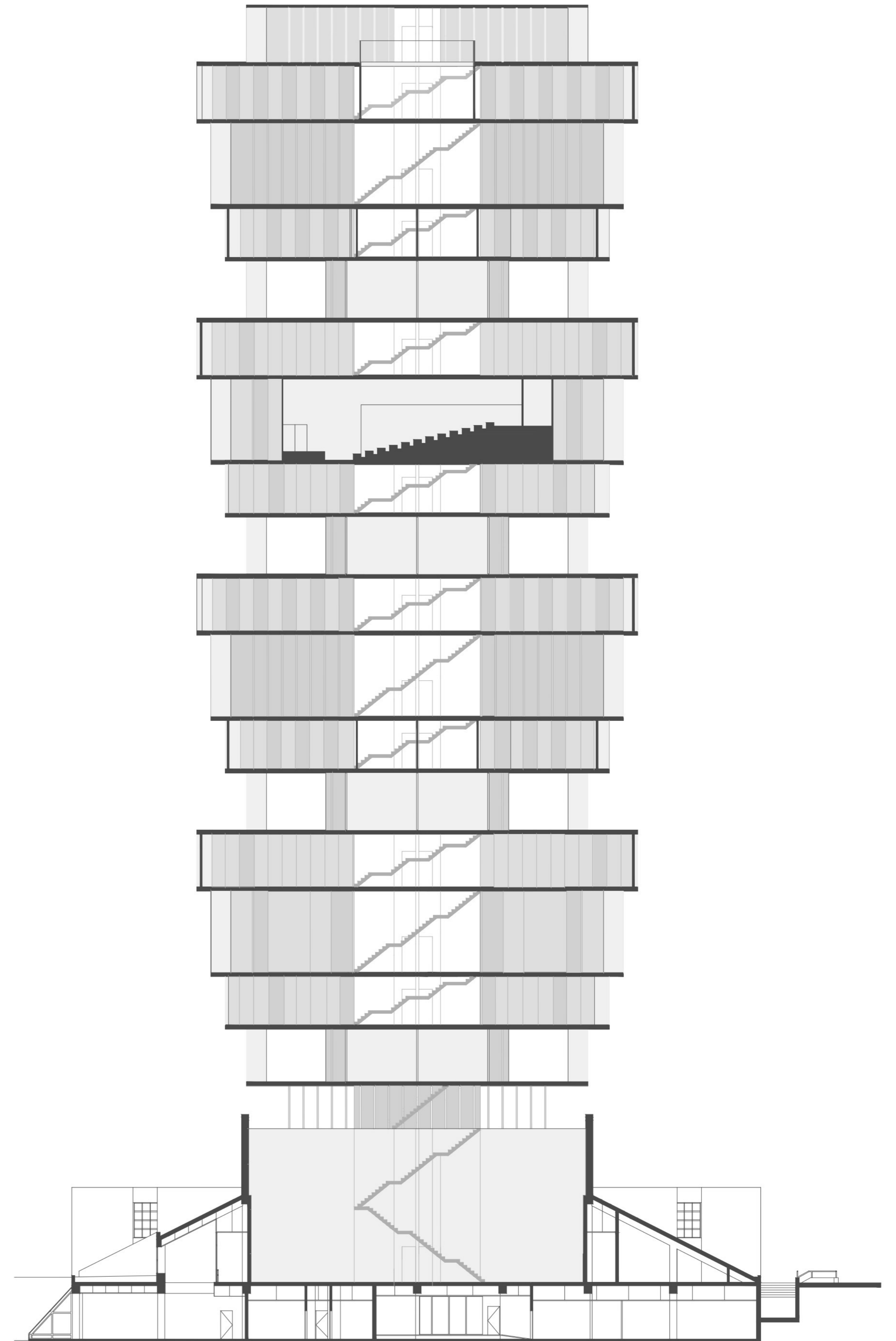
CUBO - CORTE BB • ESCALA 1:200
