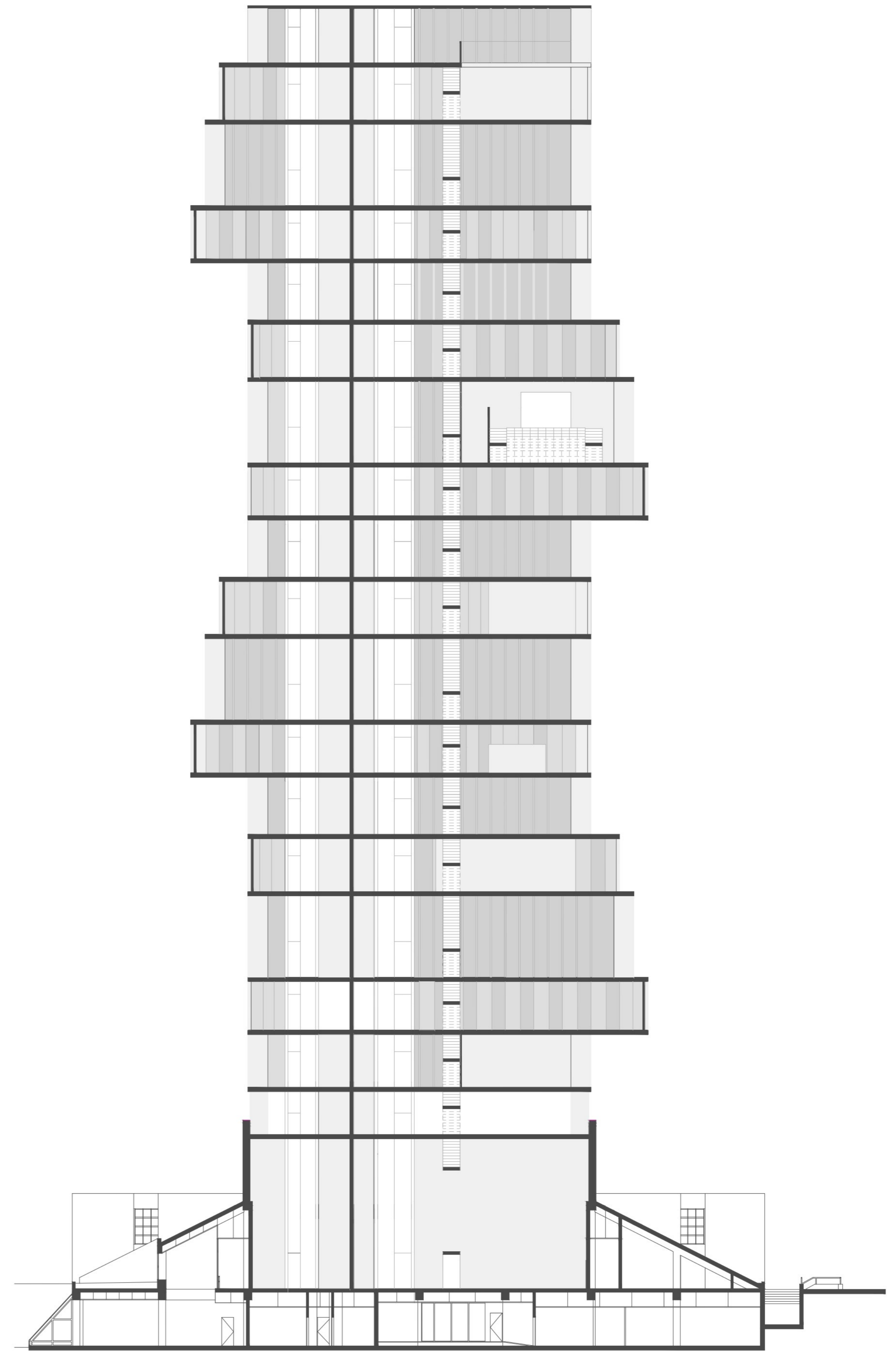
CUBO - CORTE AA' - ESCALA 1:200
