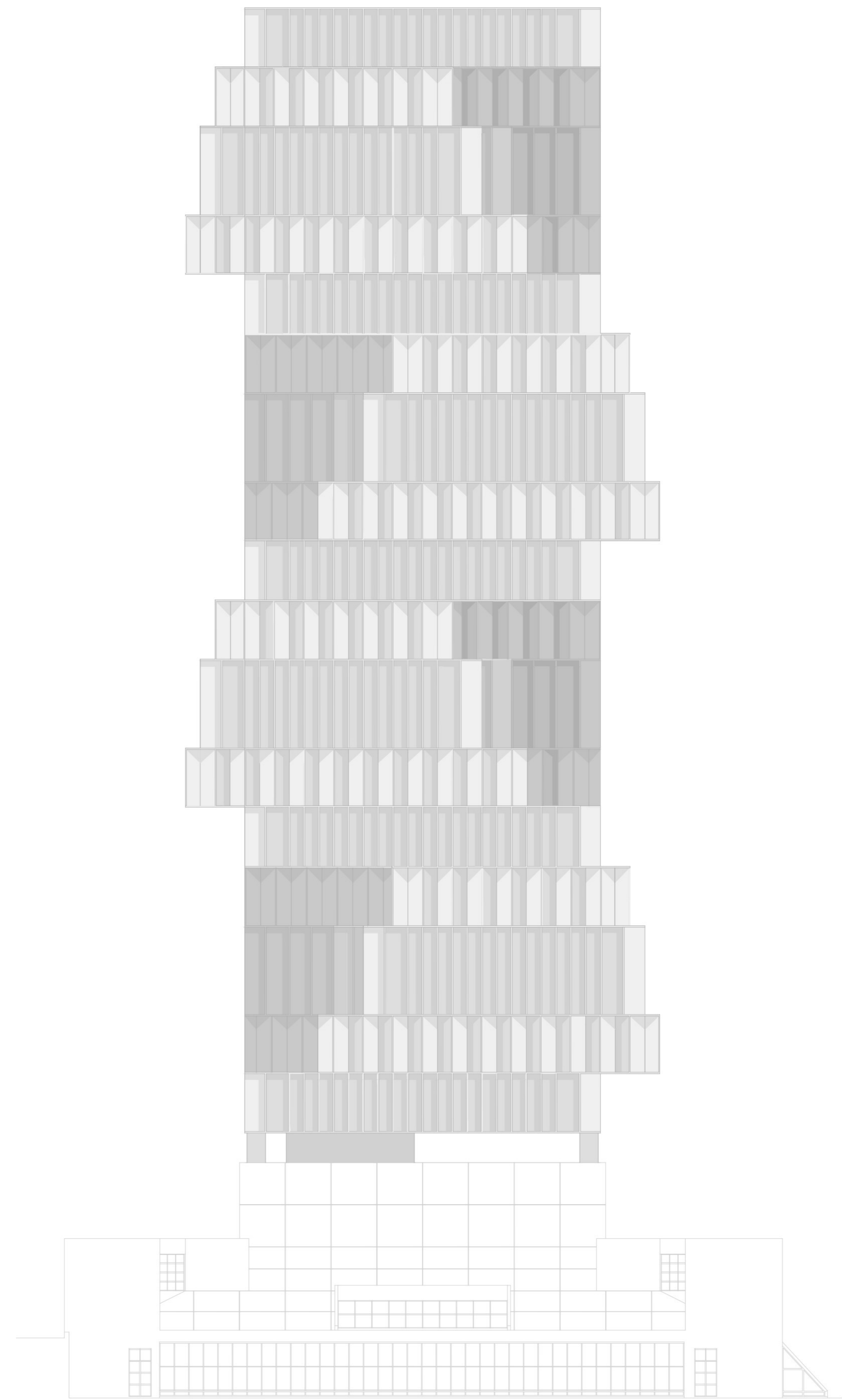
CUBO - ALÇADO POENTE • ESCALA 1:200
