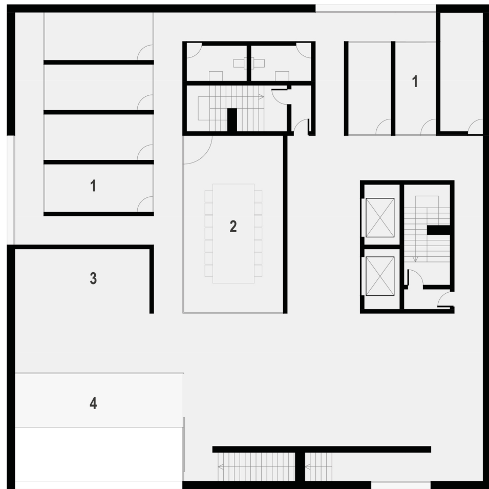
PROFESSORES + BAR PLANTA TORRE PISO 8
