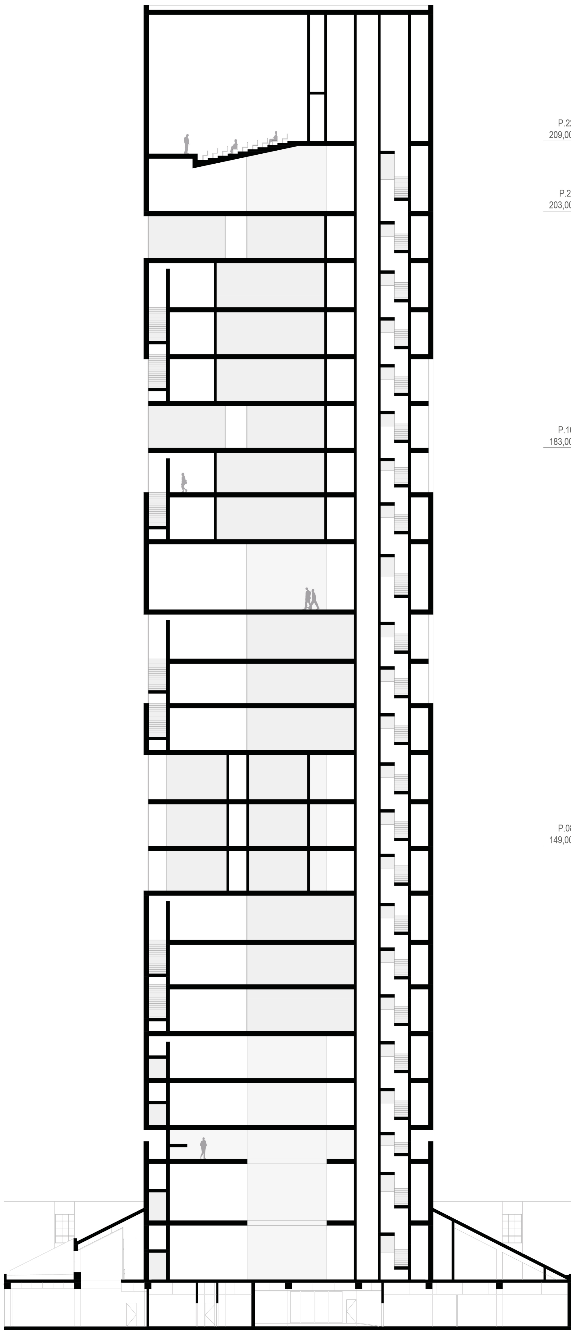
CORTE BB'
