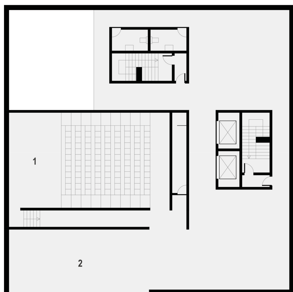
ÁTRIO + AUDITÓRIO PLANTA TORRE PISO 22
