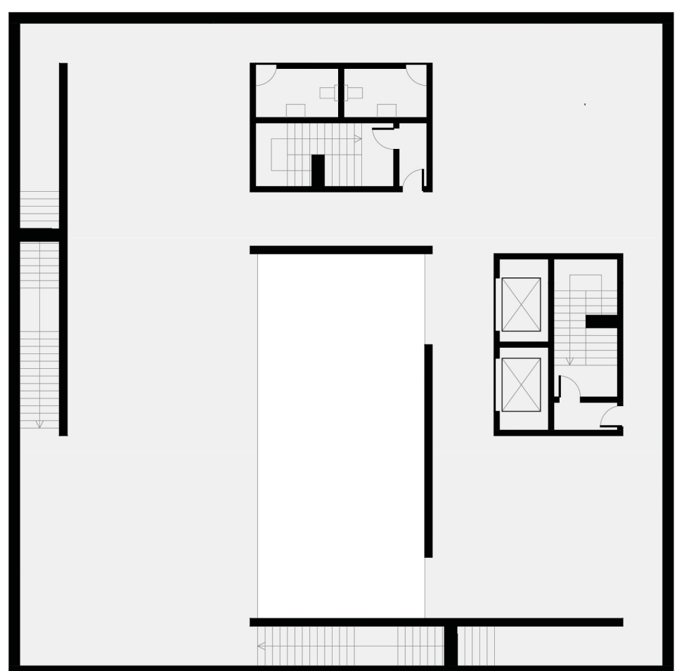
PLANTA CUBO PISO 1
