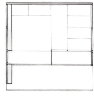
CORTE CC'
