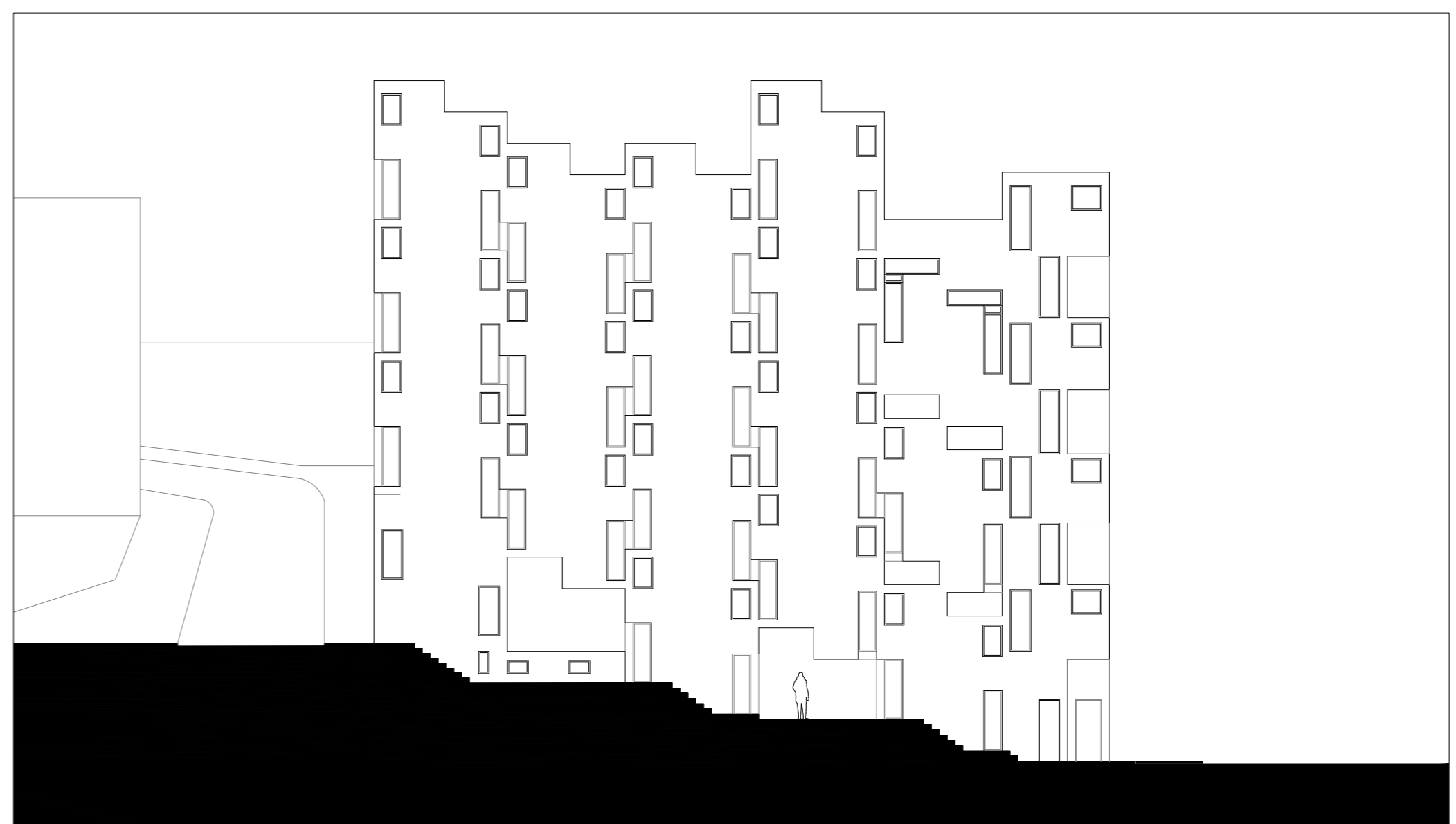
ALÇADO NORTE CC' | ESC. 1:200
