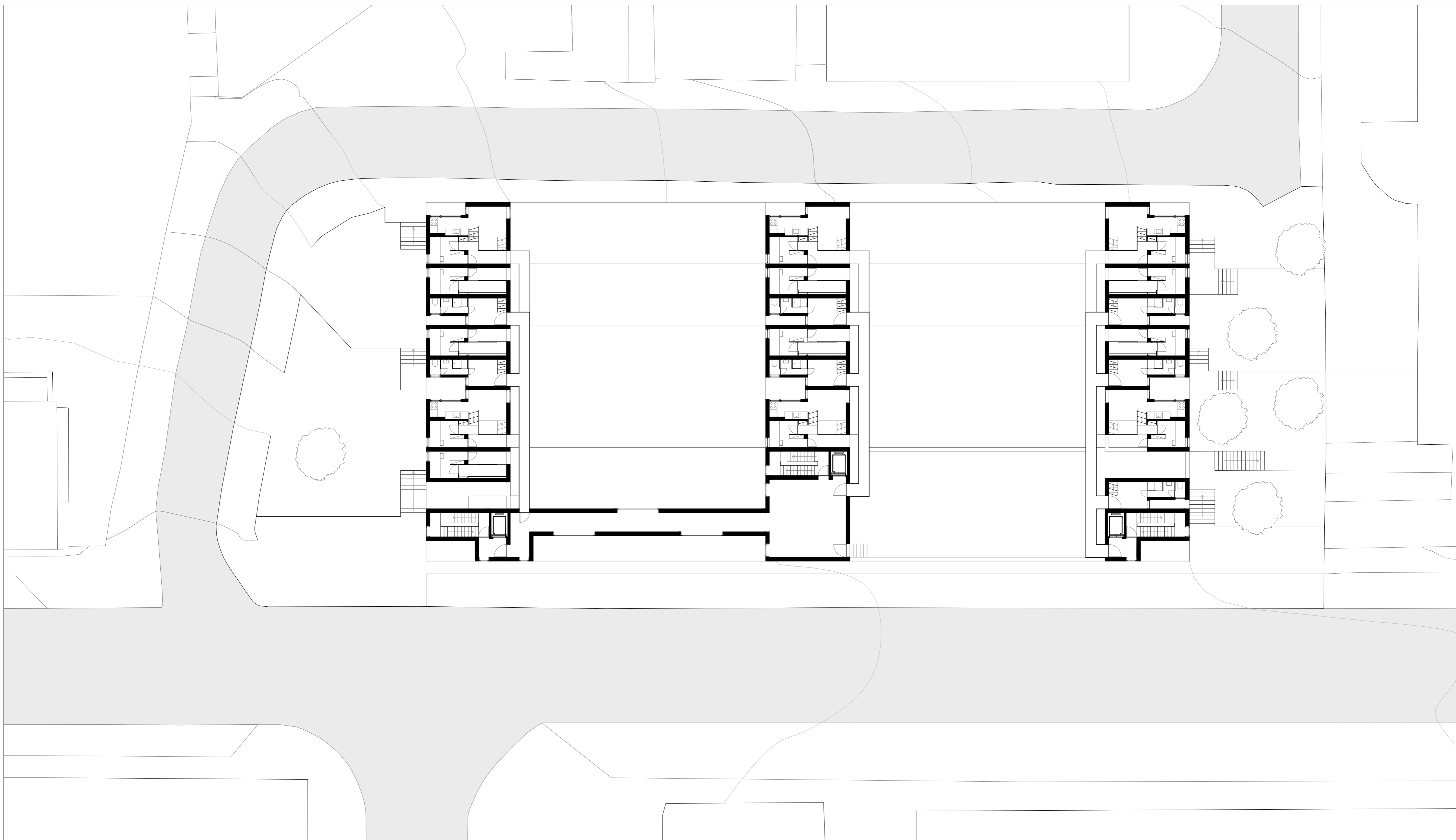
PLANTA – PISO 4 DE PROTÓTIPOS; LIGAÇÃO HORIZONTAL AÉREA; COBERTURA DA SALA POLIVALENTE | ESC. 1:200
