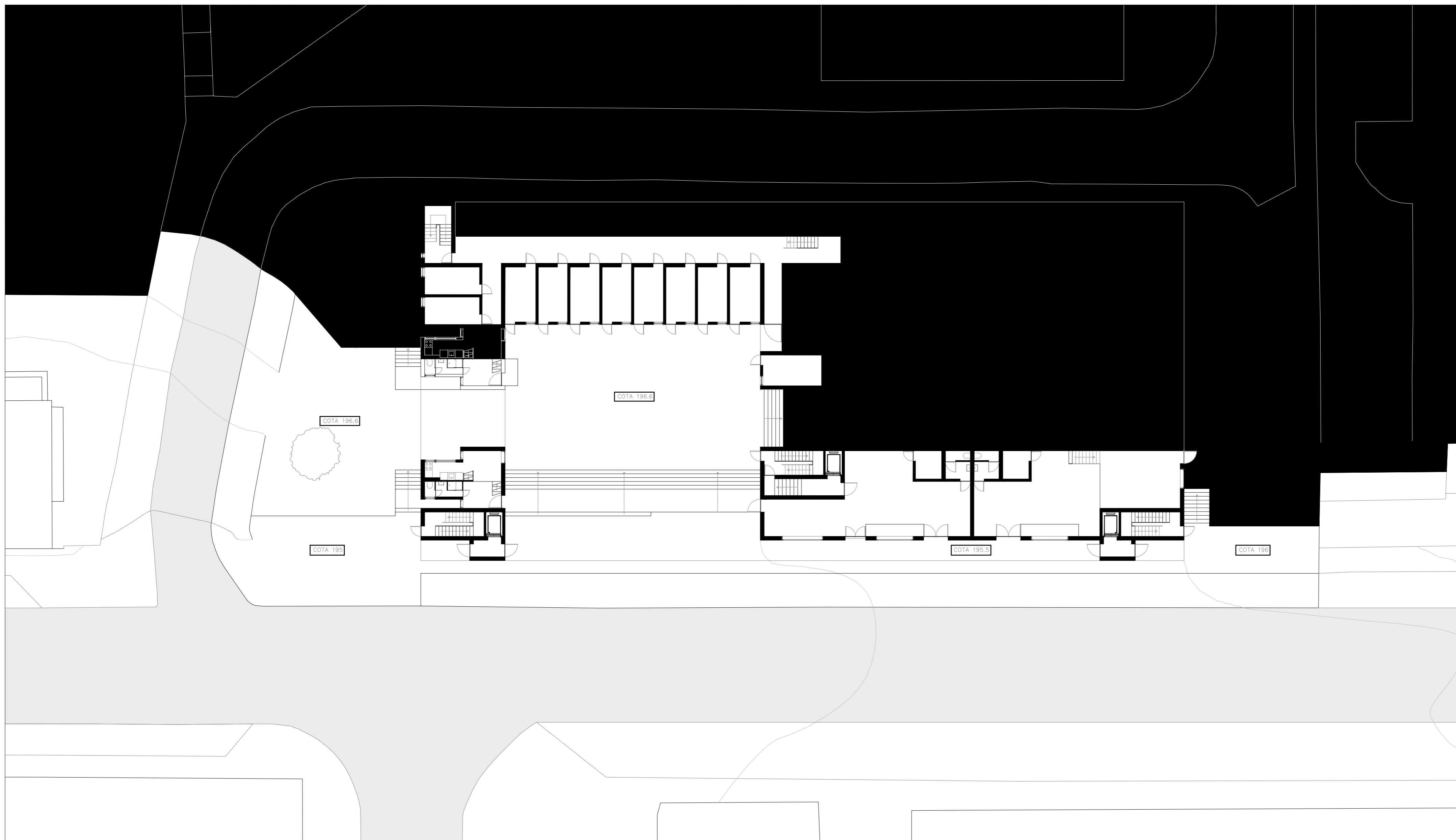
PLANTA CORTADA À COTA 198 – PISO TÉRREO (ZONA COMERCIAL; ARRUMOS/ESPAÇO DE TRABALHO) | ESC. 1:200
