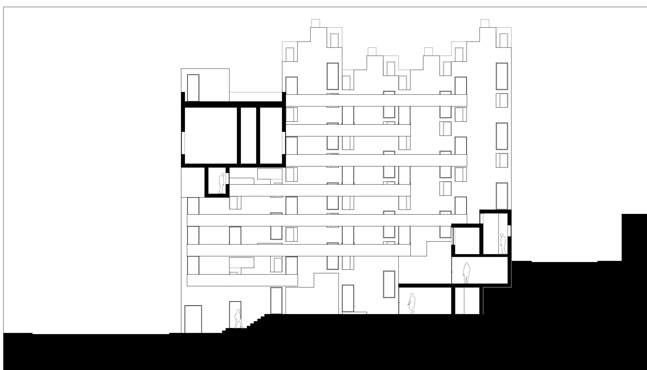
CORTE TRANSVERSAL BB' | ESC. 1:200
