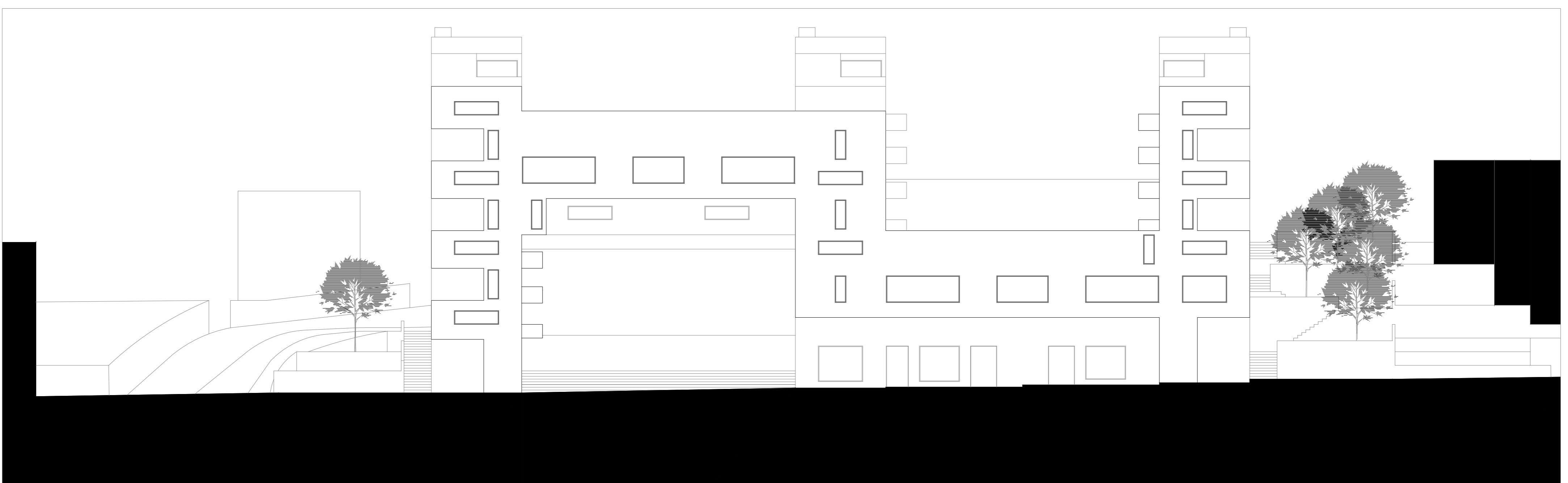
ALÇADO DA RUA DR. FELIX ALVES PEREIRA GG' | ESC. 1:200
