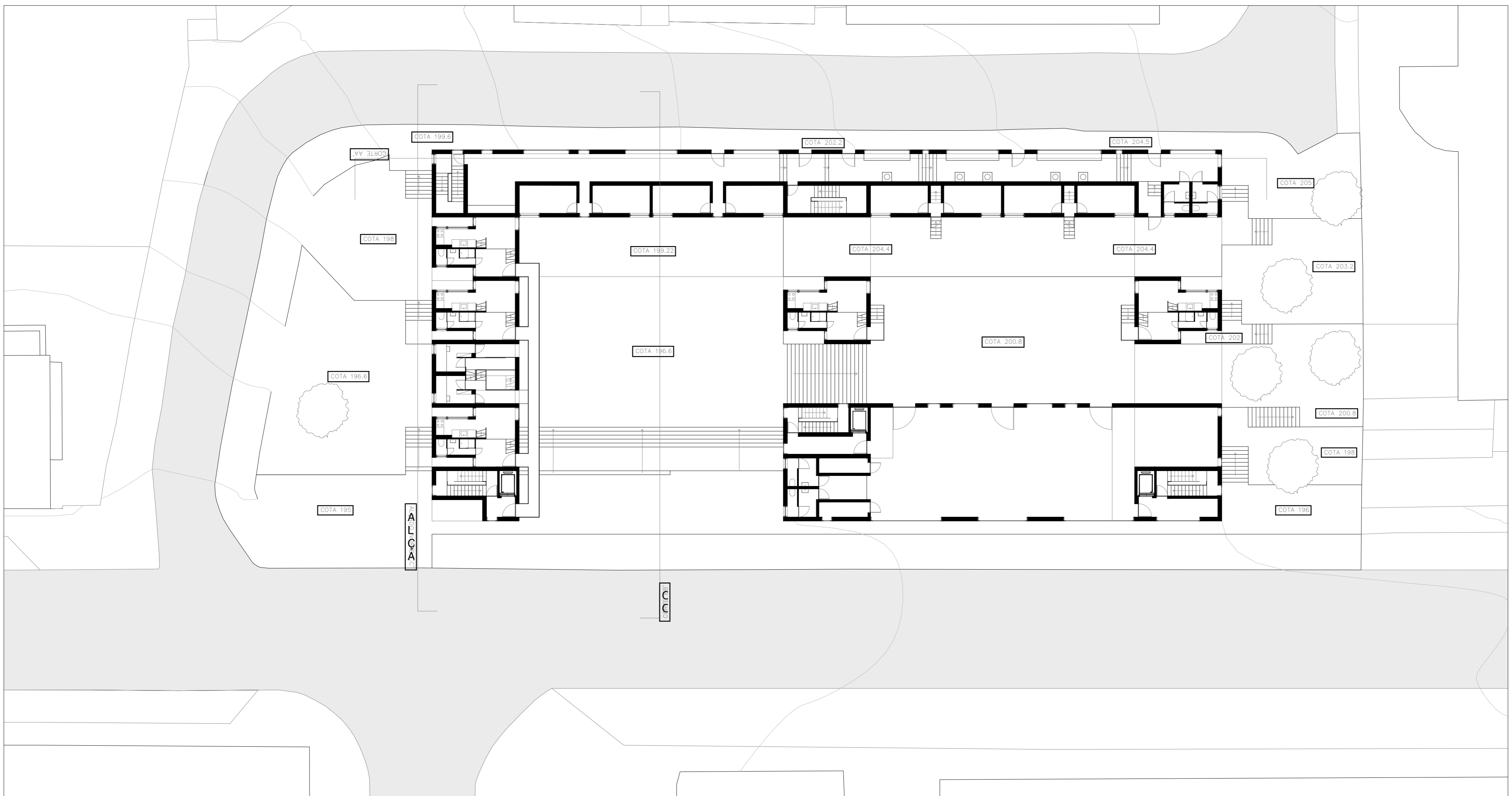
PLANTA CORTADA À COTA 206 – PISO 2 DE PROTÓTIPOS; LAVANDARIA; ARRUMOS/ESPAÇO DE TRABALHO; SALA POLIVALENTE | ESC. 1:200
