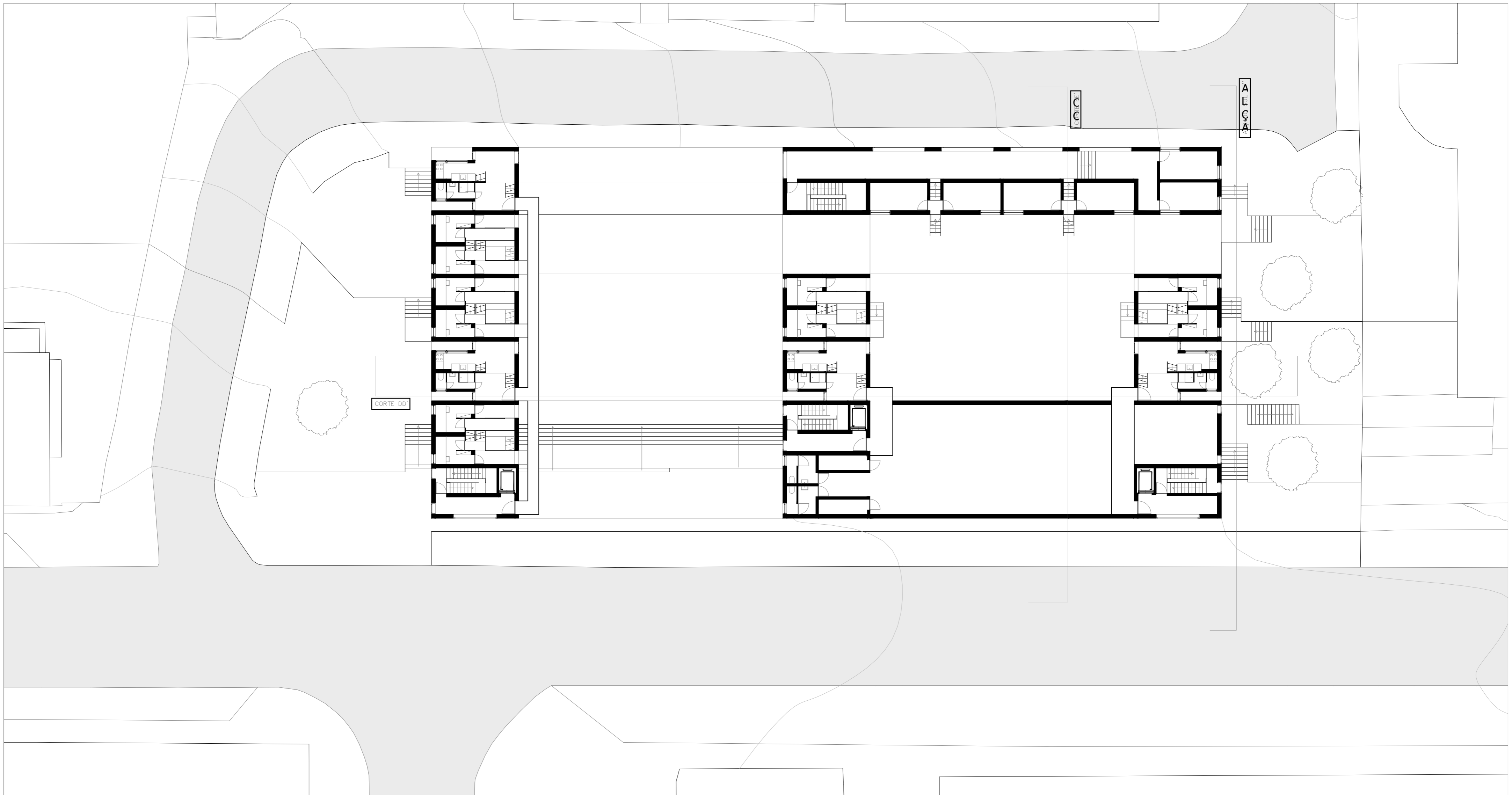
PLANTA – PISO 3 DE PROTÓTIPOS; ÚLTIMO PISO DE ARRUMOS/ESPAÇO DE TRABALHO; SALA POLIVALENTE | ESC. 1:200
