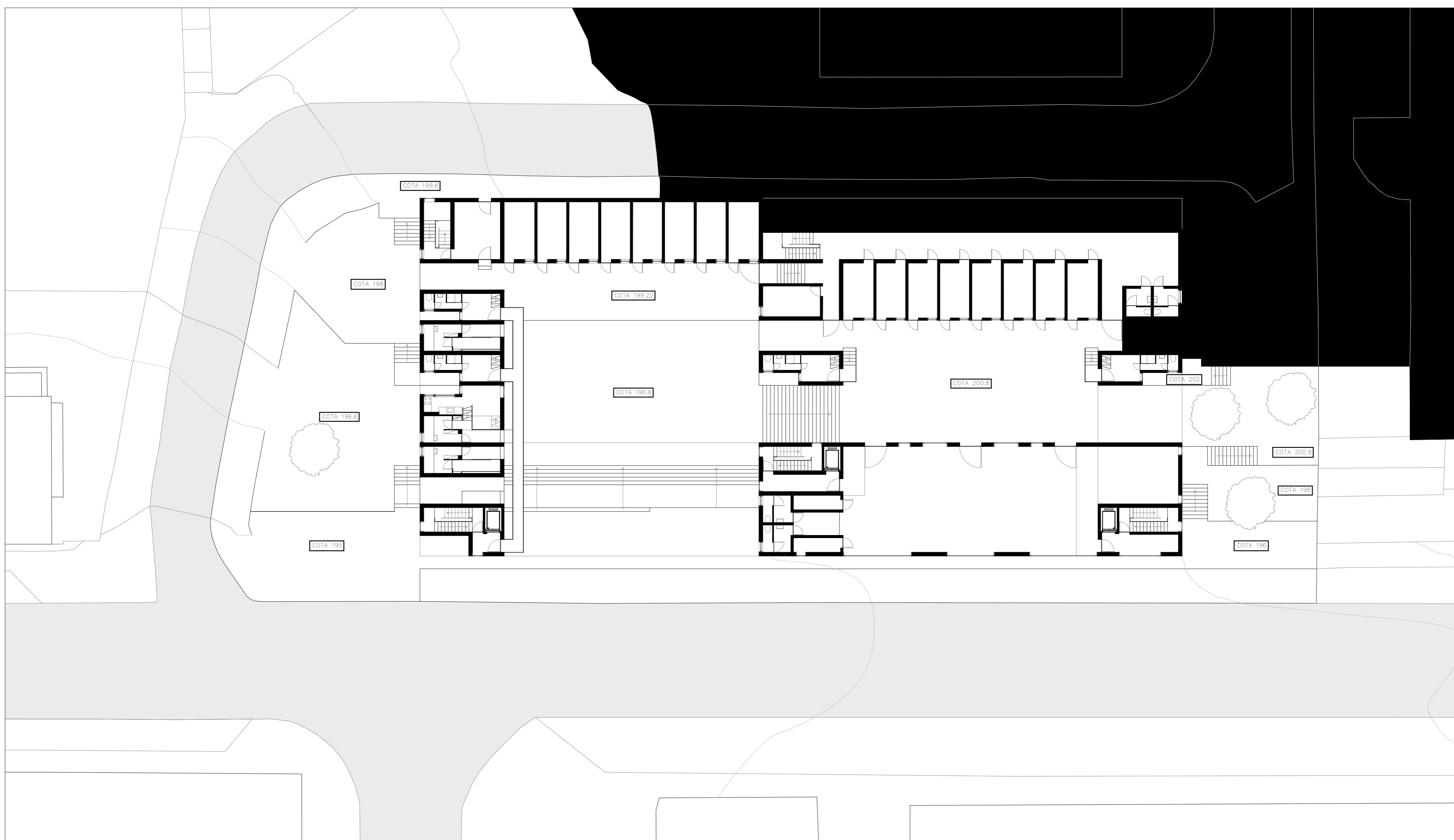
PLANTA CORTADA À COTA 202.2 – PISO 1 DE PROTÓTIPOS; SALA POLIVALENTE; ARRUMOS/ESPAÇO DE TRABALHO | ESC. 1:200
