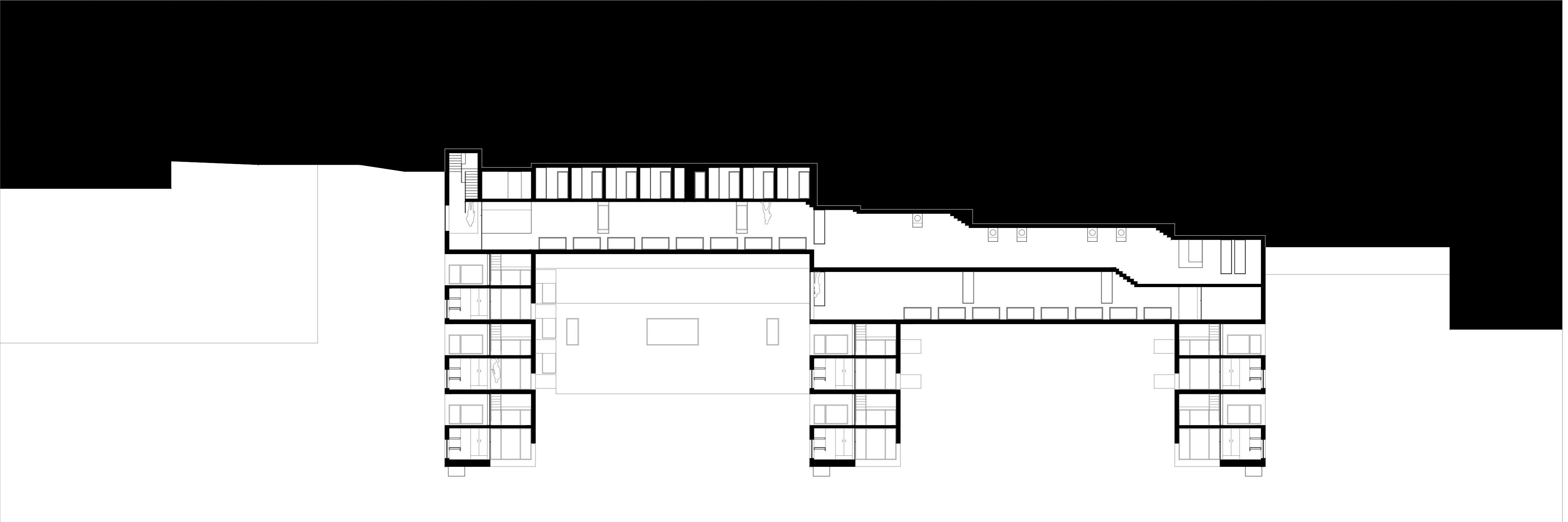
CORTE LONGITUDINAL AA' | ESC. 1:200
