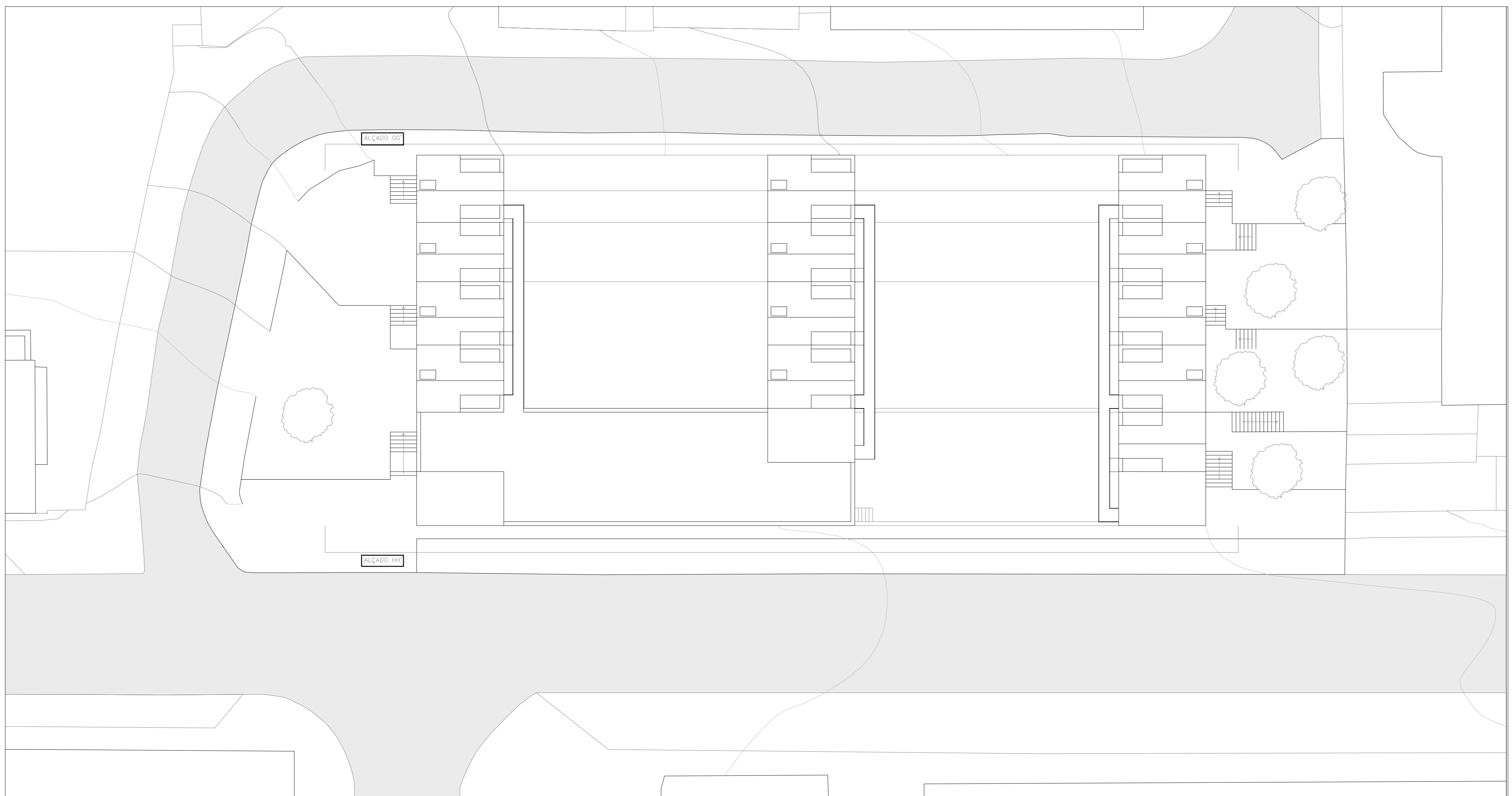
PLANTA DA COBERTURA | ESC. 1:200
