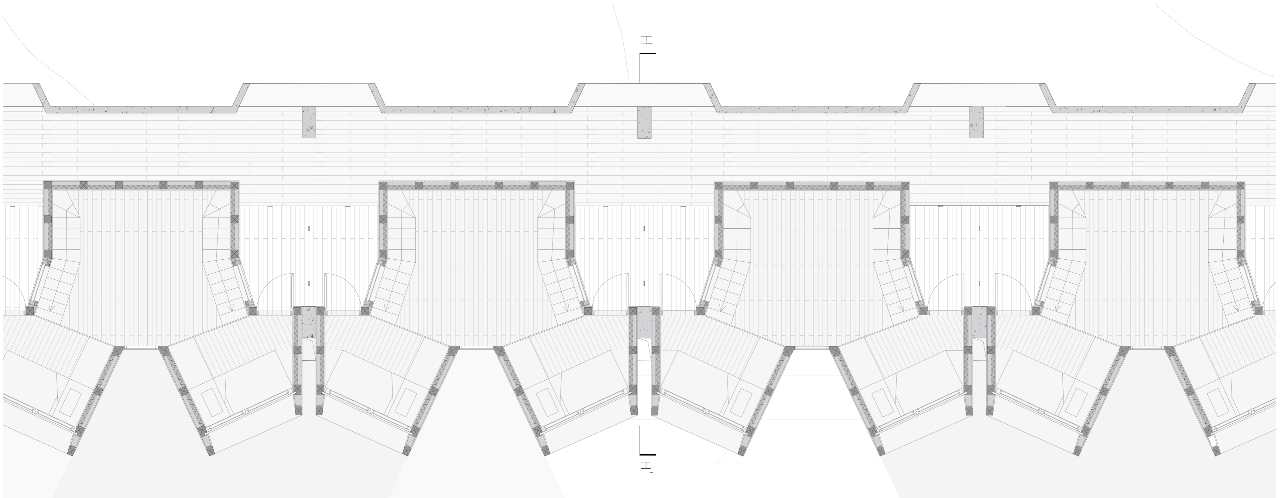
PLANTA PROTÓTIPOS PISO 1 | ESC. 1:50
