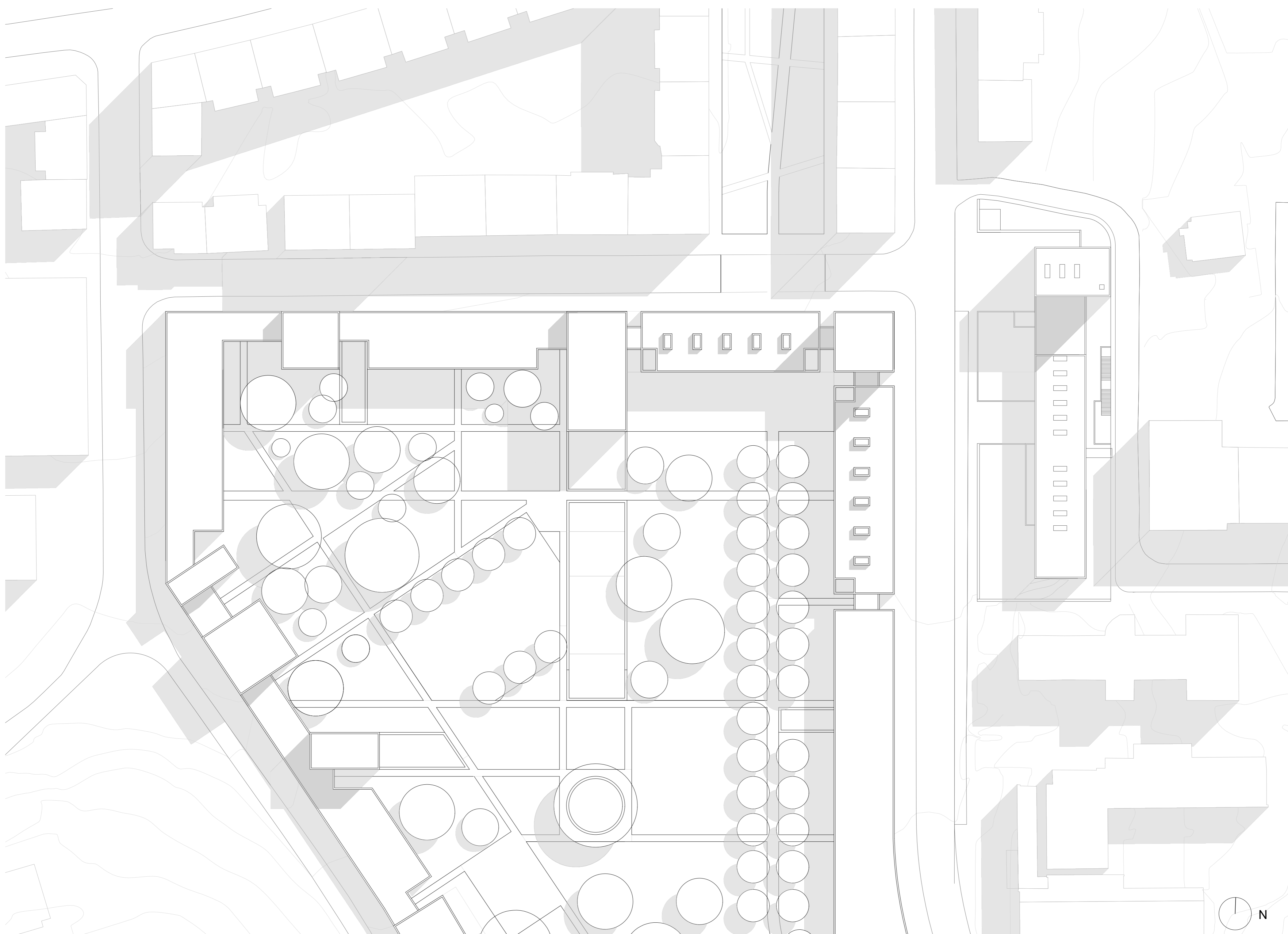
planta geral de enquadramento | escala 1:500
