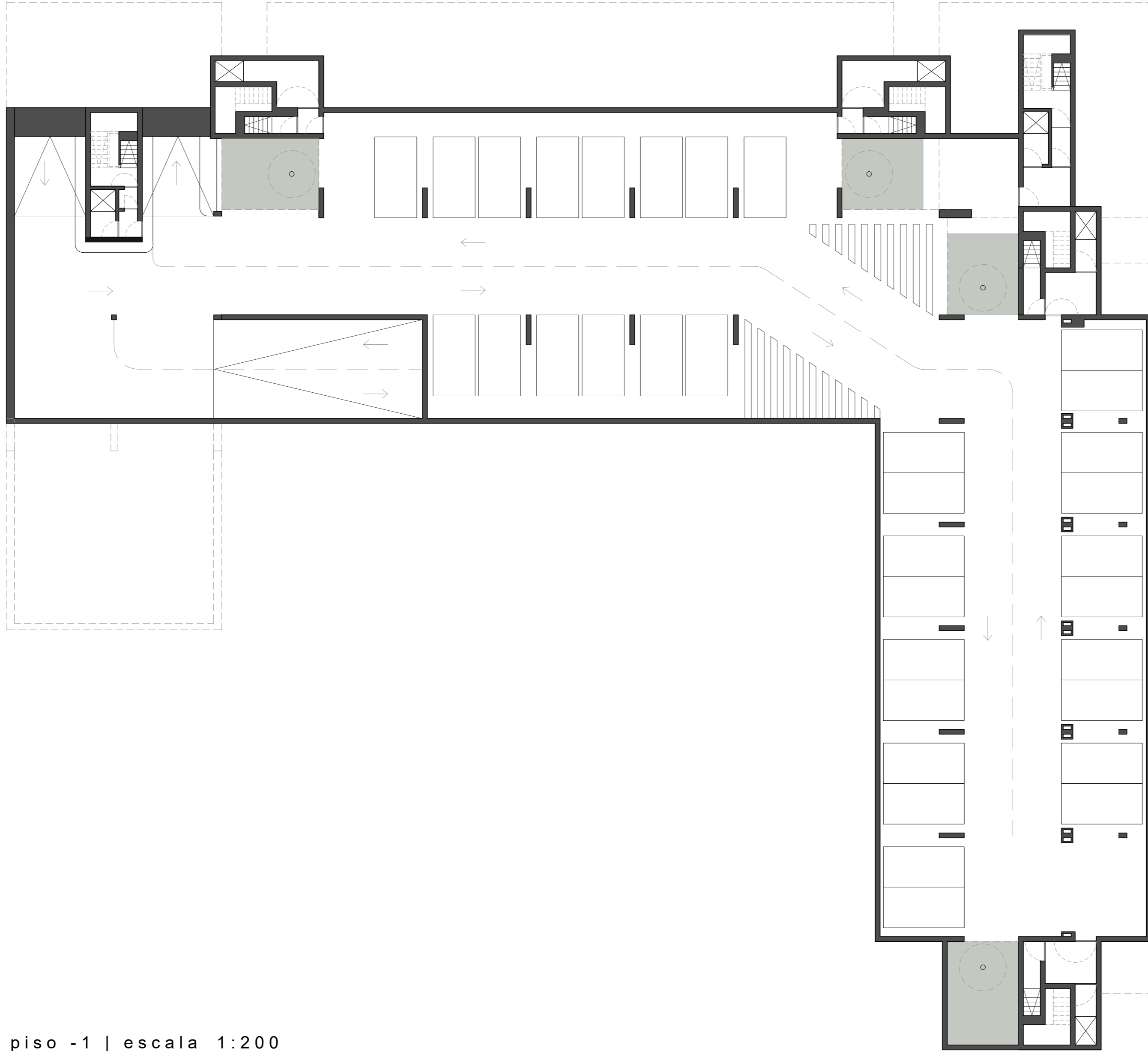
planta estacionamento | piso -1 | escala 1:200
