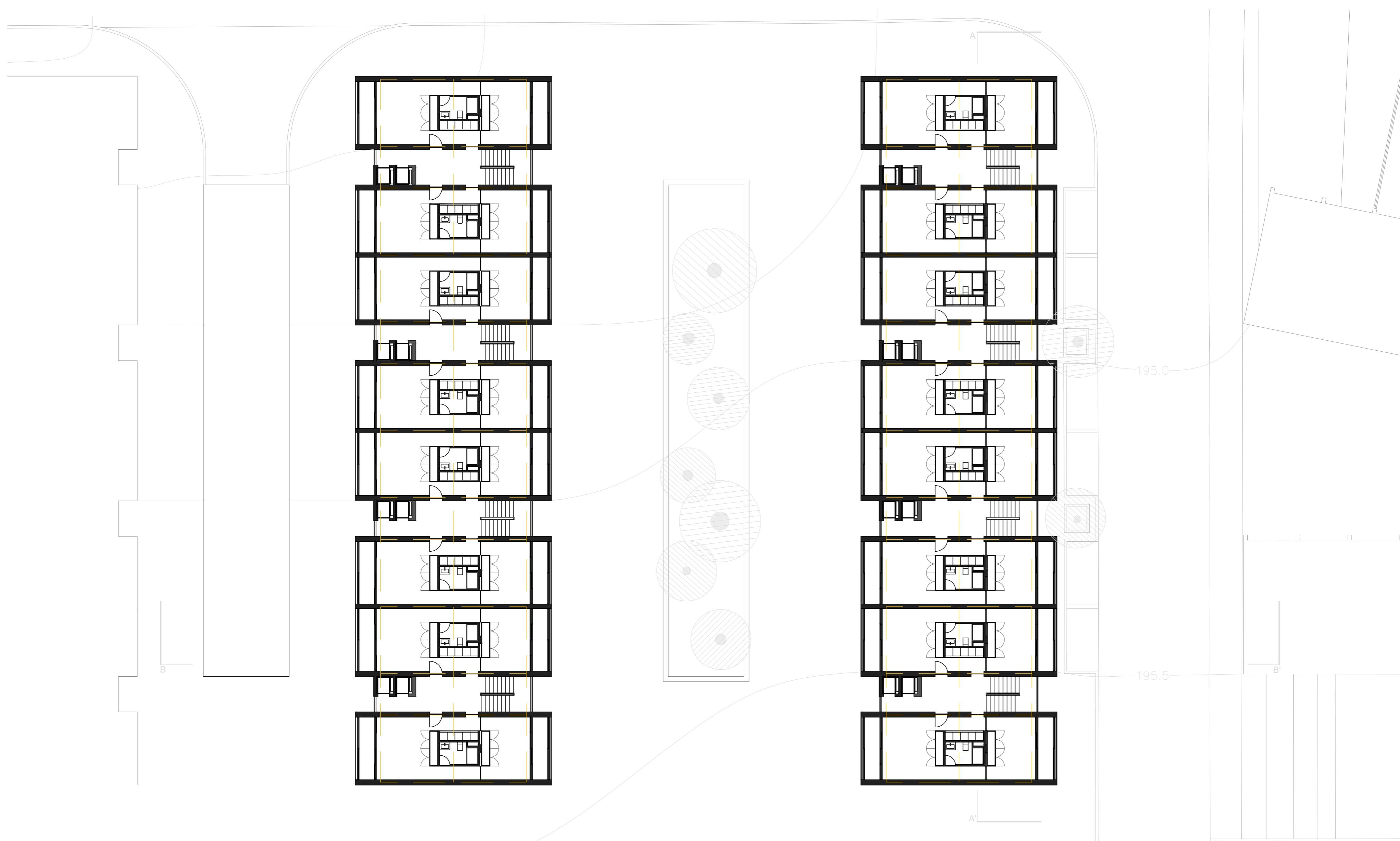
ESC. 1/200 | PLANTA PISO TIPO
