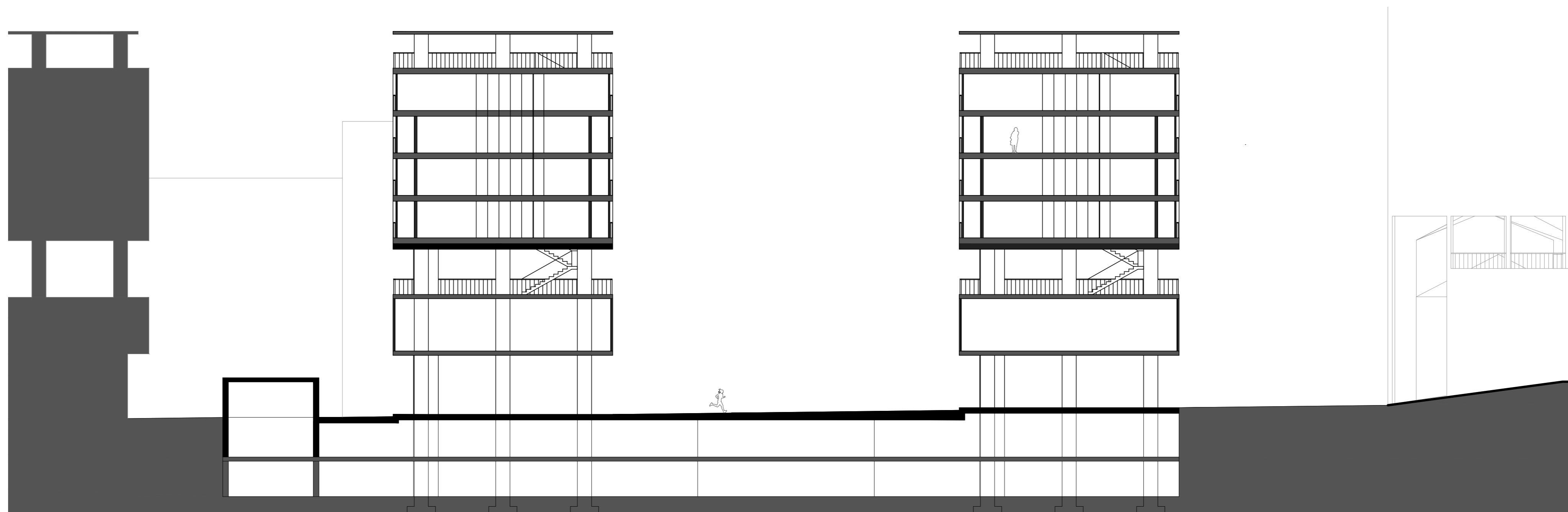
PERFIL TRANSVERSAL
