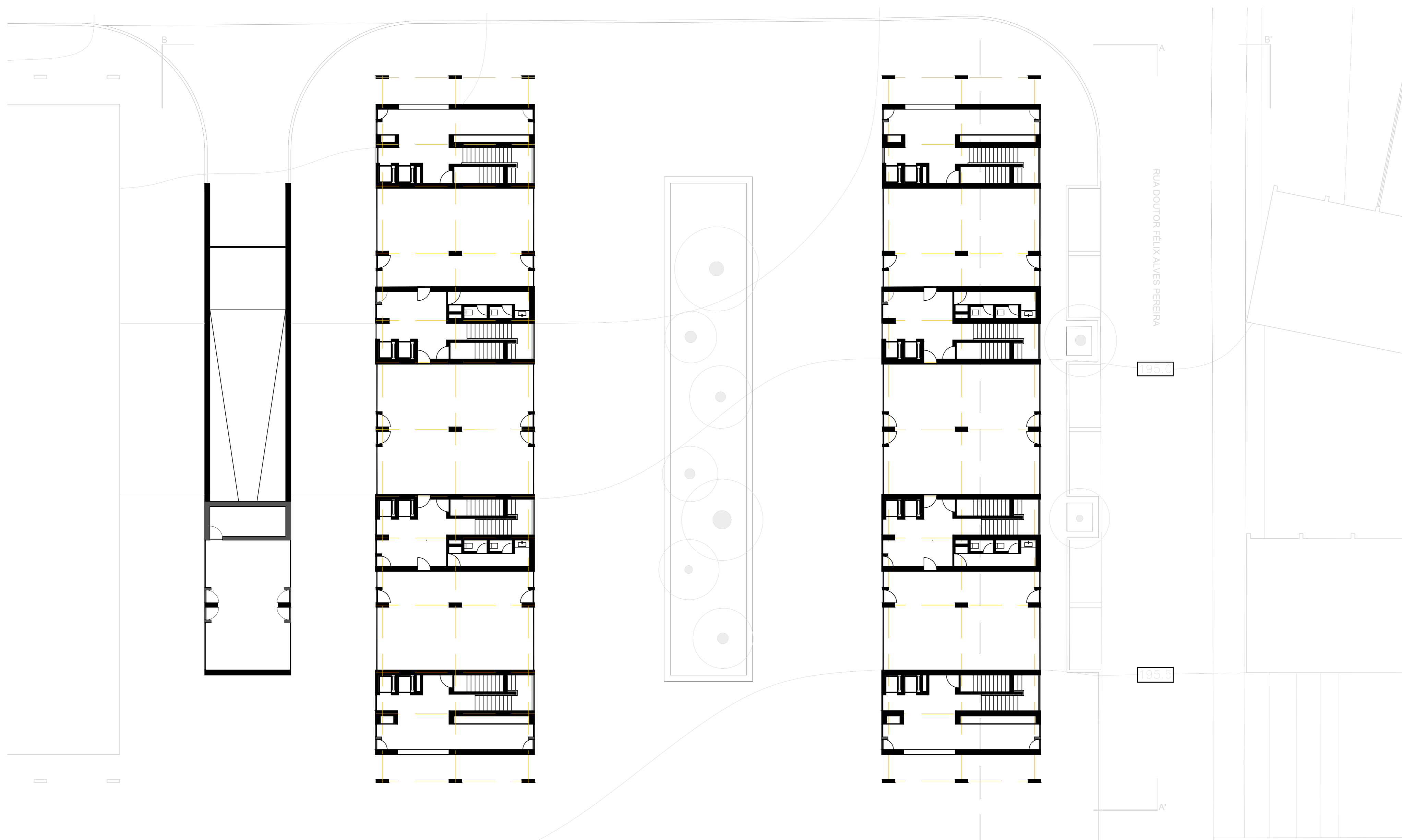
ESC. 1/200 | PLANTA PISO TÉRREO
