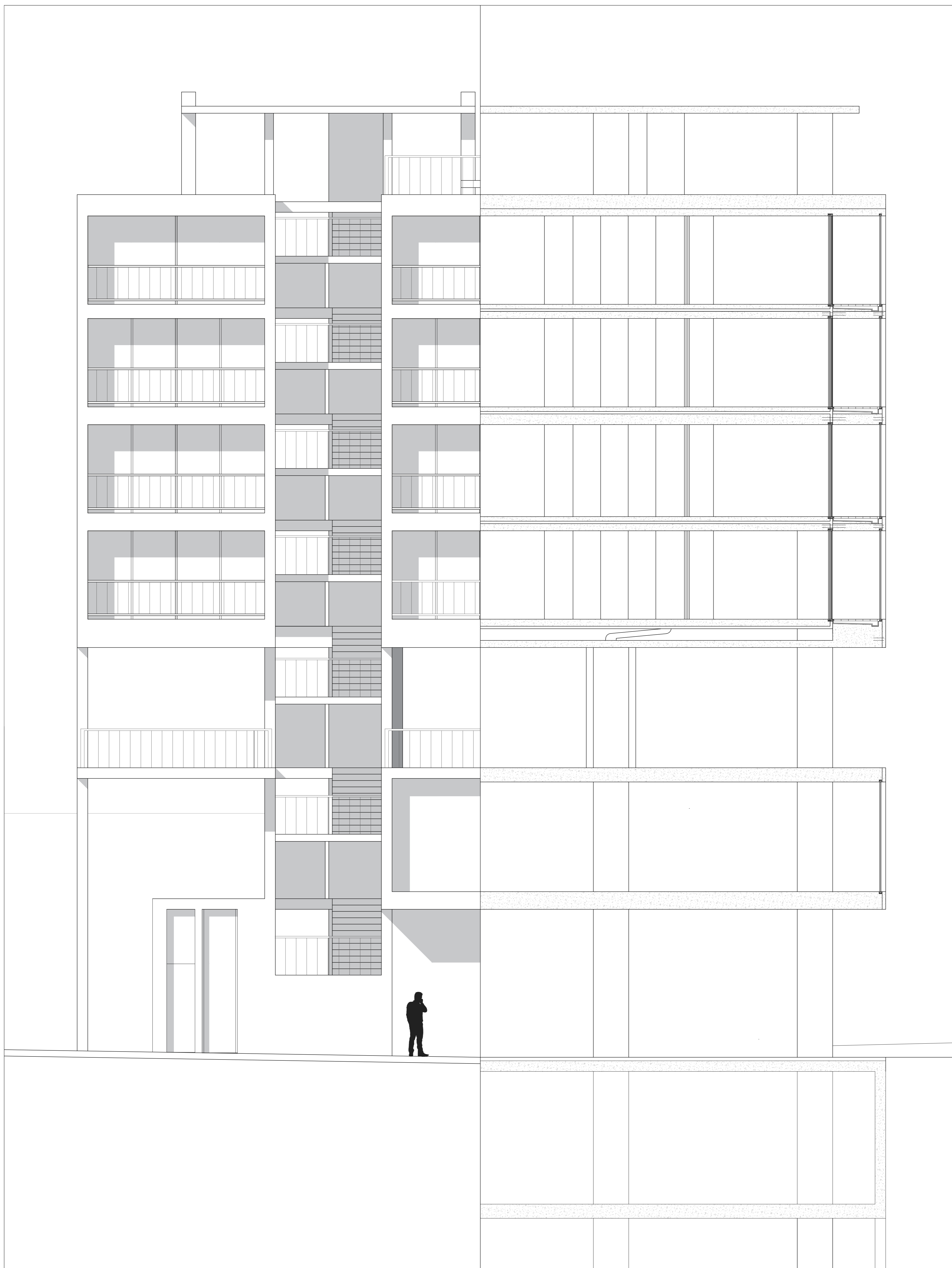
PERFIL LONGITUDINAL
