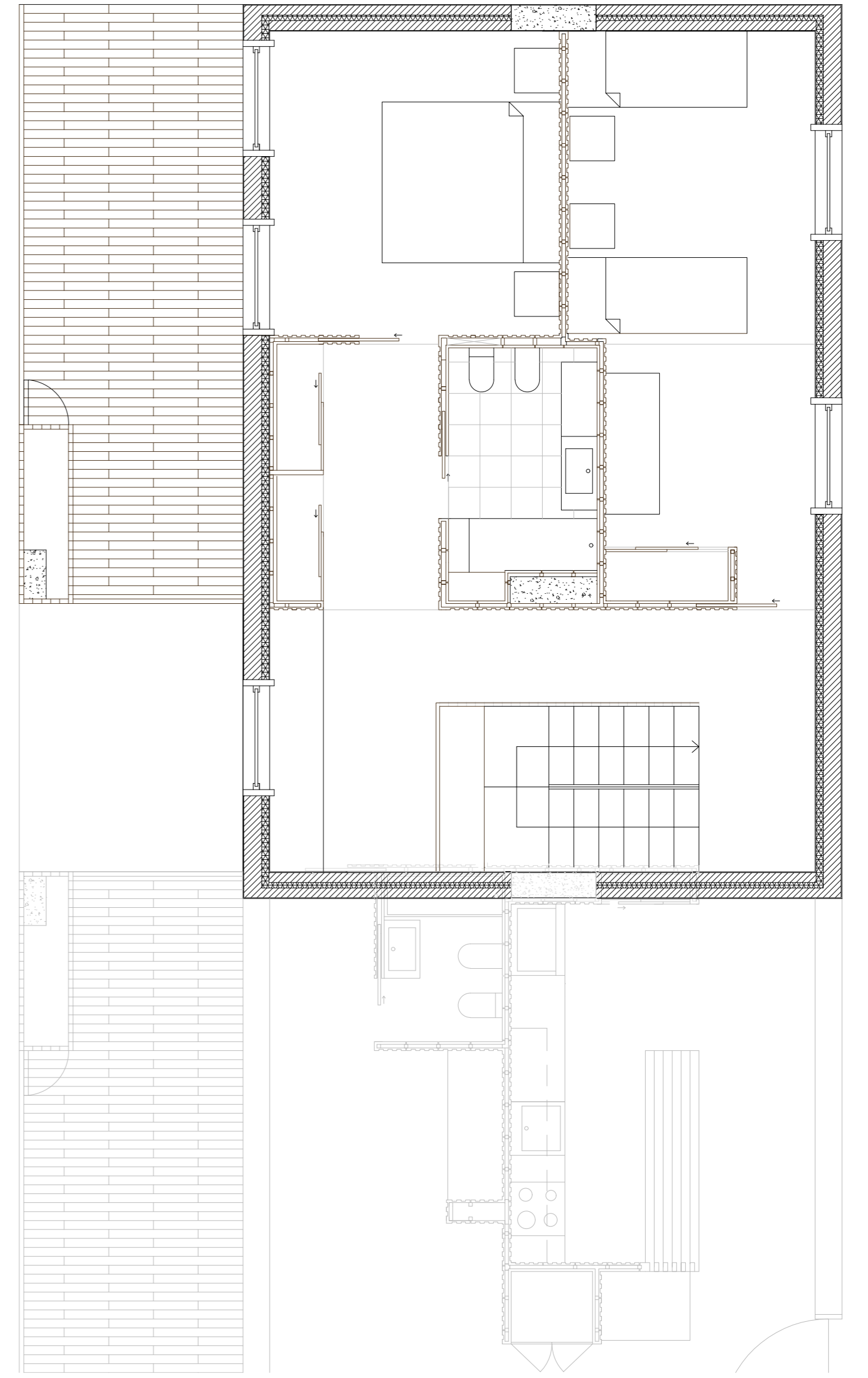
PLANTA | ESC. 1:50
