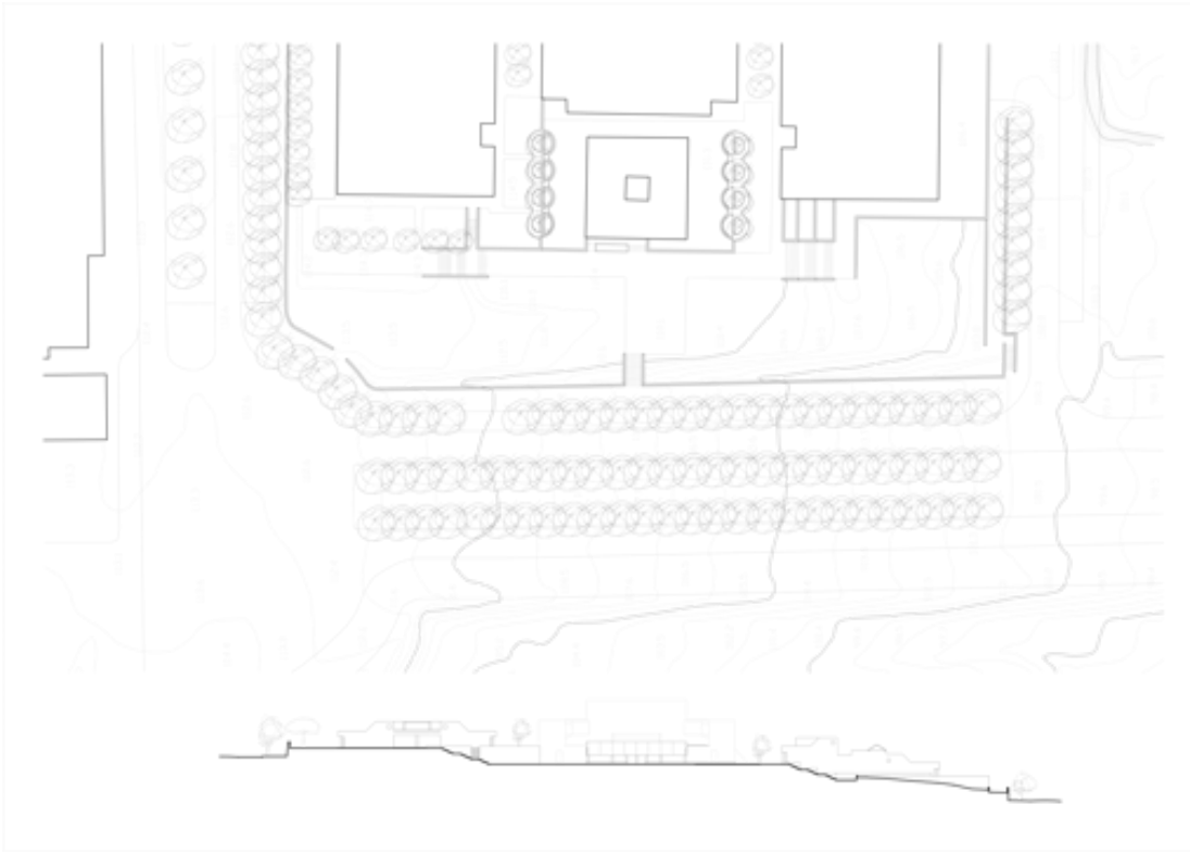
04 Planta de Implantação e Alçado Frontal esc. 1/500
