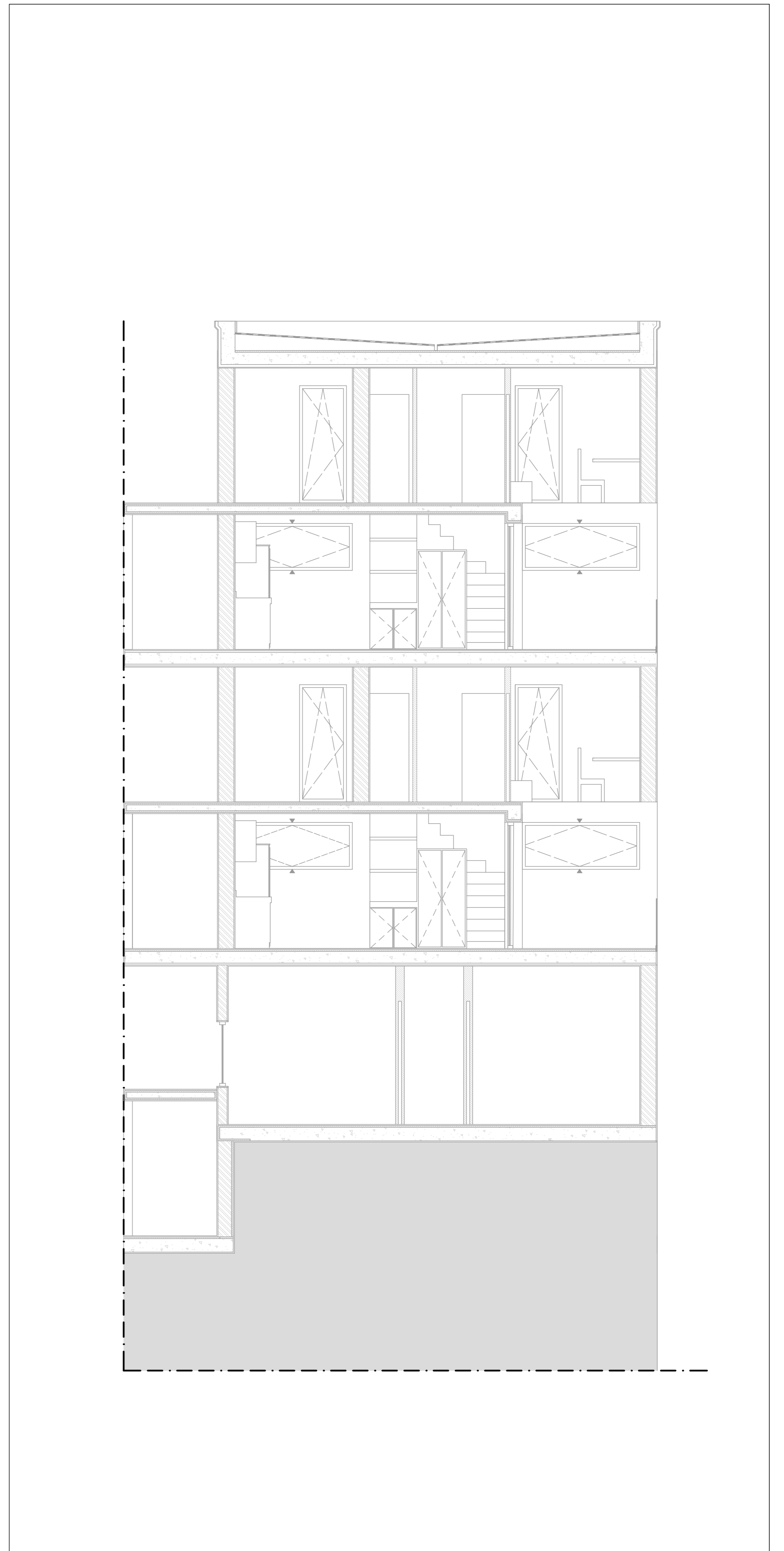
CORTE | ESC. 1:50
