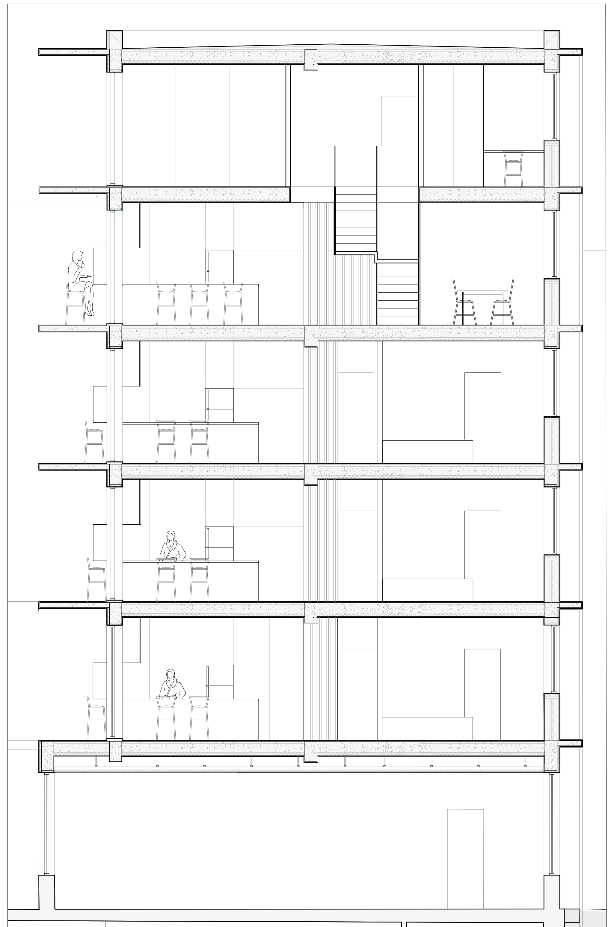
CORTE | ESC. 1:50
