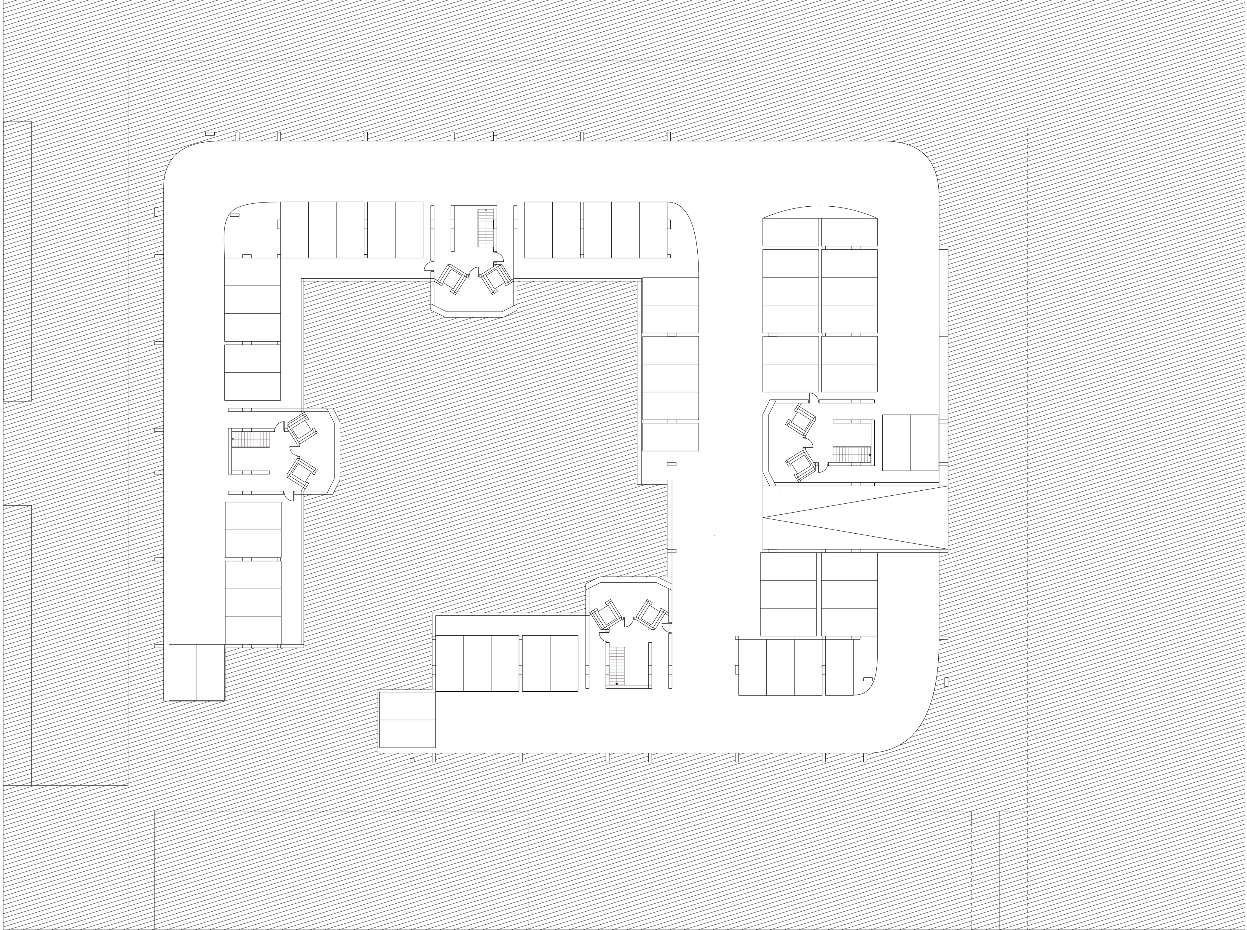
ESC. 1/200 | PLANTA DE ESTACIONAMENTO
