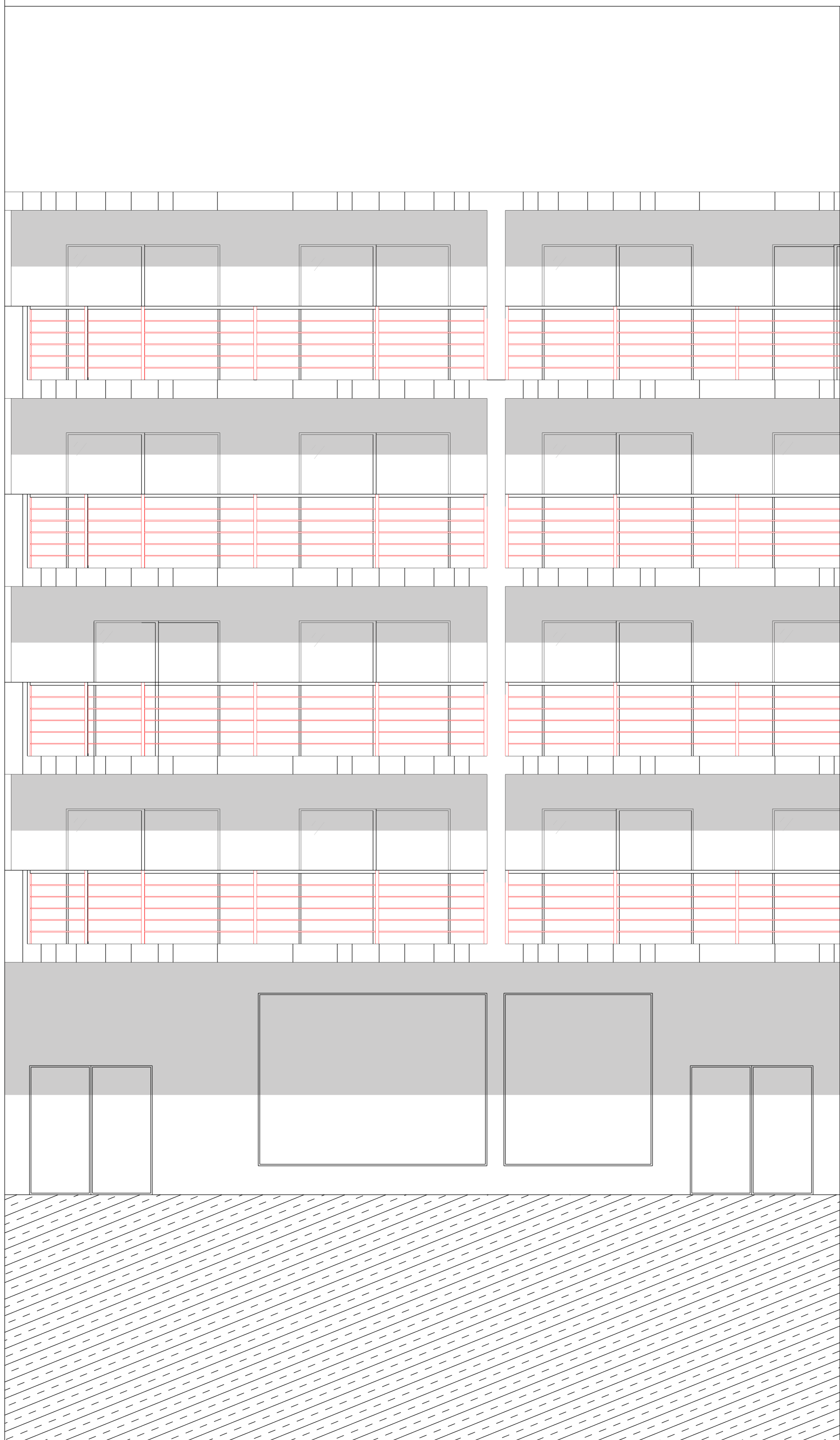
ALÇADO | ESC. 1:50
