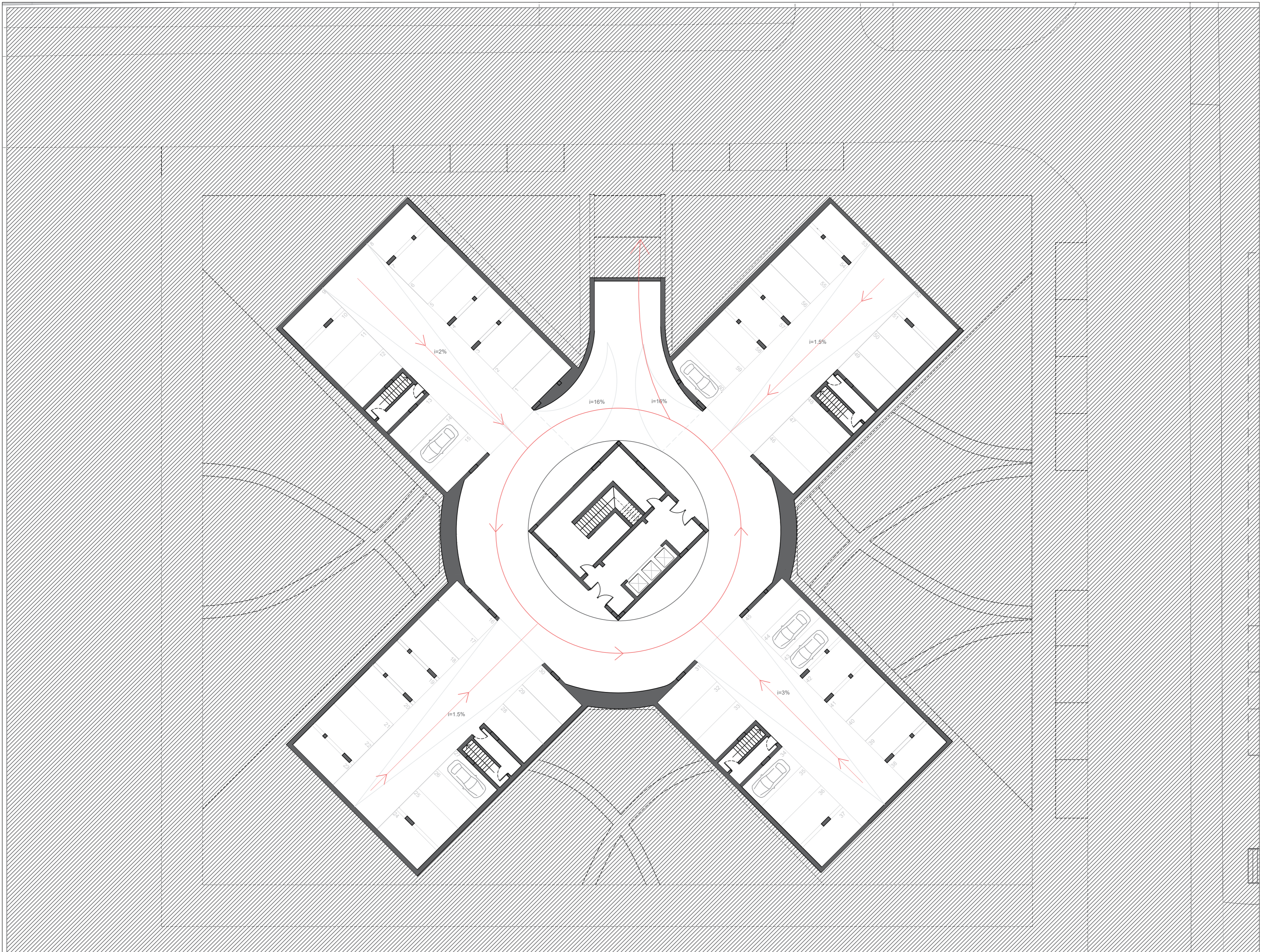
PLANTA DO ESTACIONAMENTO | COTA 193 | N ⌚
