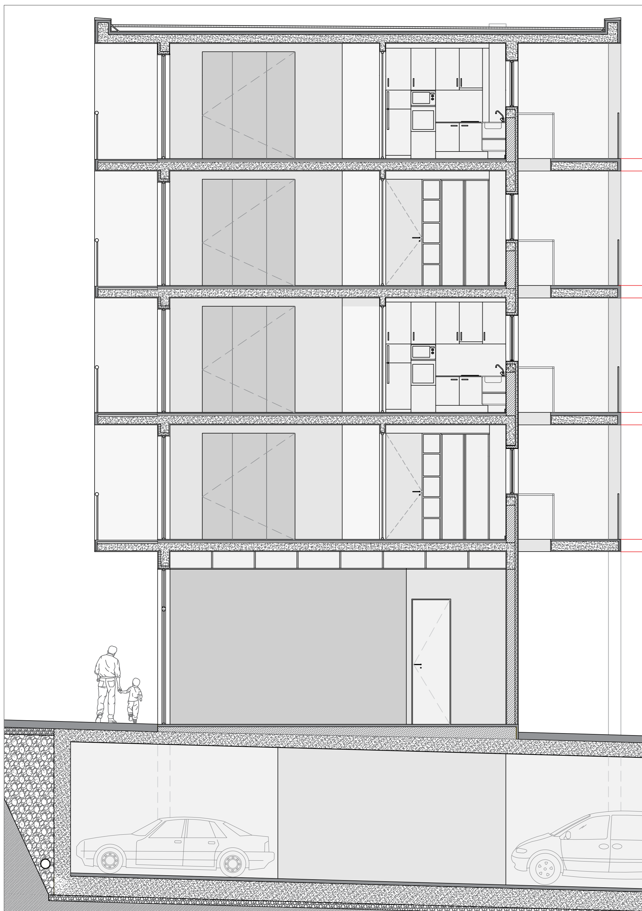
ALÇADO | ESC. 1:50
