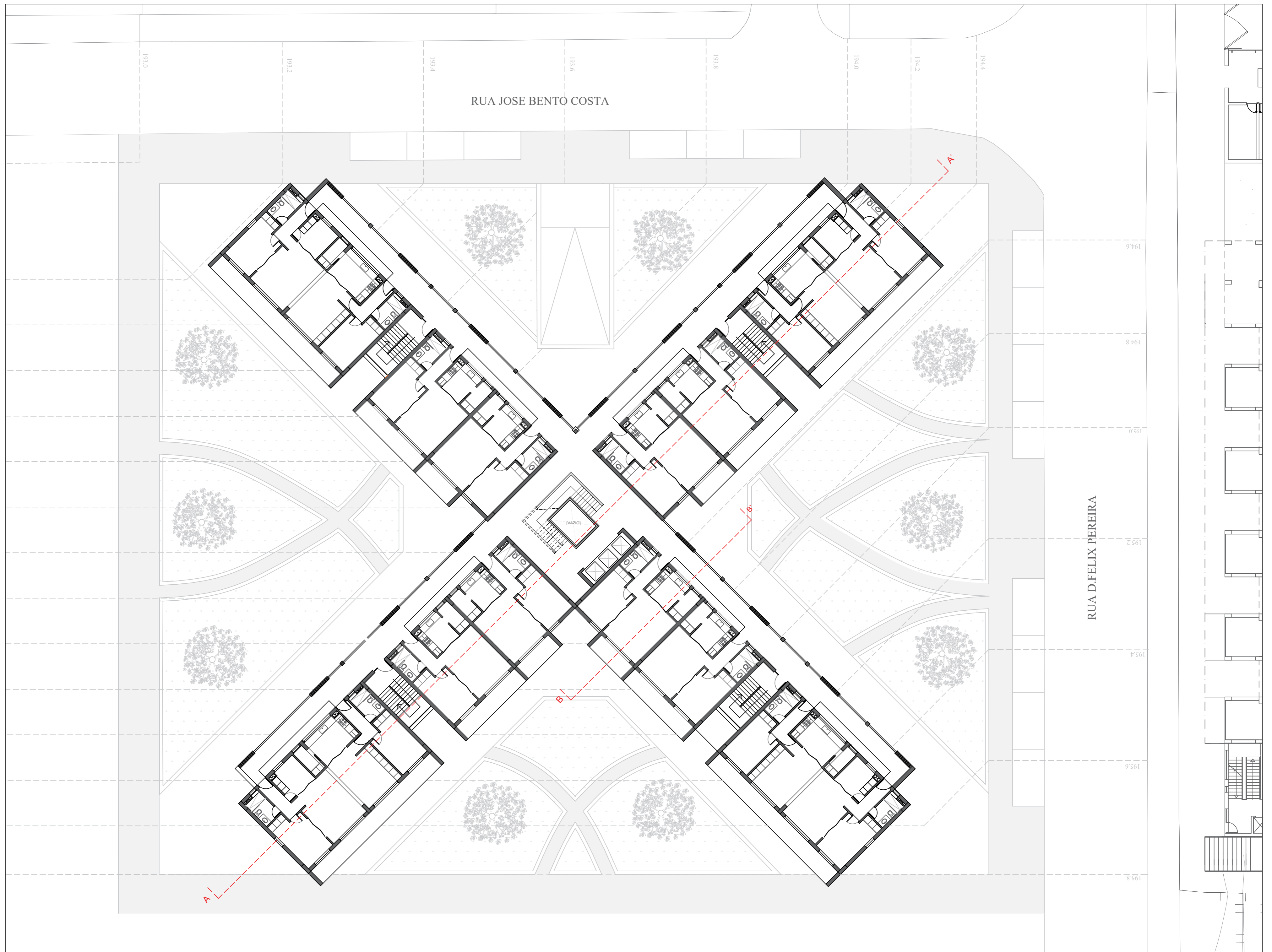
PLANTA PISO TIPO | N 1
