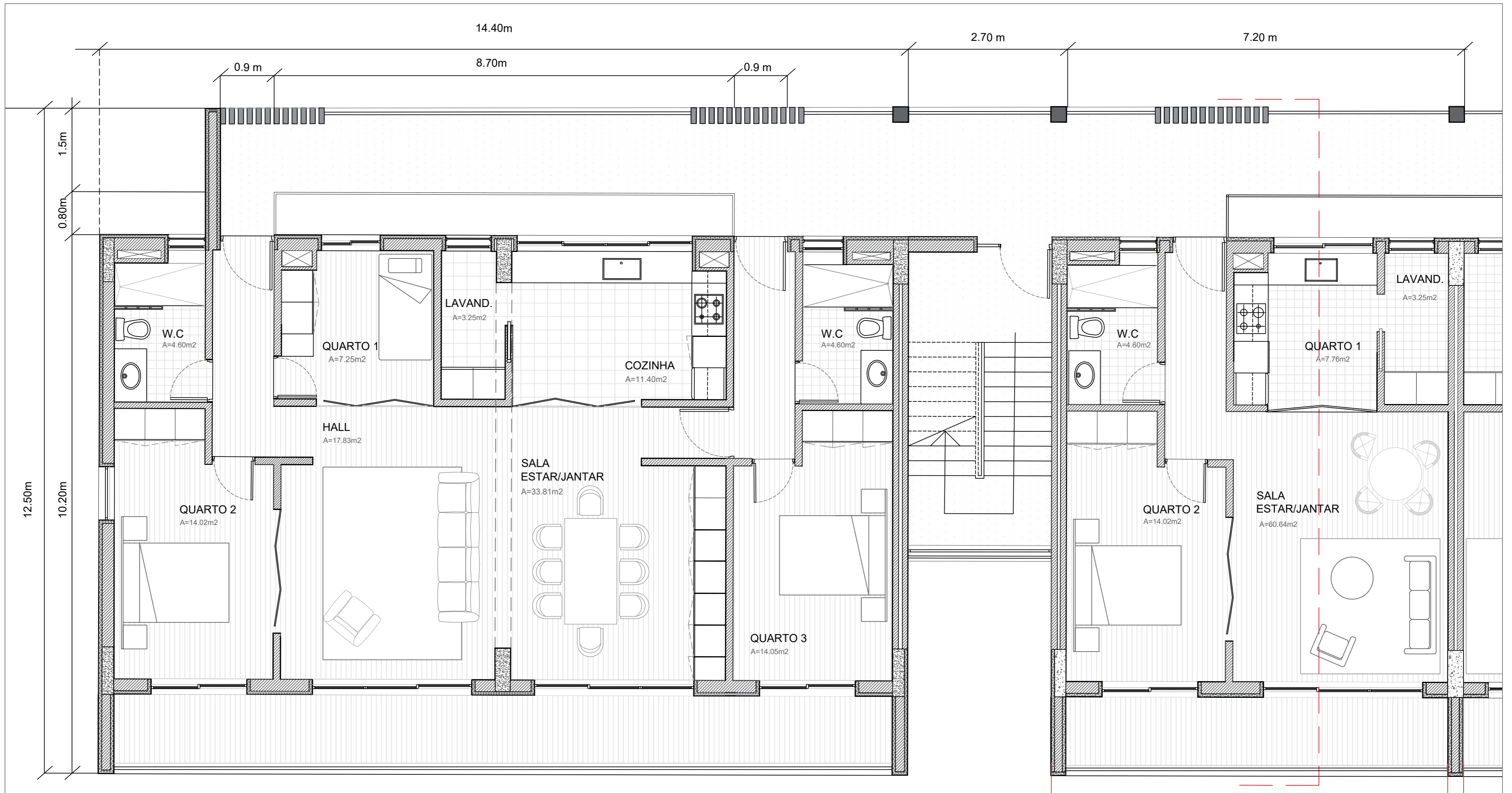
ESC. 1/50 | PLANTA PISO TIPO
