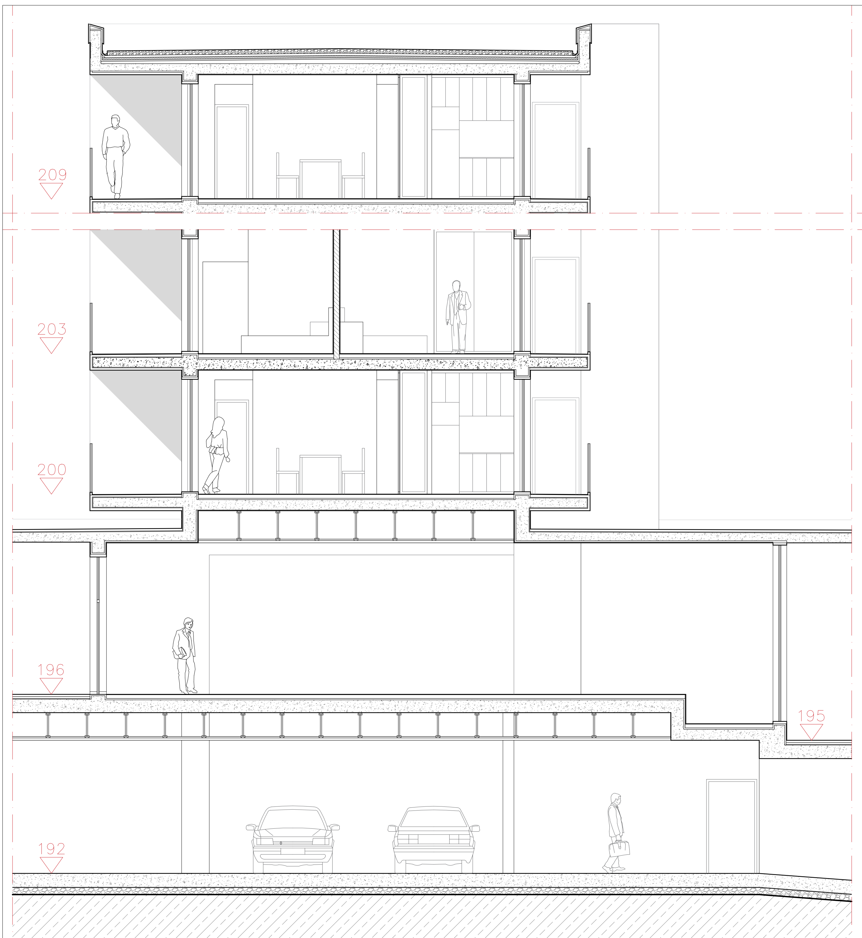
CORTE AA' | ESC. 1:50
