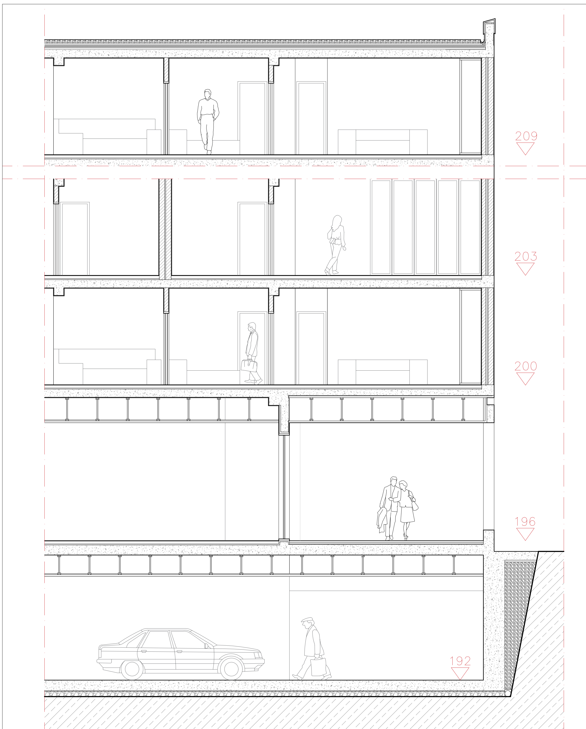
CORTE BB' | ESC. 1:50
