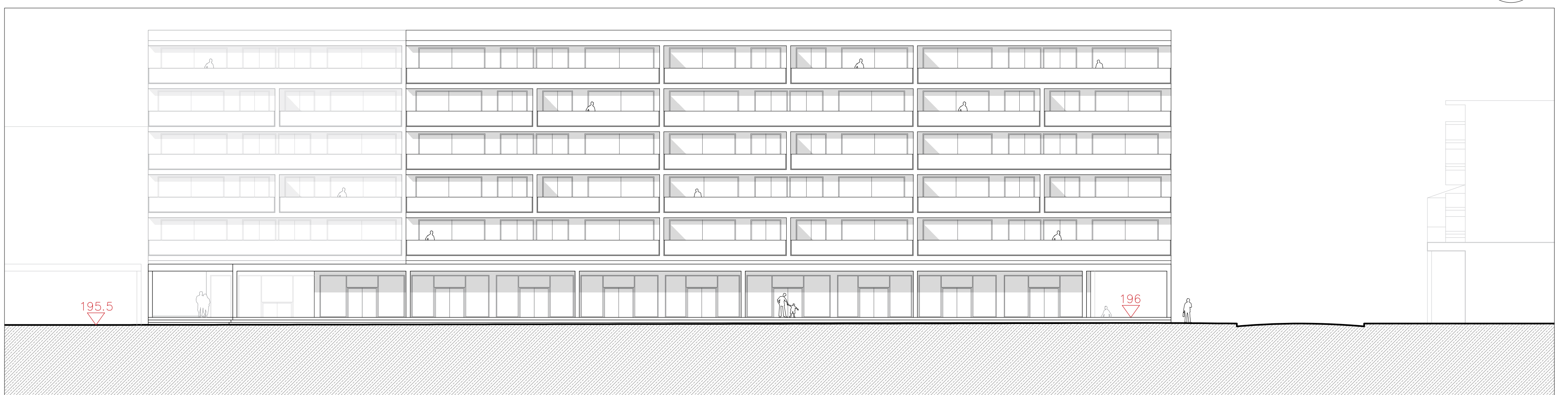
ALÇADO SUL
