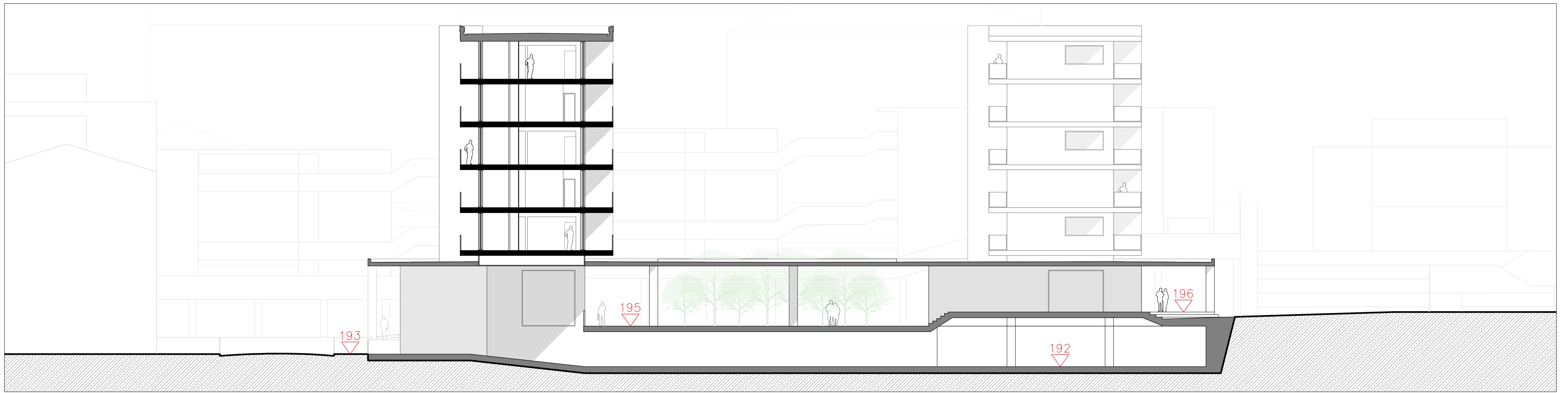
CORTE CC'
