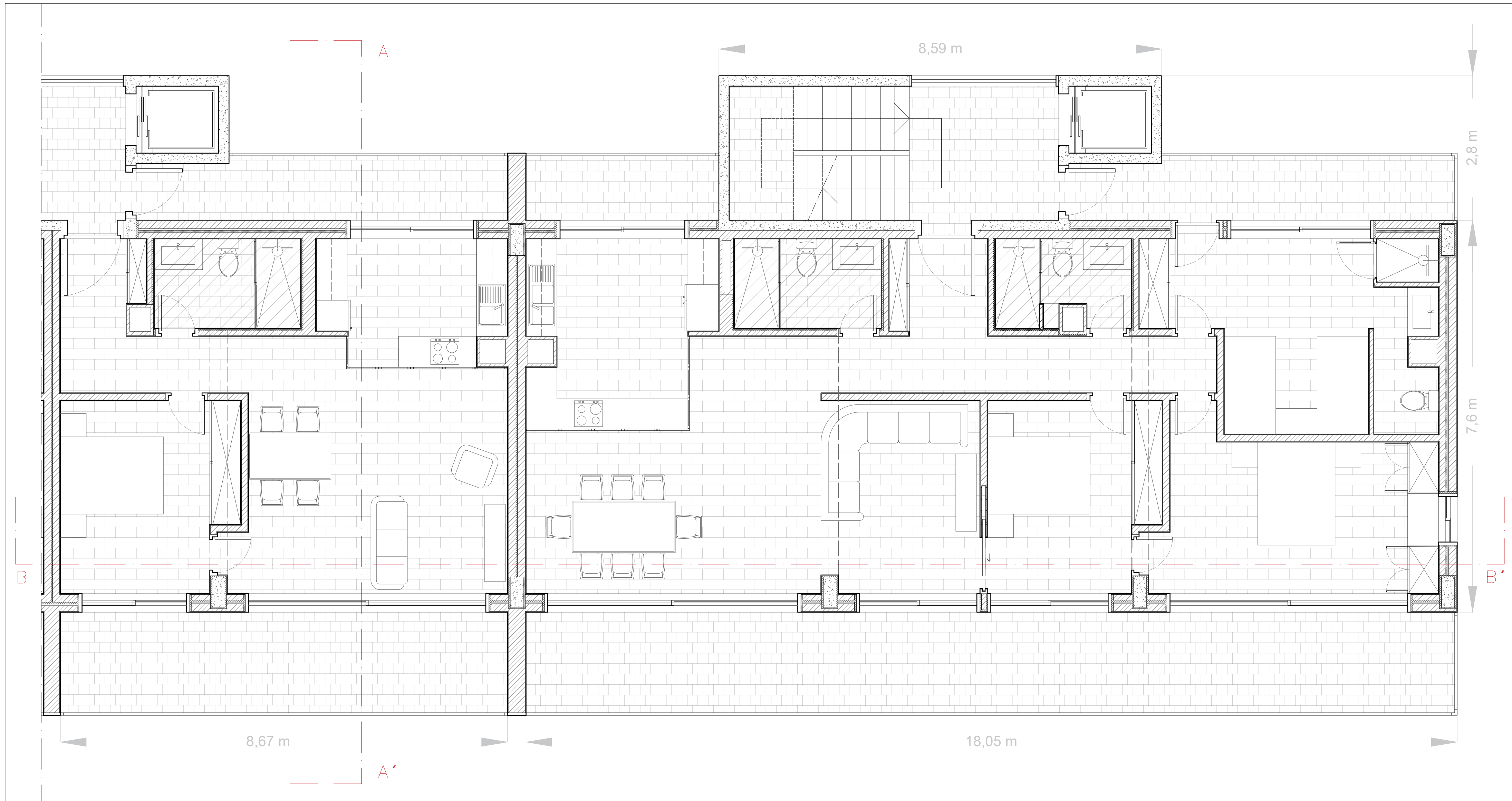
PLANTA | ESC. 1:50
