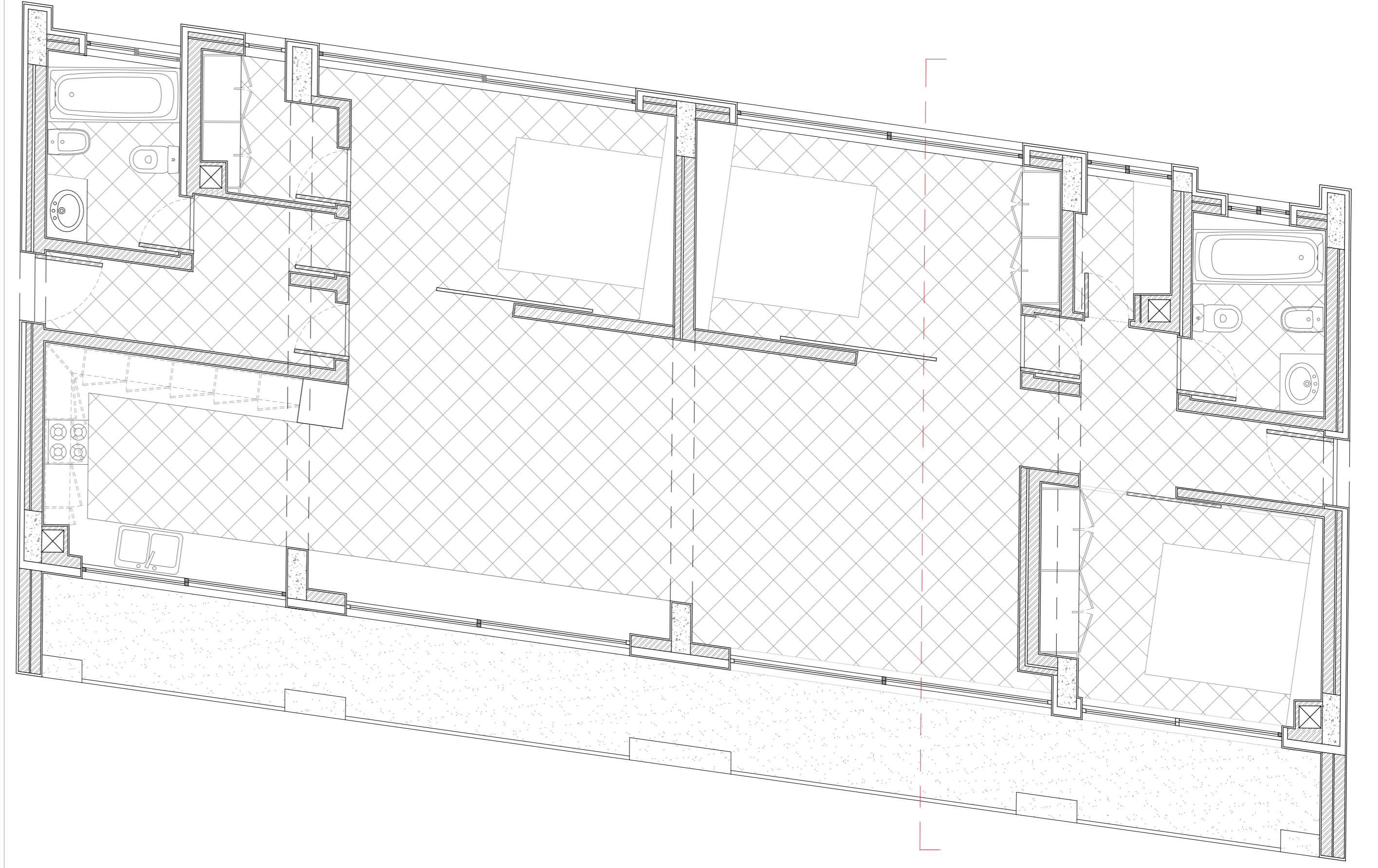
ESC. 1/50 | PLANTA DO FOGO GRANDE
