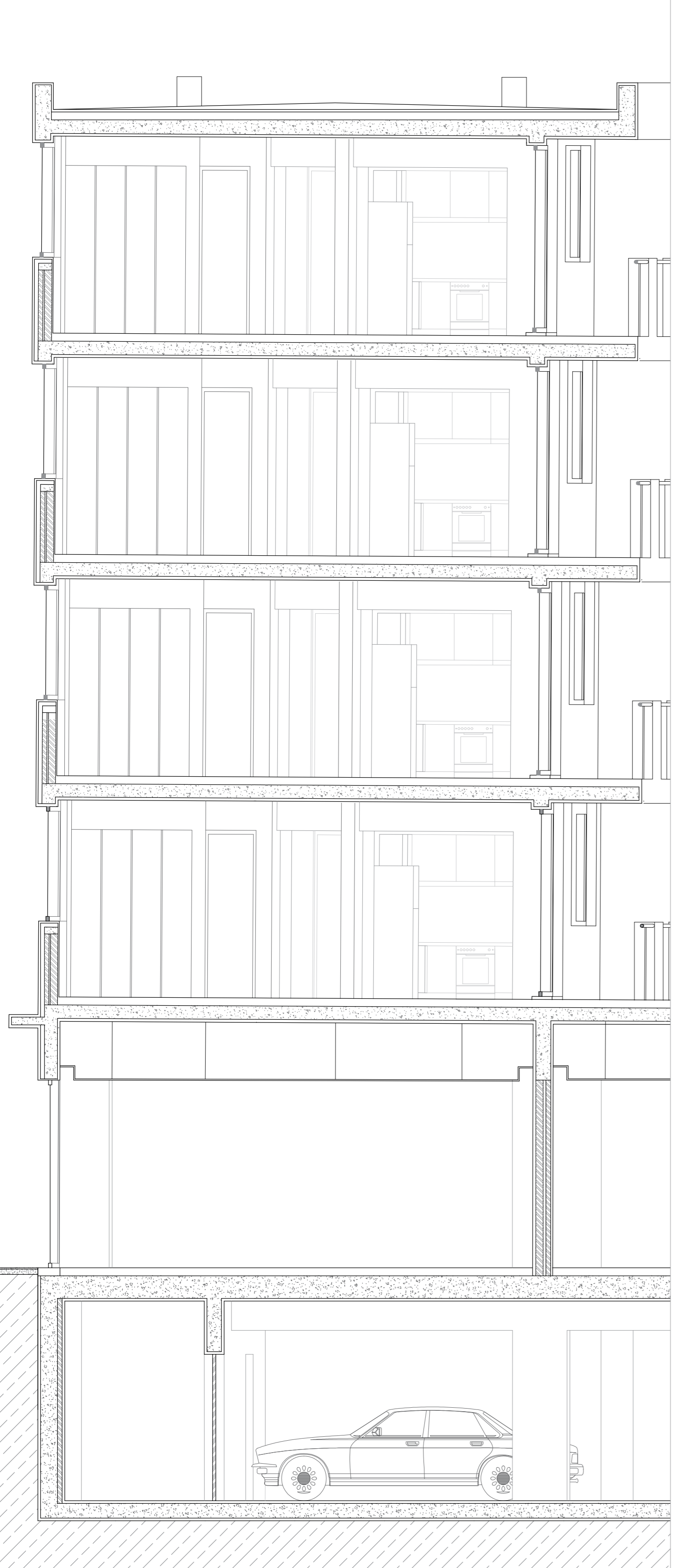
ESC. 1/50 | CORTE EE'
