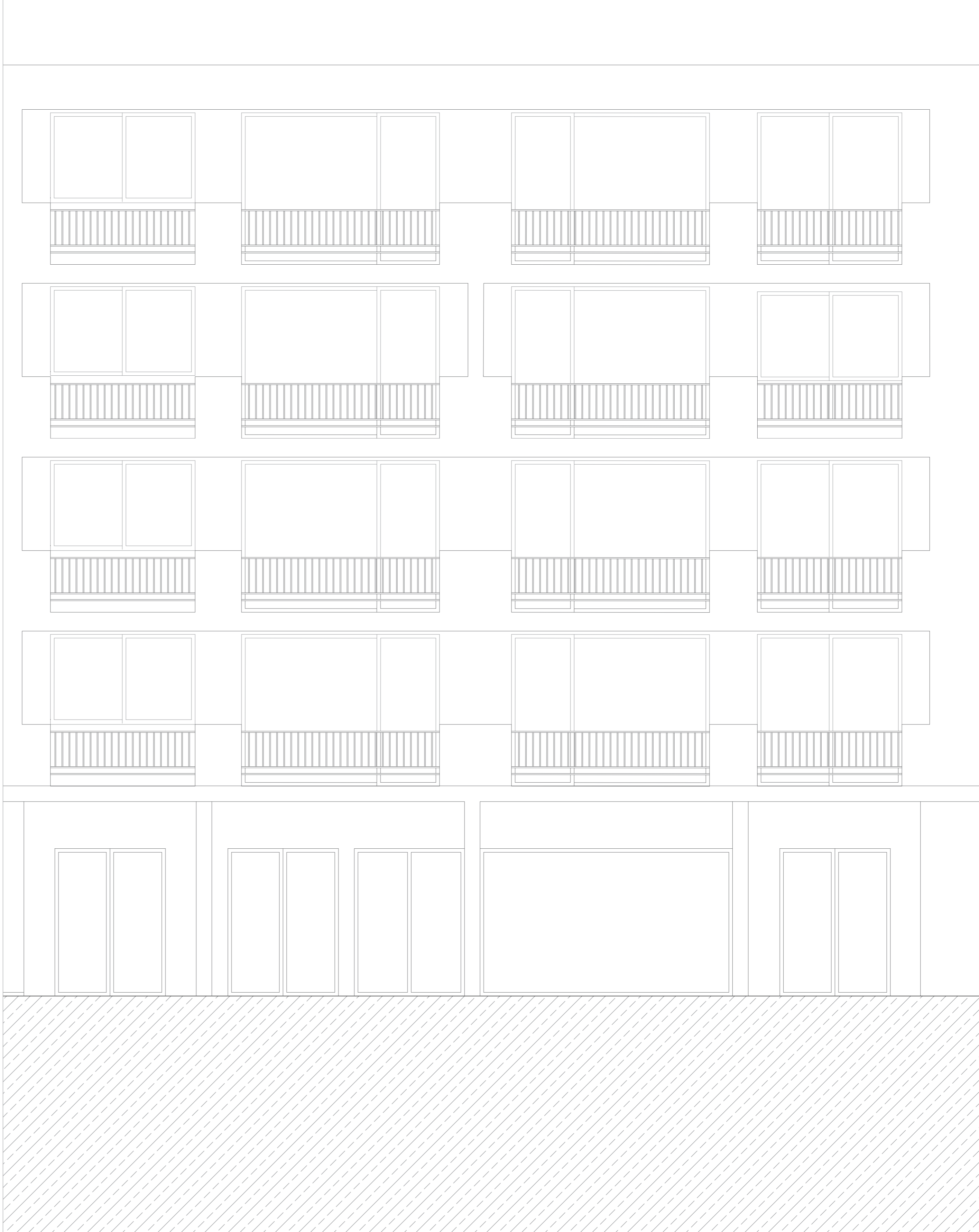
ESC. 1/50 | ALÇADO SUL
