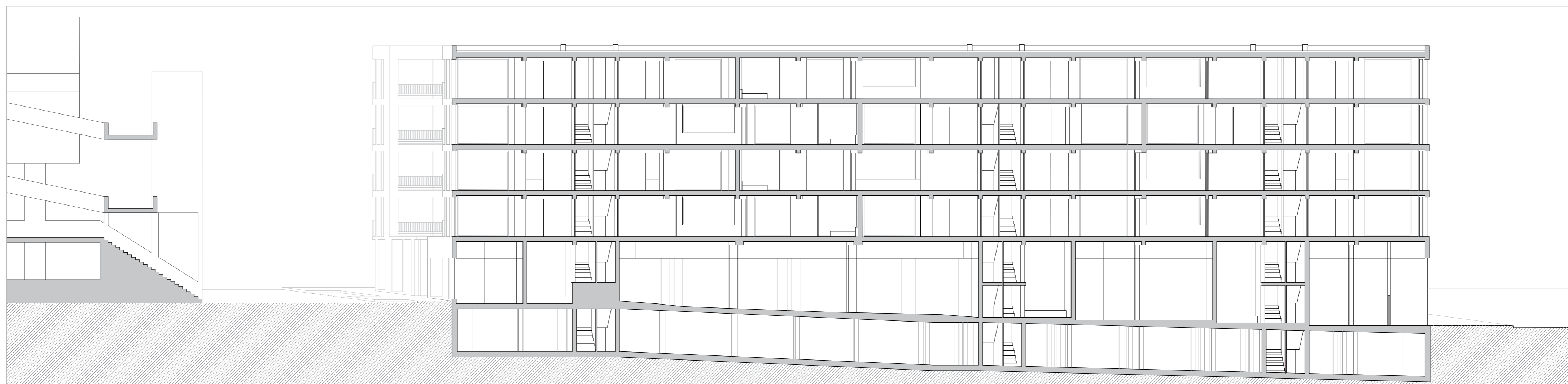
PERFIL LONGITUDINAL CC'
