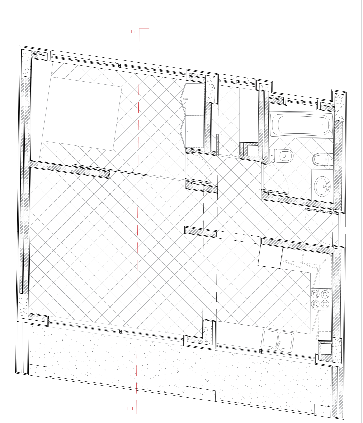
ESC. 1/50 | PLANTA DO FOGO PEQUENO
