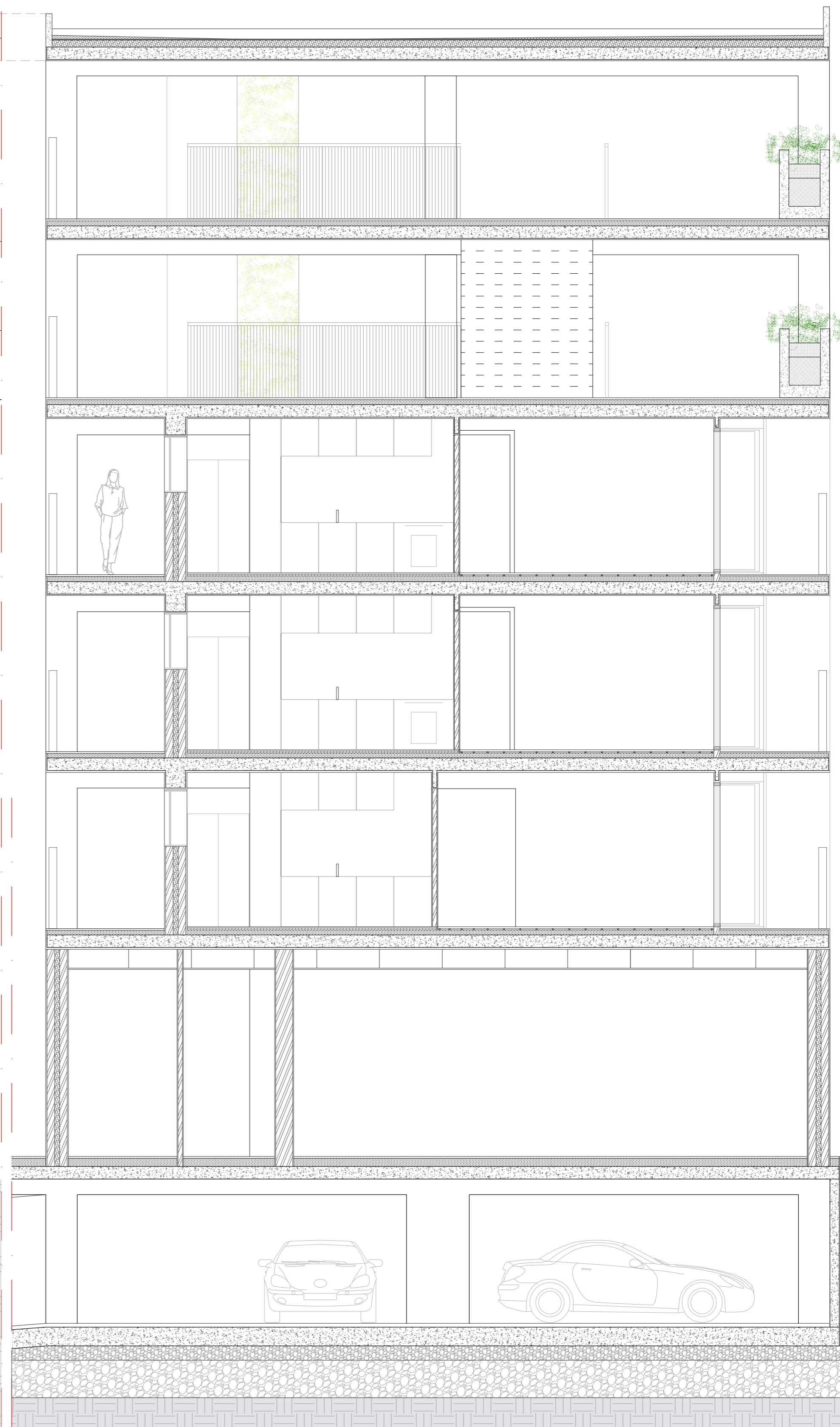
CORTE A A' | ESC. 1:50
