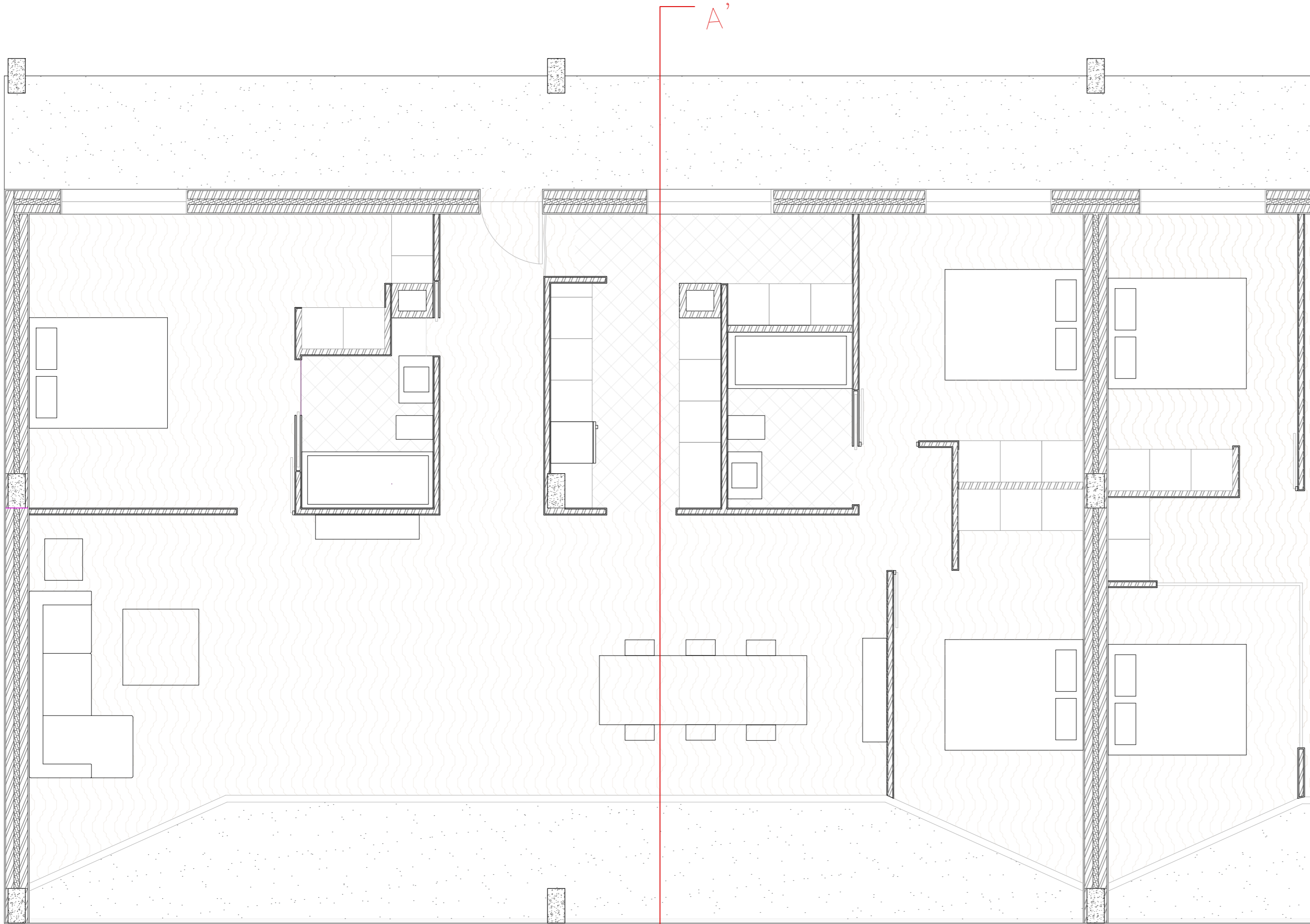
PLANTA FOGO GRANDE | ESC. 1:50
