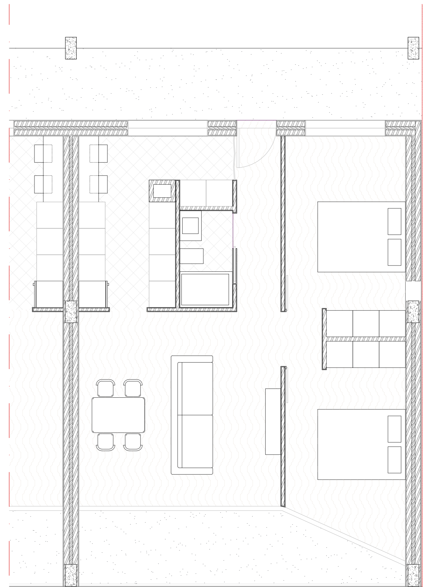
PLANTA FOGO PEQUENO | ESC. 1:50
