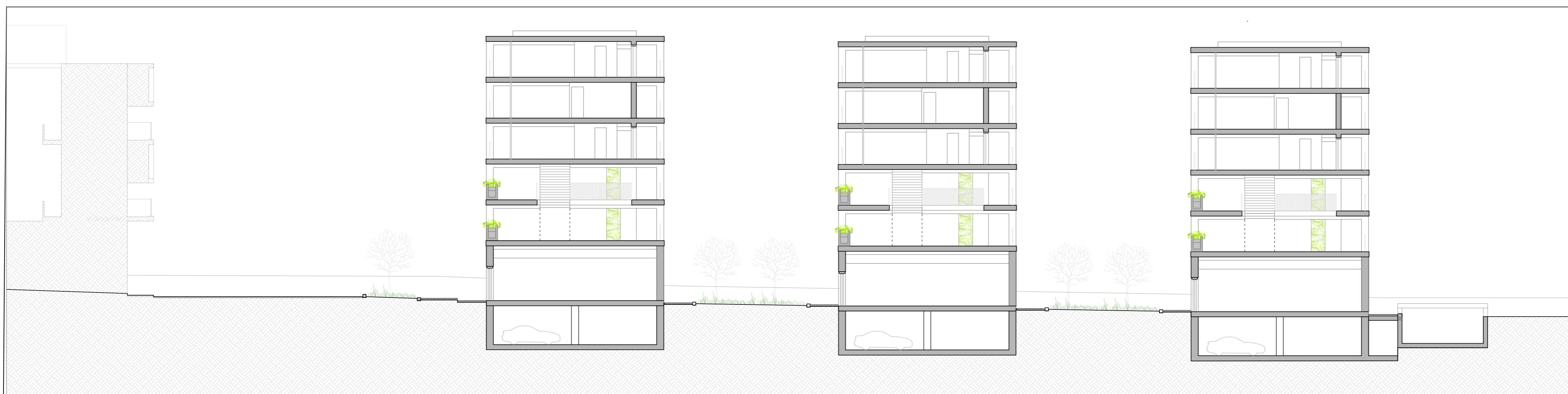
PERFIL TRANSVERSAL
