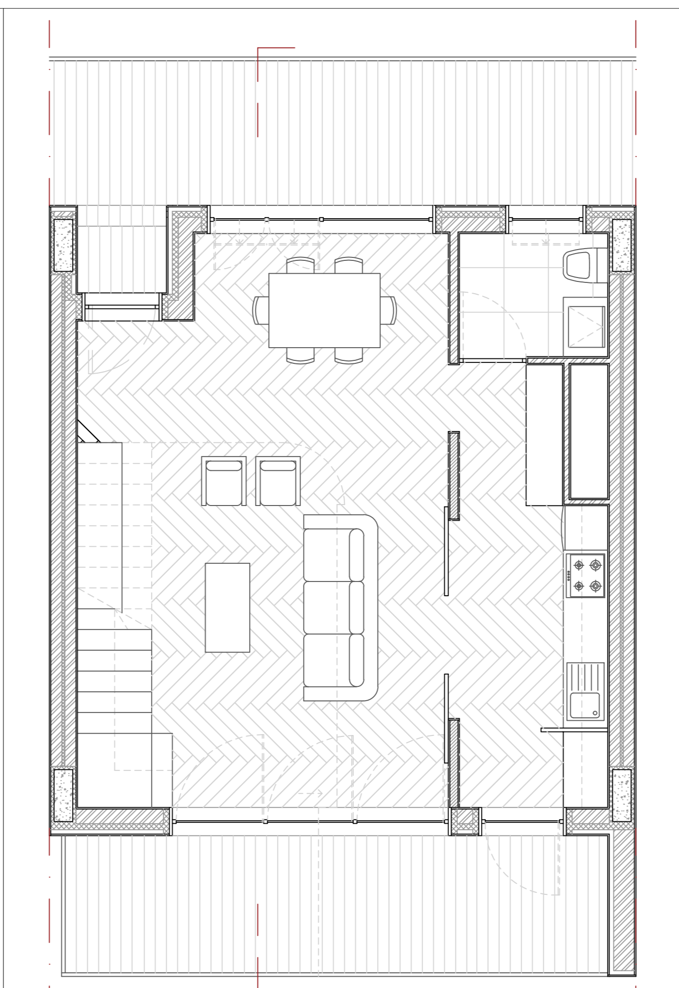
Planta Fogo Grande | Piso 0
