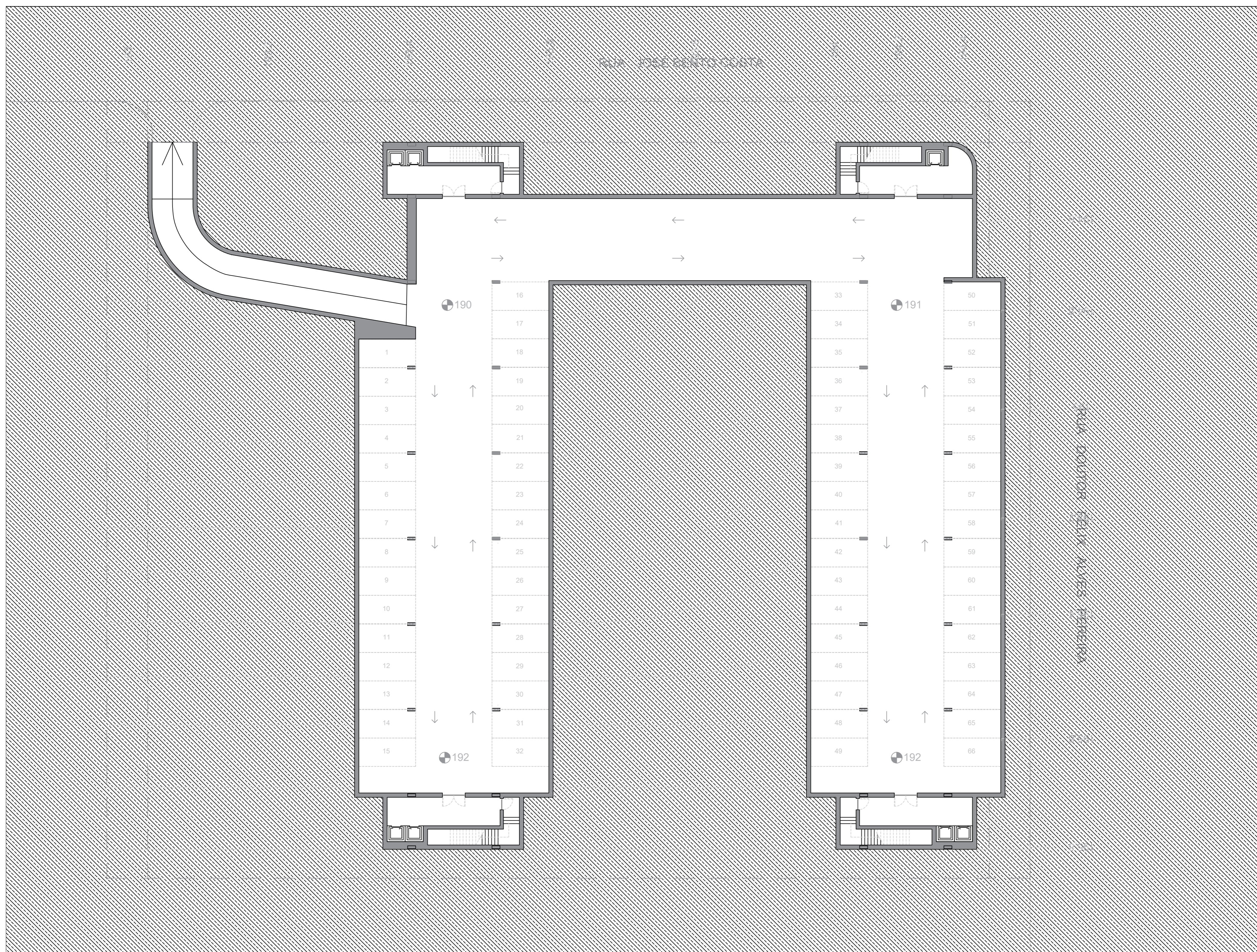
Planta Estacionamento N
