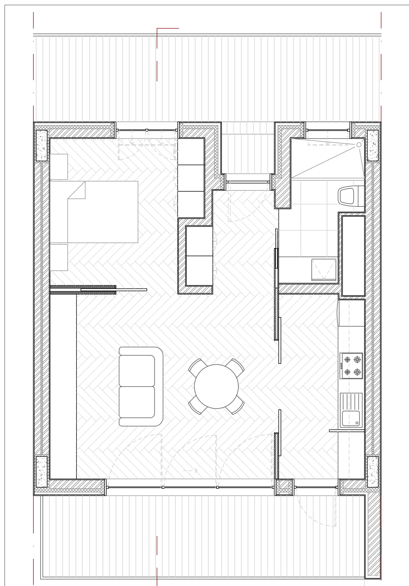
Planta Fogo Pequeno
