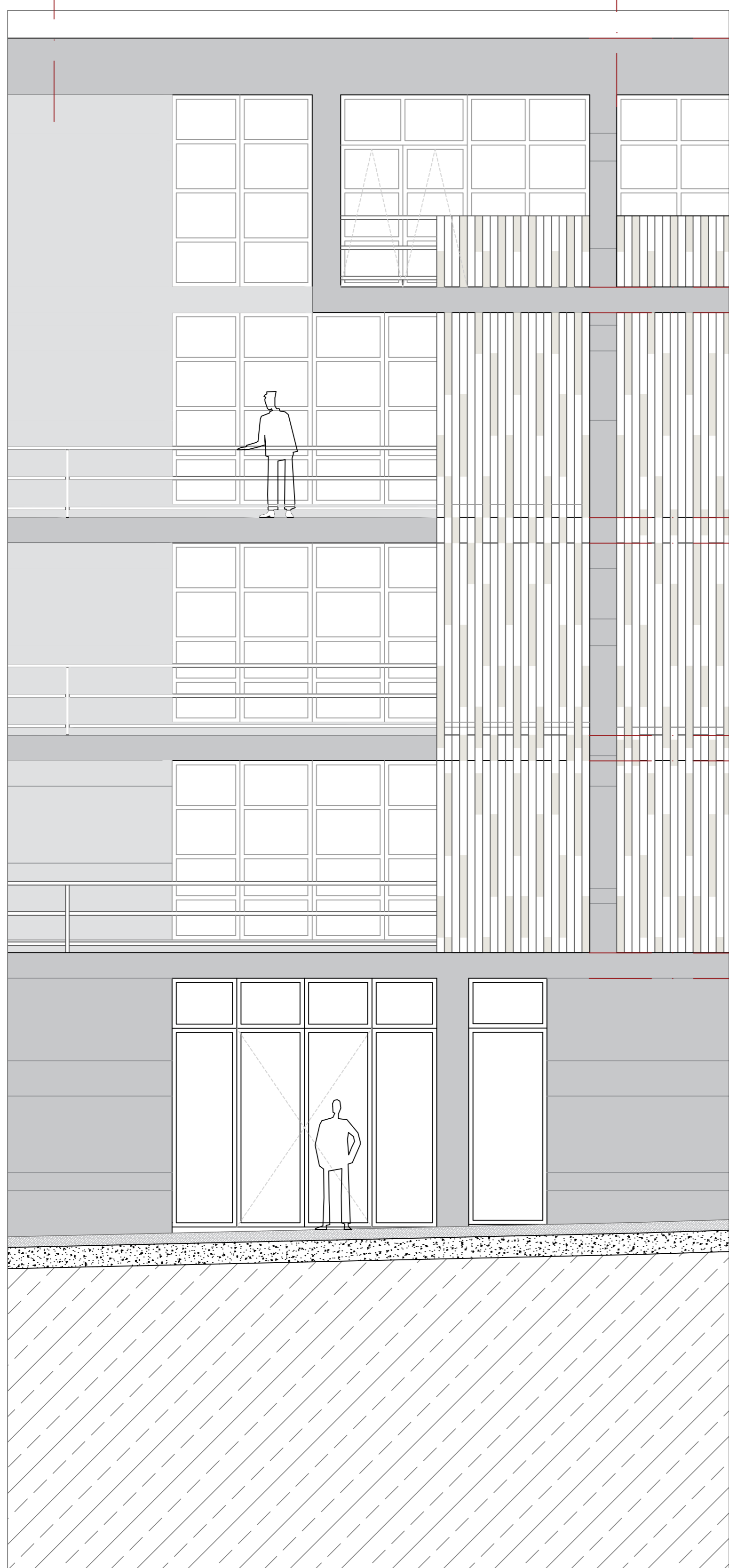
Alçado
