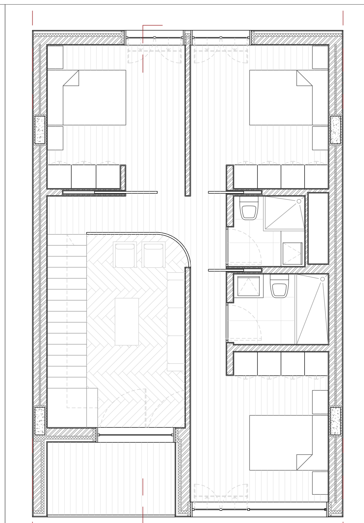
Planta Fogo Grande | Piso 1
