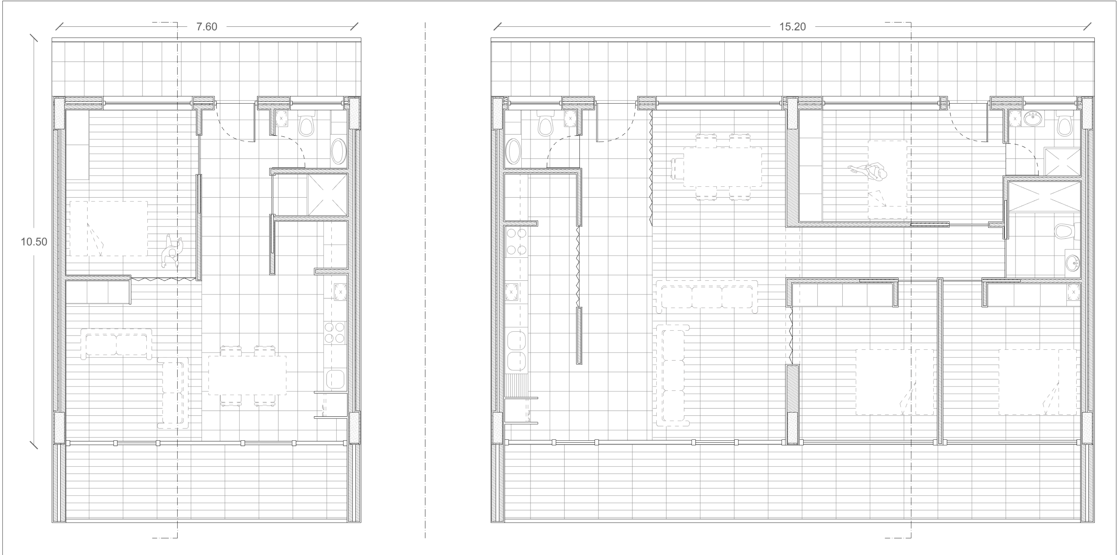
ESC. 1/50 PLANTA
