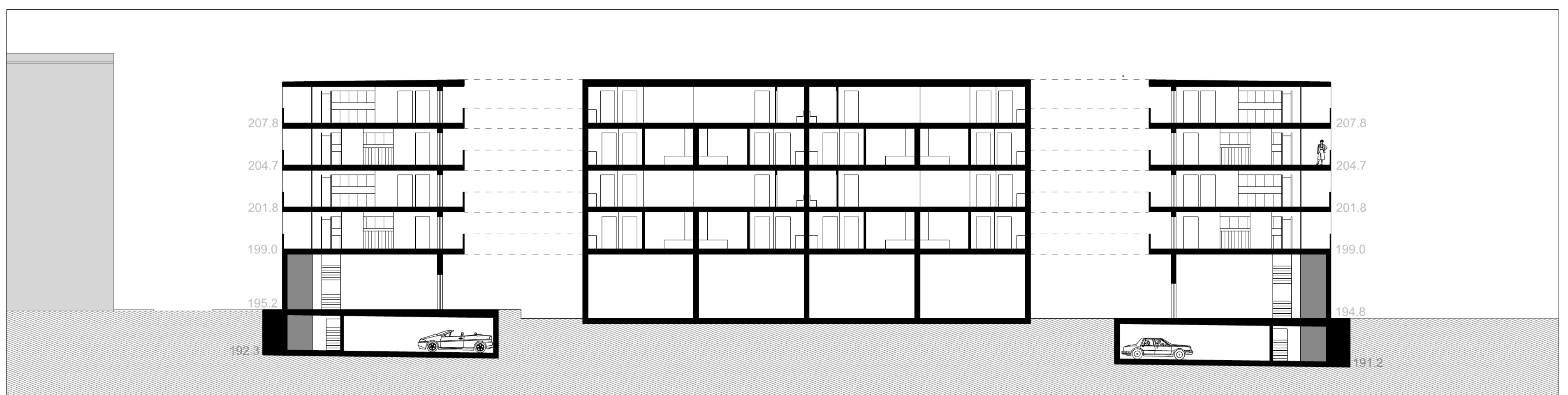
ESC. 1/200 PERFIL LONGITUDINAL AA'
