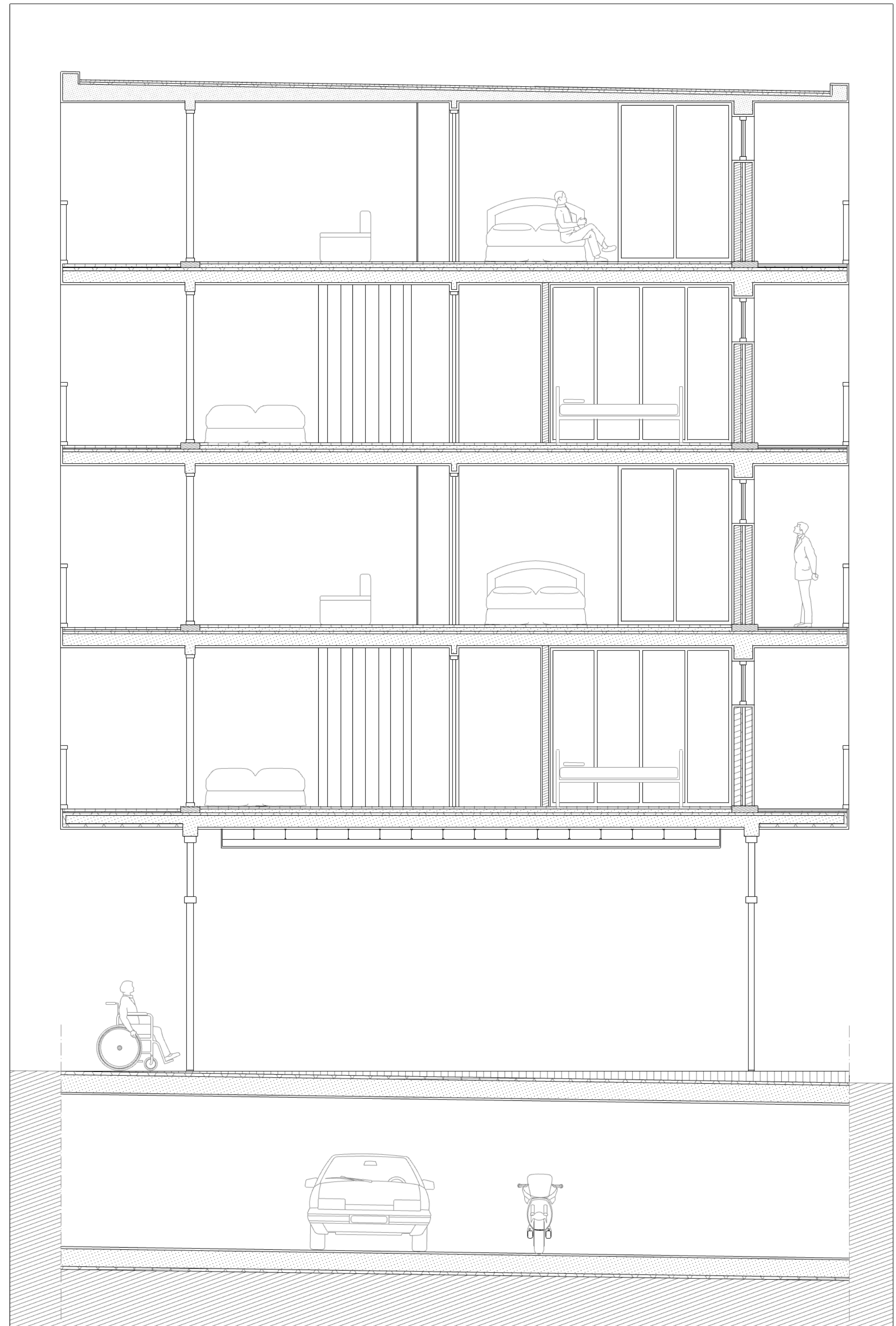
ESC. 1/50 CORTE
