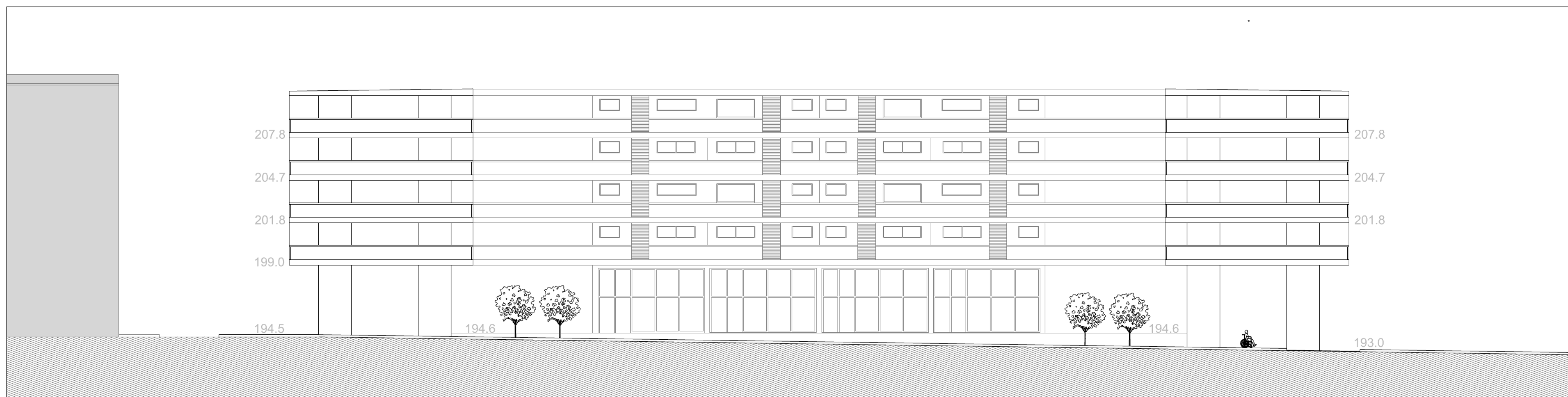
ESC. 1/200 ALÇADO RUA JOSÉ BENTO COSTA
