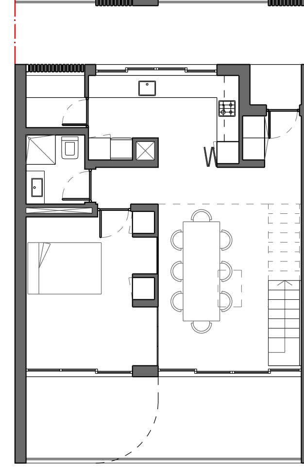
PLANTA T3 [sala piso 1]
