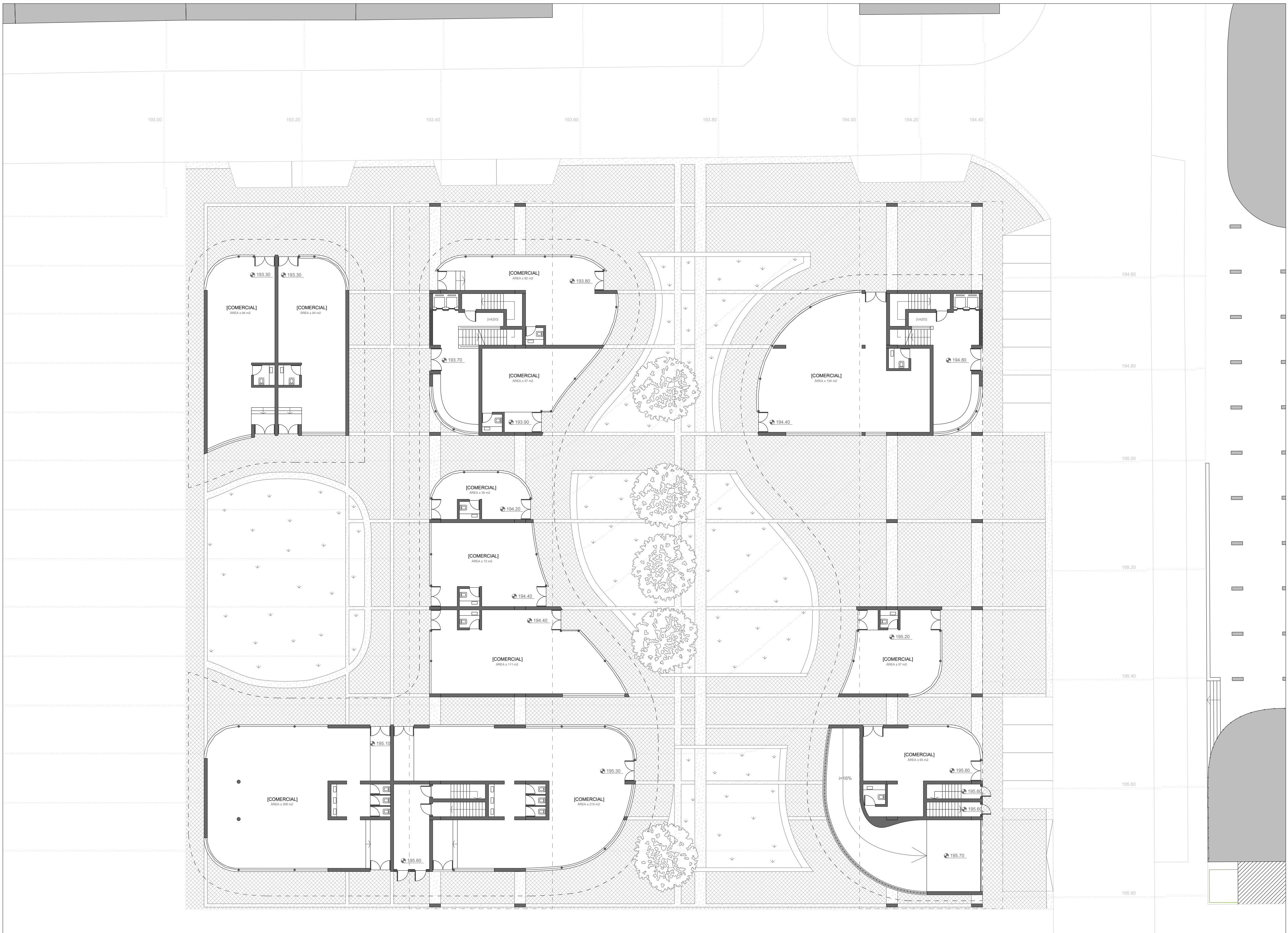
PLANTA PISO TÉRREO | COTA 197 | N
