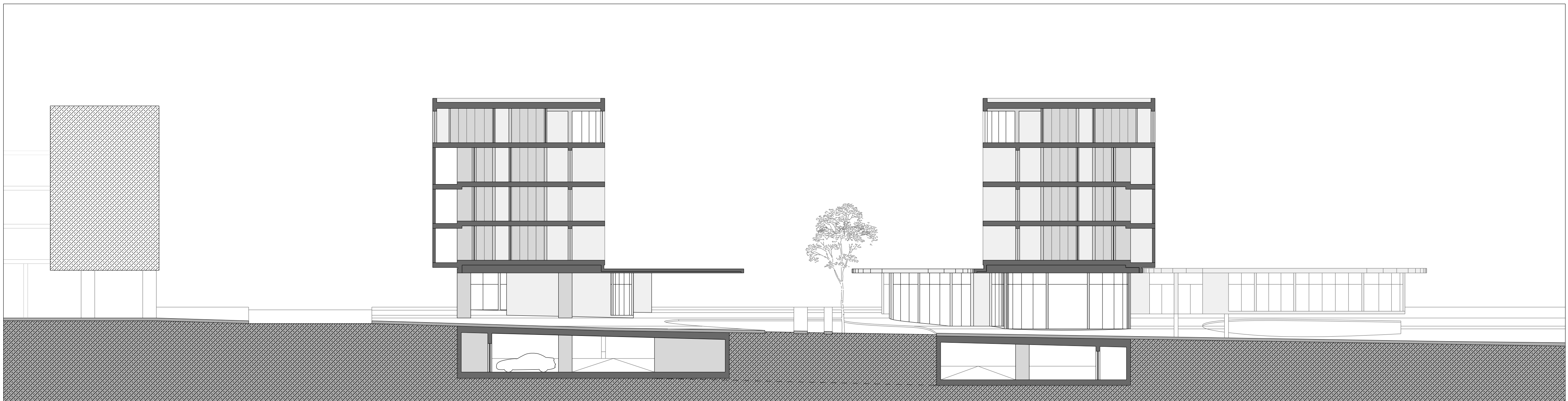
CORTE AA'
