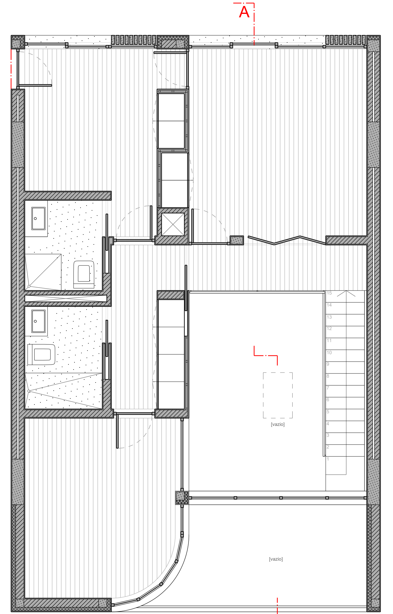
PLANTA FOGO GRANDE | PISO 1 [área ±69m 2 ]
