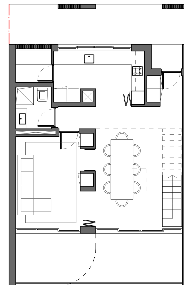
PLANTA T1 E T1 [entrada independente]
