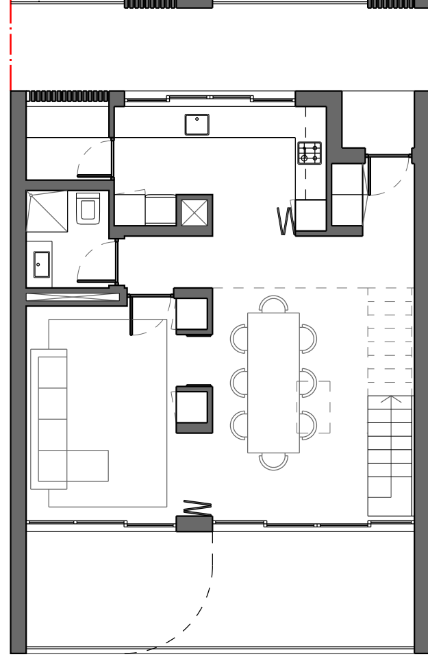
PLANTA T3 [quartos piso 1]
