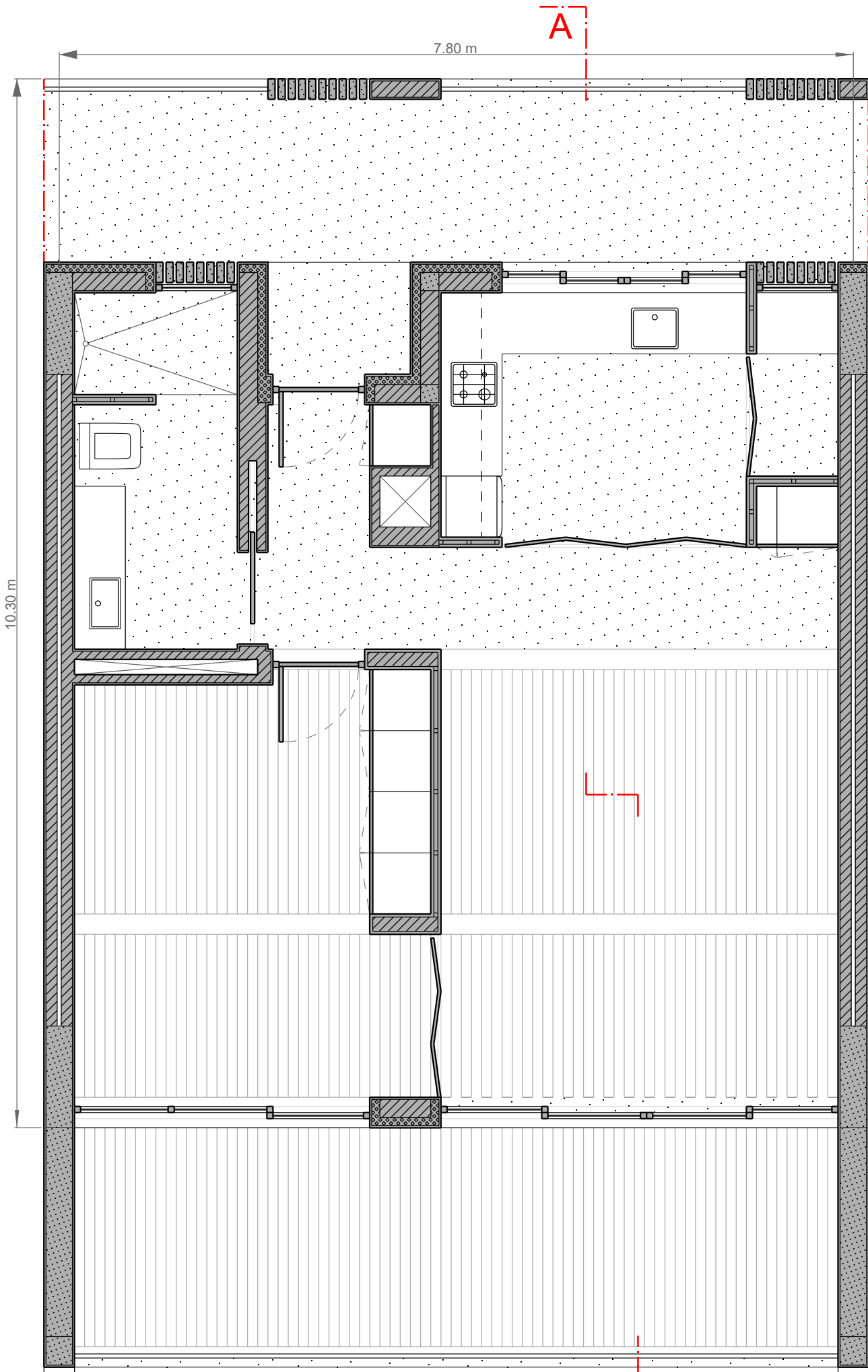
PLANTA FOGO PEQUENO [área 80m 2 ]
