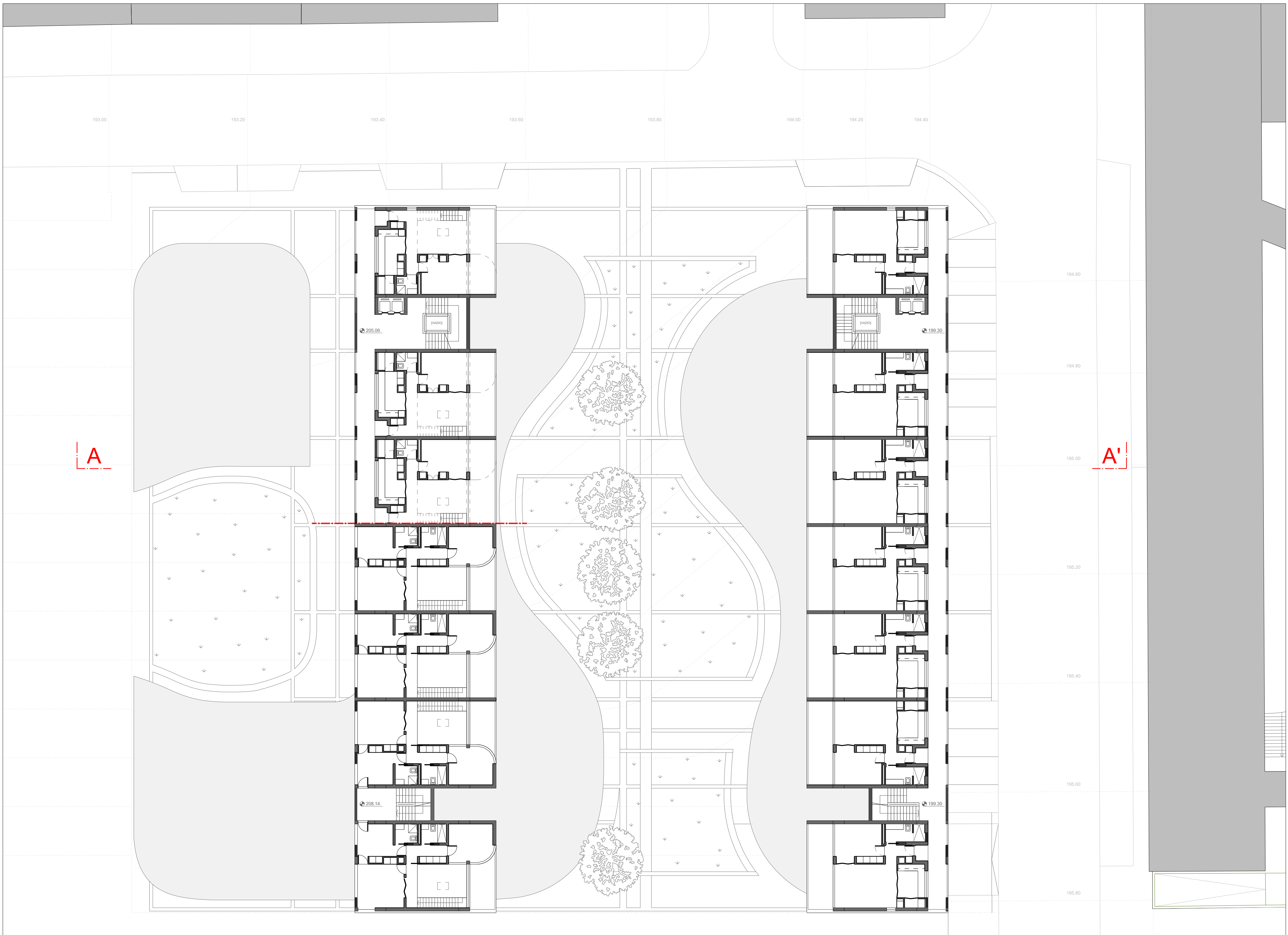
PLANTA PISO TIPO | VÁRIAS COTAS | N 0
