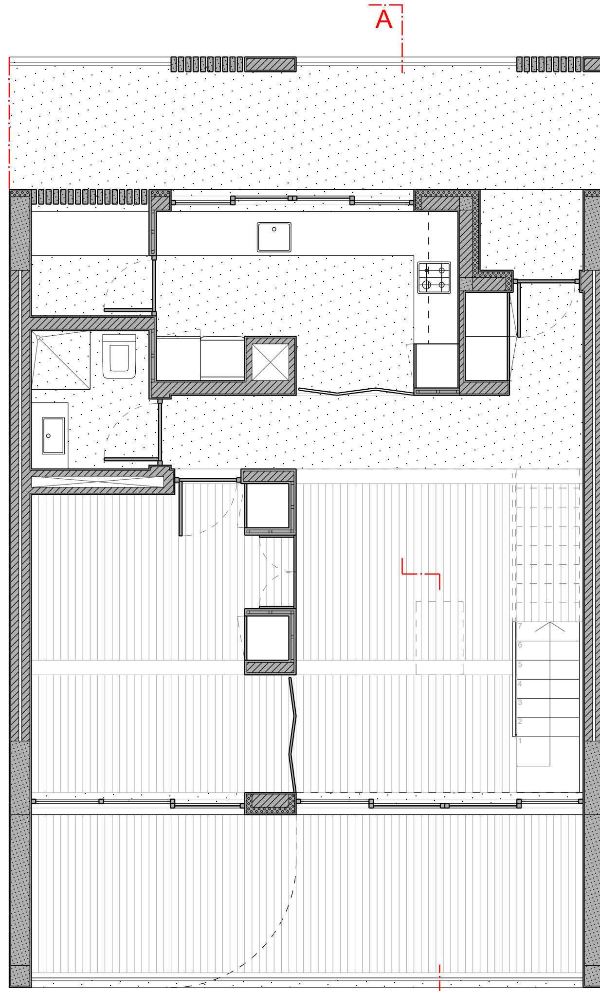
PLANTA FOGO GRANDE | PISO 0 [área 80m 2 ]
