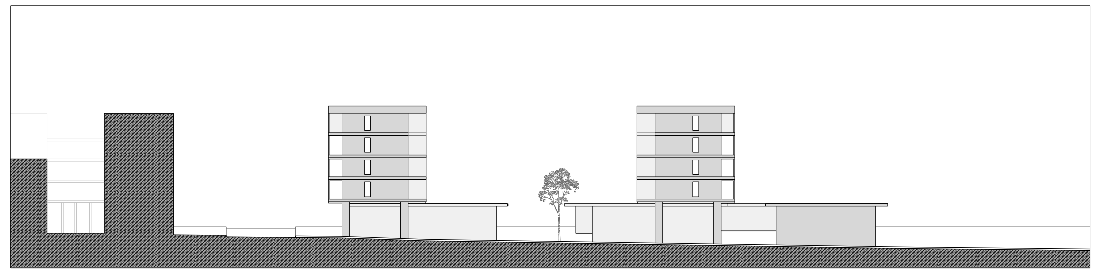
ALÇADO RUA BENTO DA COSTA
