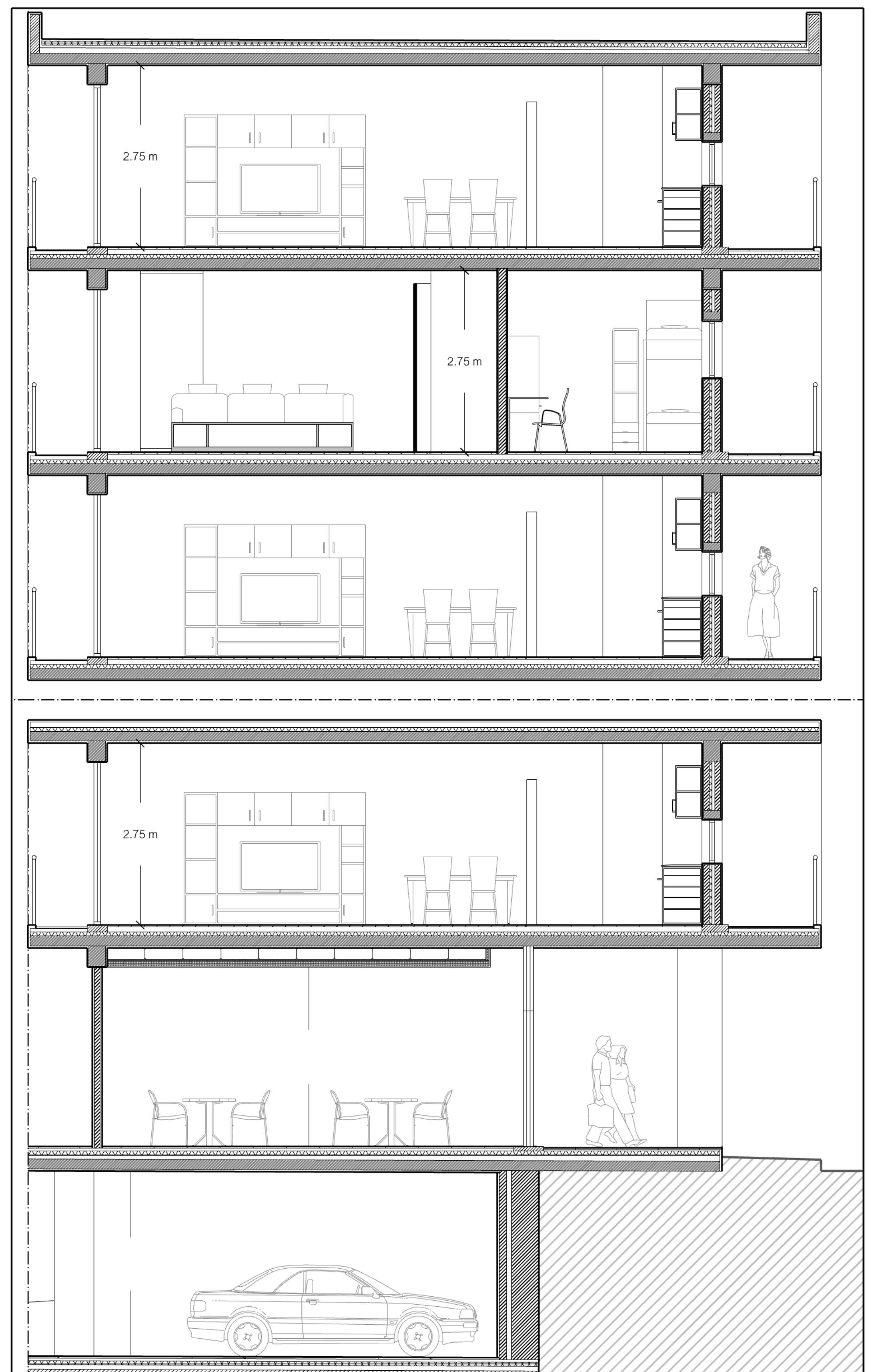
CORTE | ESC 1:50
