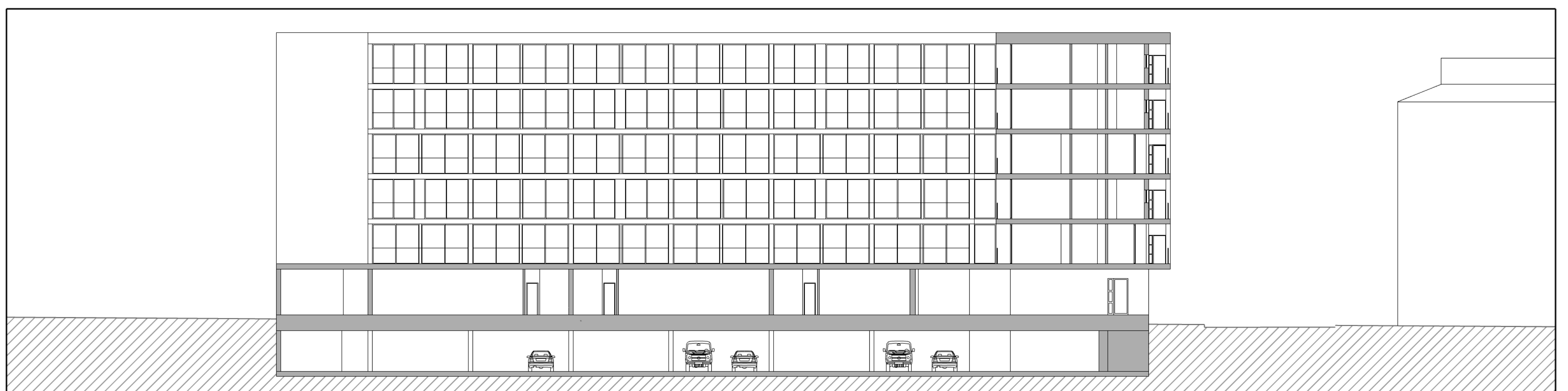
PERFIL BB'
