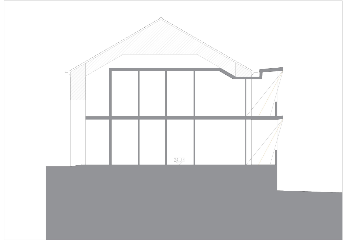
CORTE ESQUEMÁTICO PARA INTENÇÃO DE NOVA ADIÇÃO DE PALAS DE SOMBREAMENTO NA FACHADA SUL
