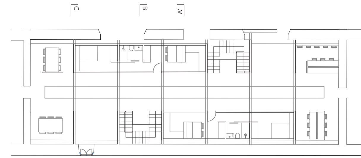
PLANTA PISO 0
