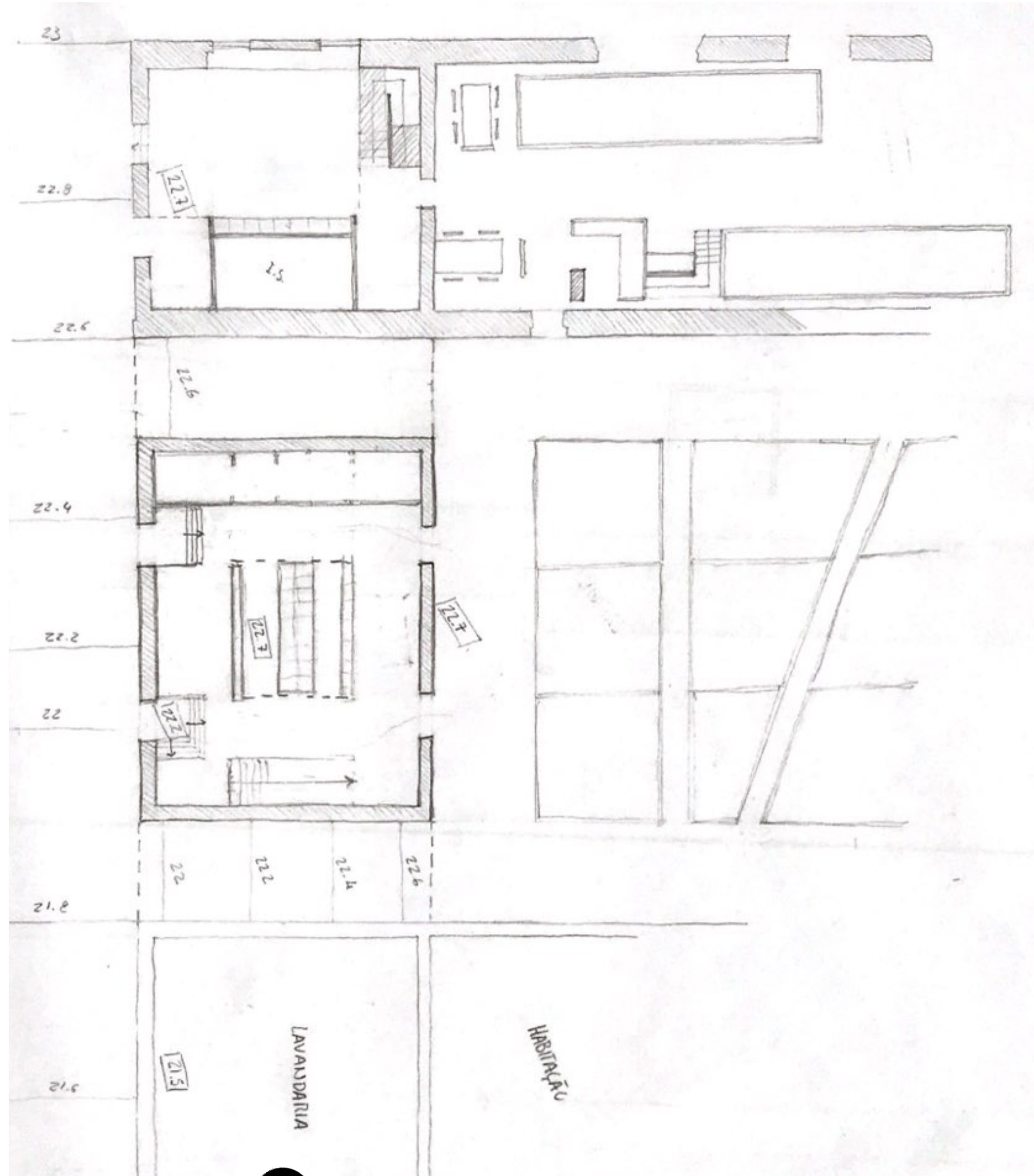
Piso 0 | esc. 1:200
