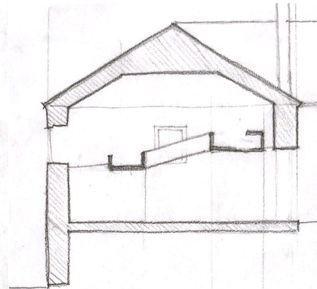
Corte AA' | esc. 1:200
