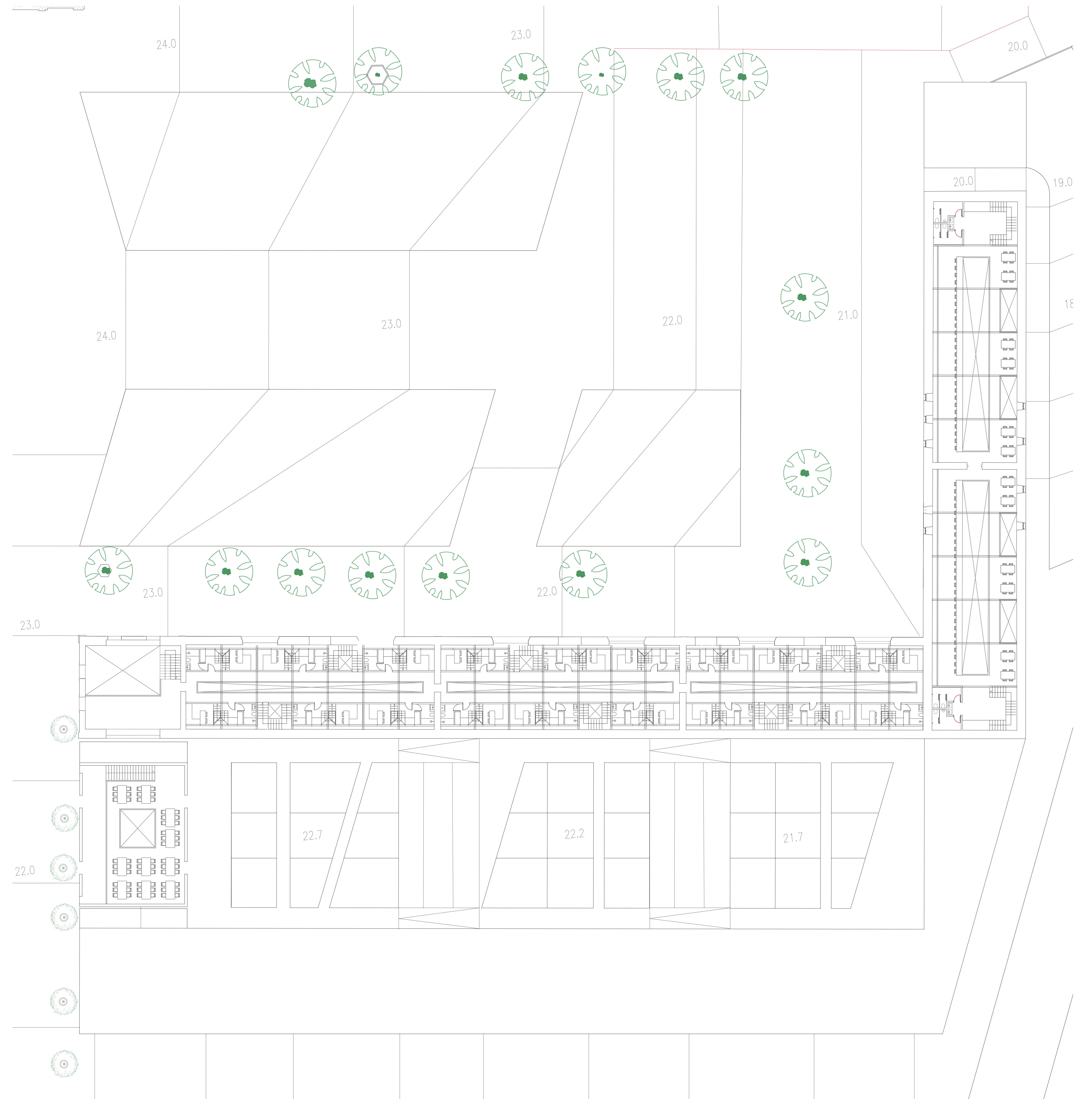
PLANTA CONJUNTO PISO 1 ESC. 1:200
