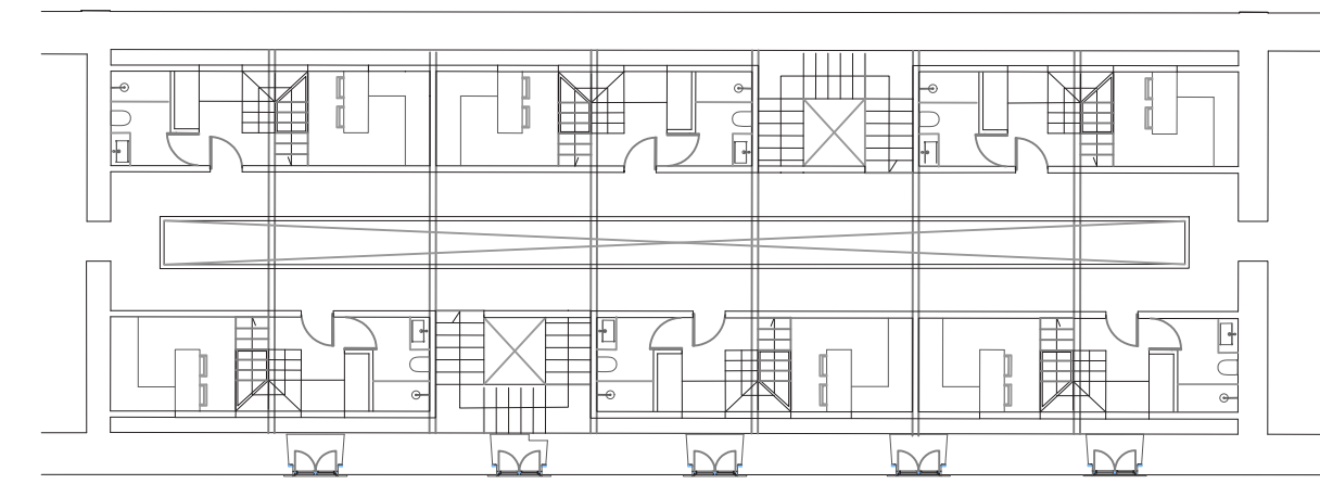
PLANTA PISO 1
