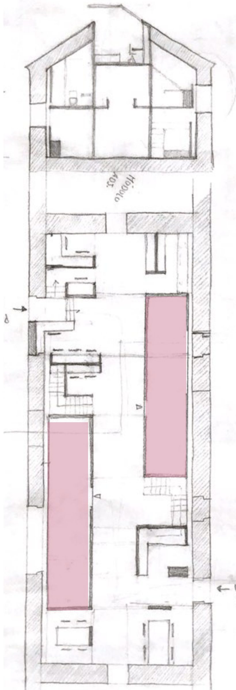
Piso 0 | esc. 1:200
