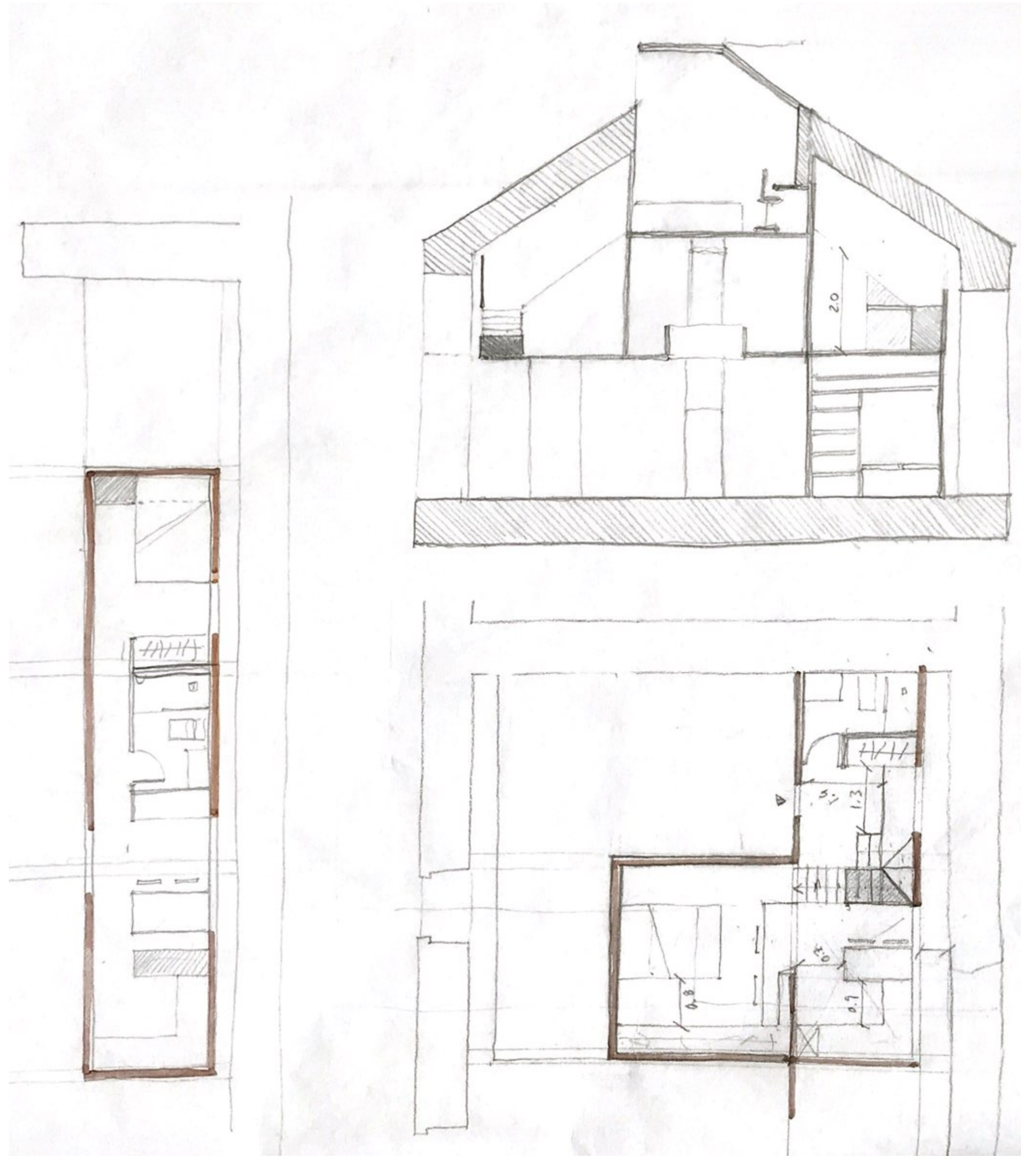
Micro casas | esc. 1:100
