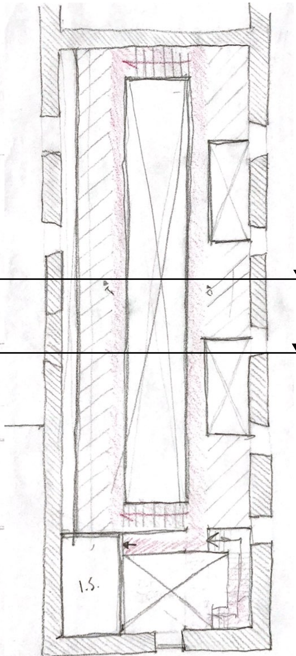
Piso 1 | esc. 1:200
