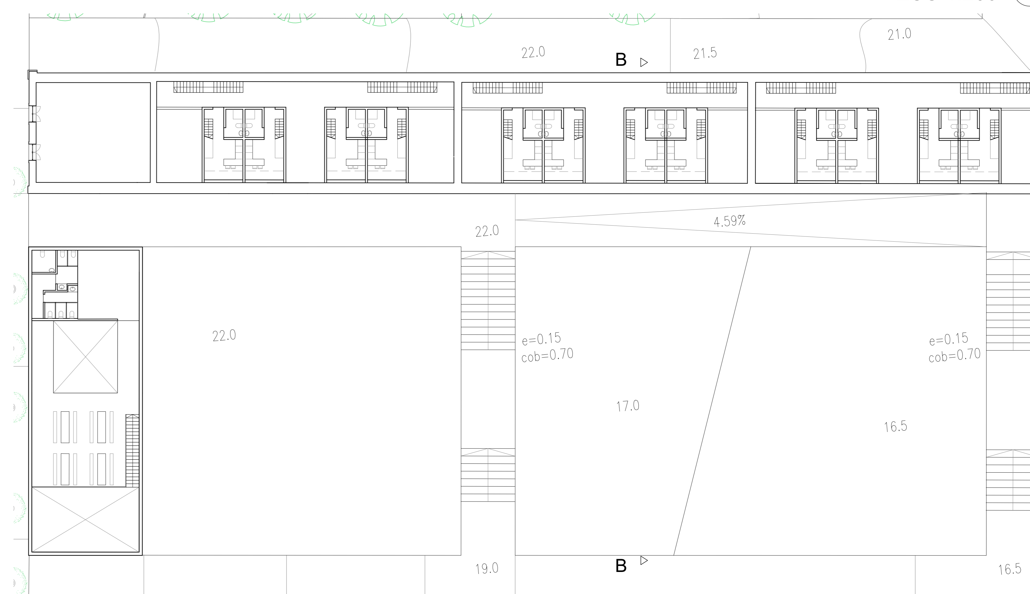
CO-LIVING PLANTA PIS0 1 ESC 1:200
