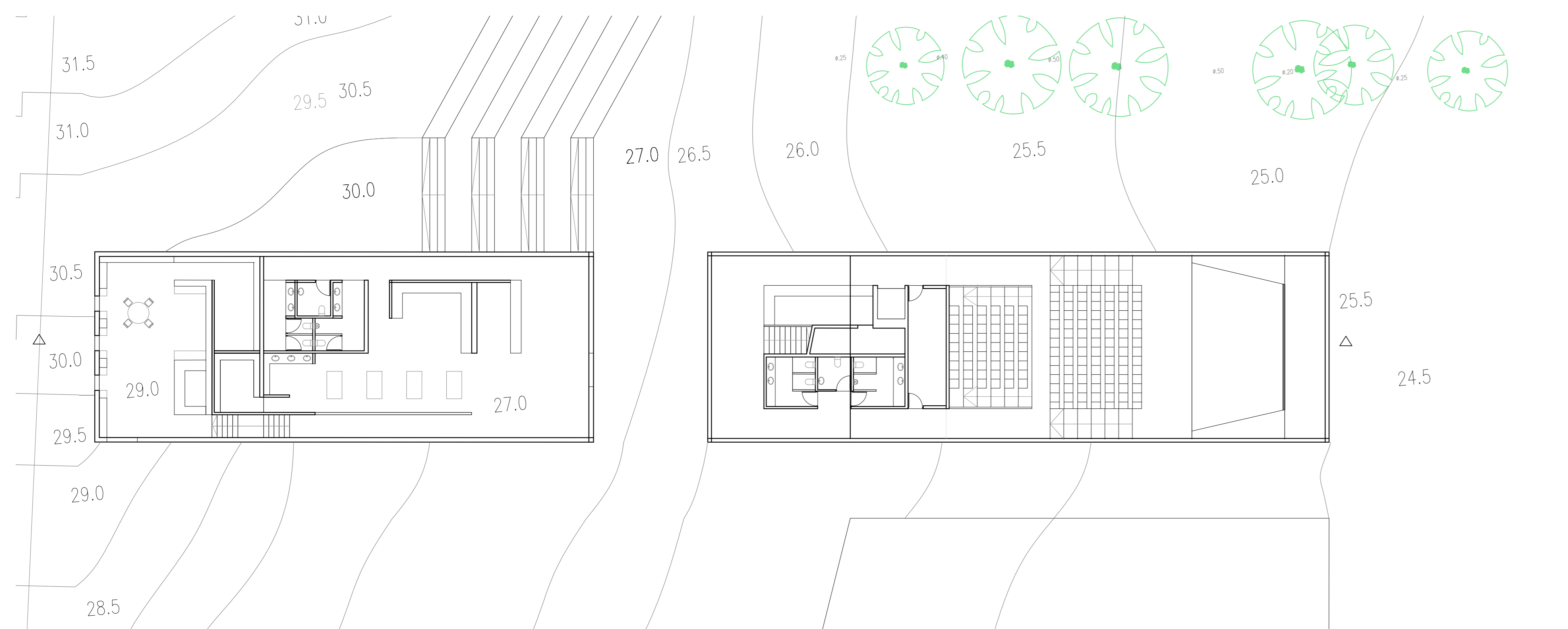
PLANTA PISO 0 LIVRARIA + OFICINA E AUDITÓRIO ESC 1:200
