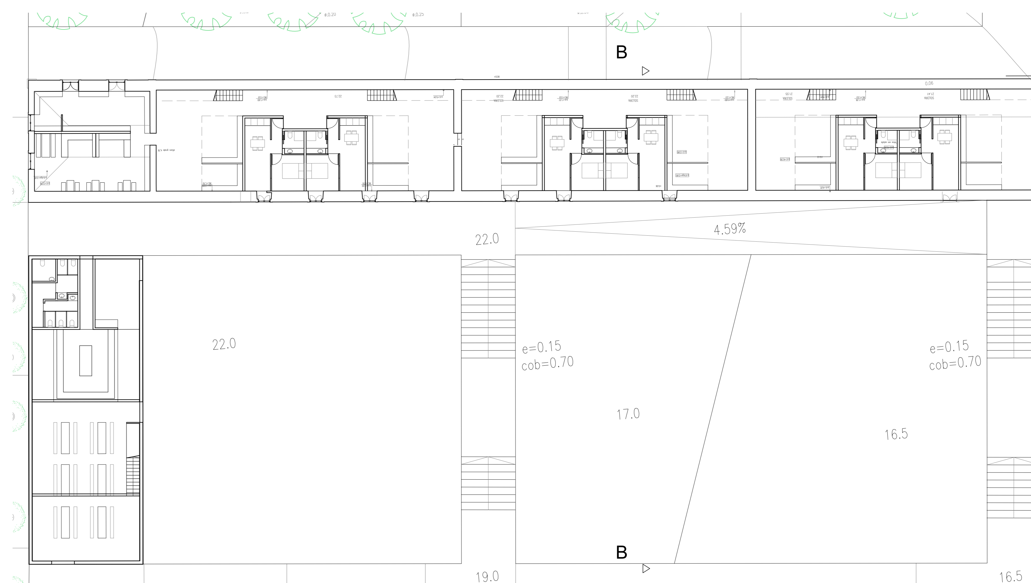
CO-LIVING PLANTA PIS0 0 ESC 1:200
