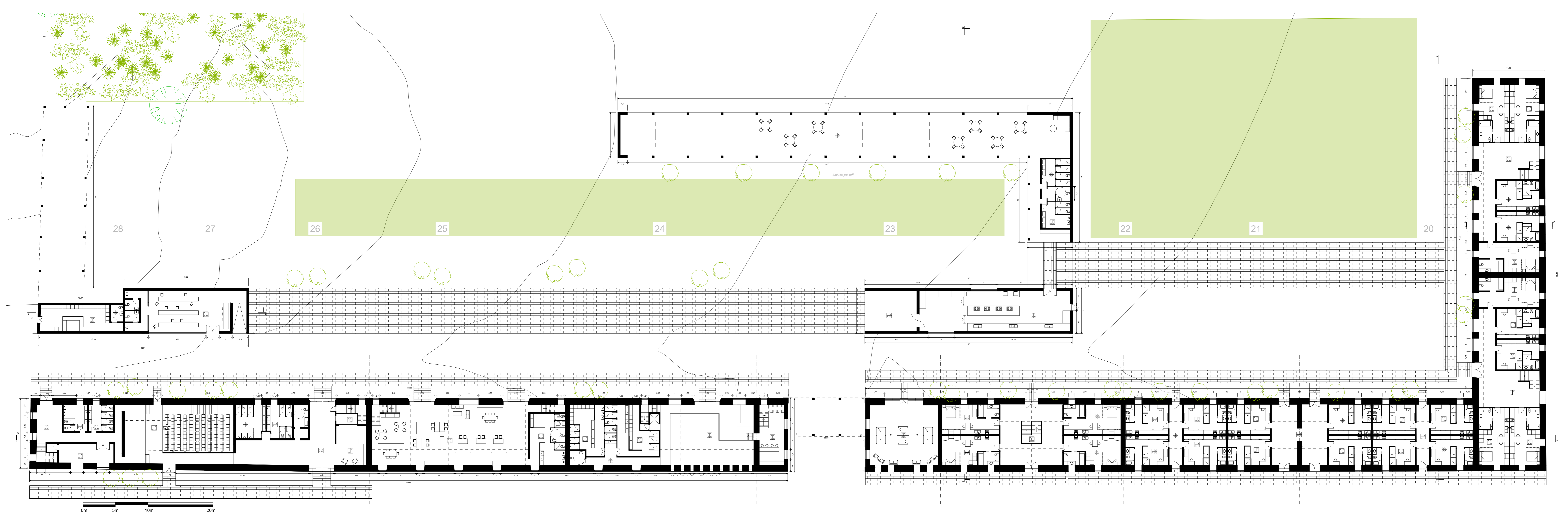
PLANTA PISO 0. ESCALA: 1/200
