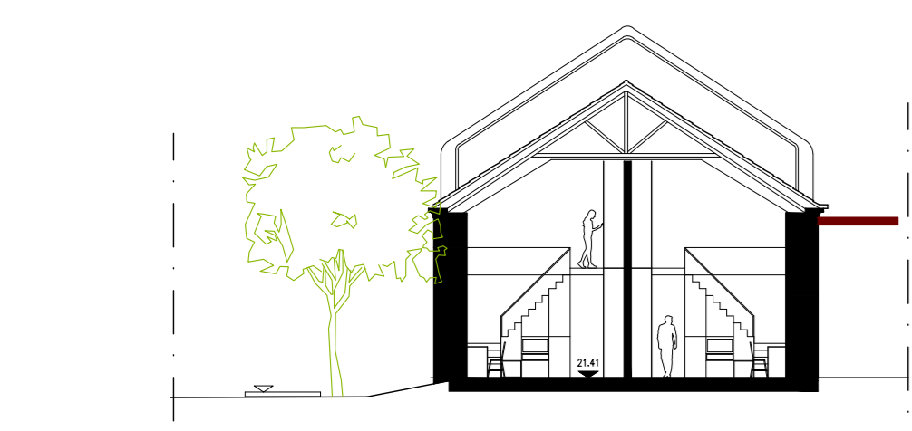
CORTE 4-4'. ESCALA: 1/200
