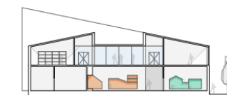
CORTE CC' : 1:200
