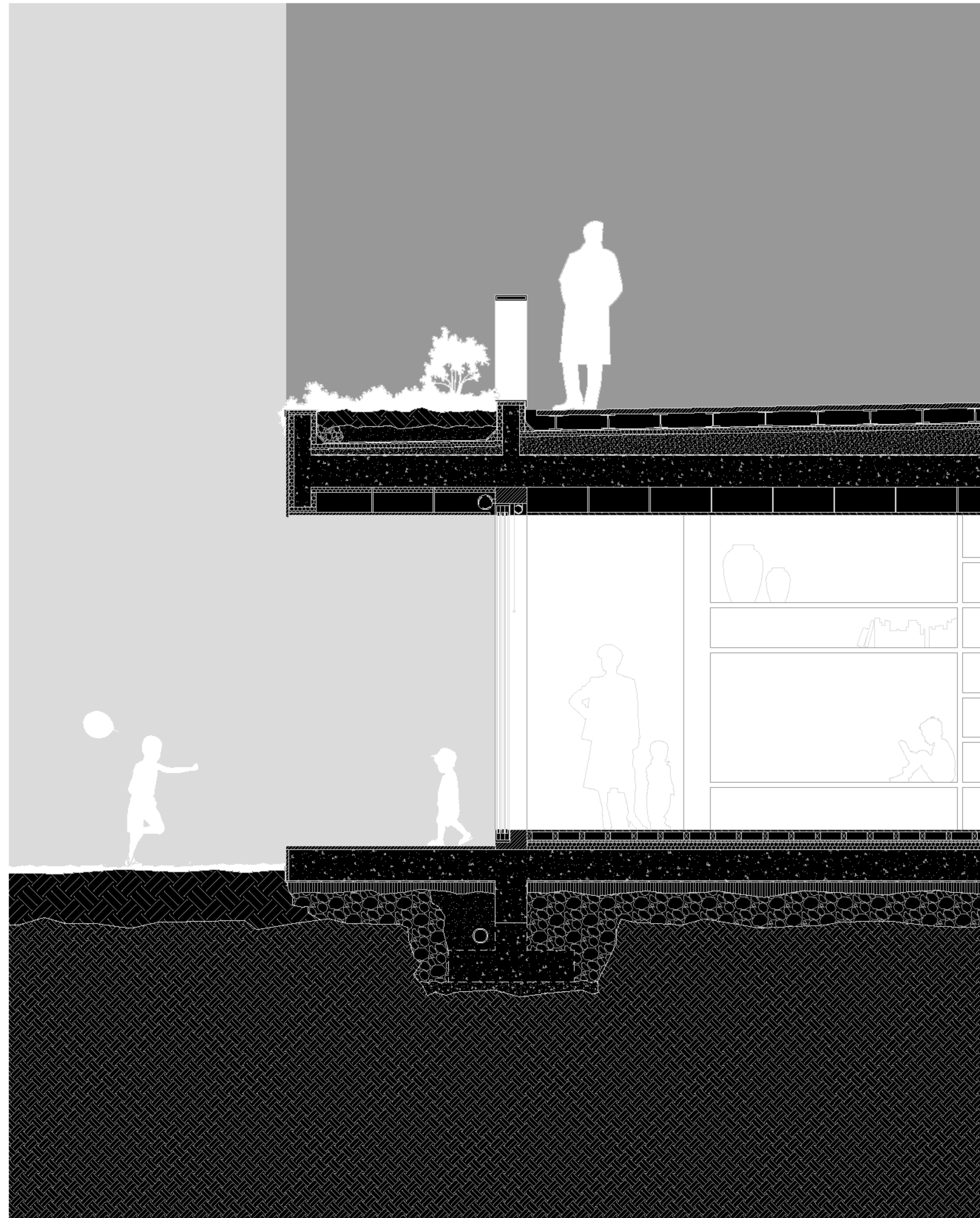
SECÇÃO PARCELAR CONSTRUTIVA 1/20
