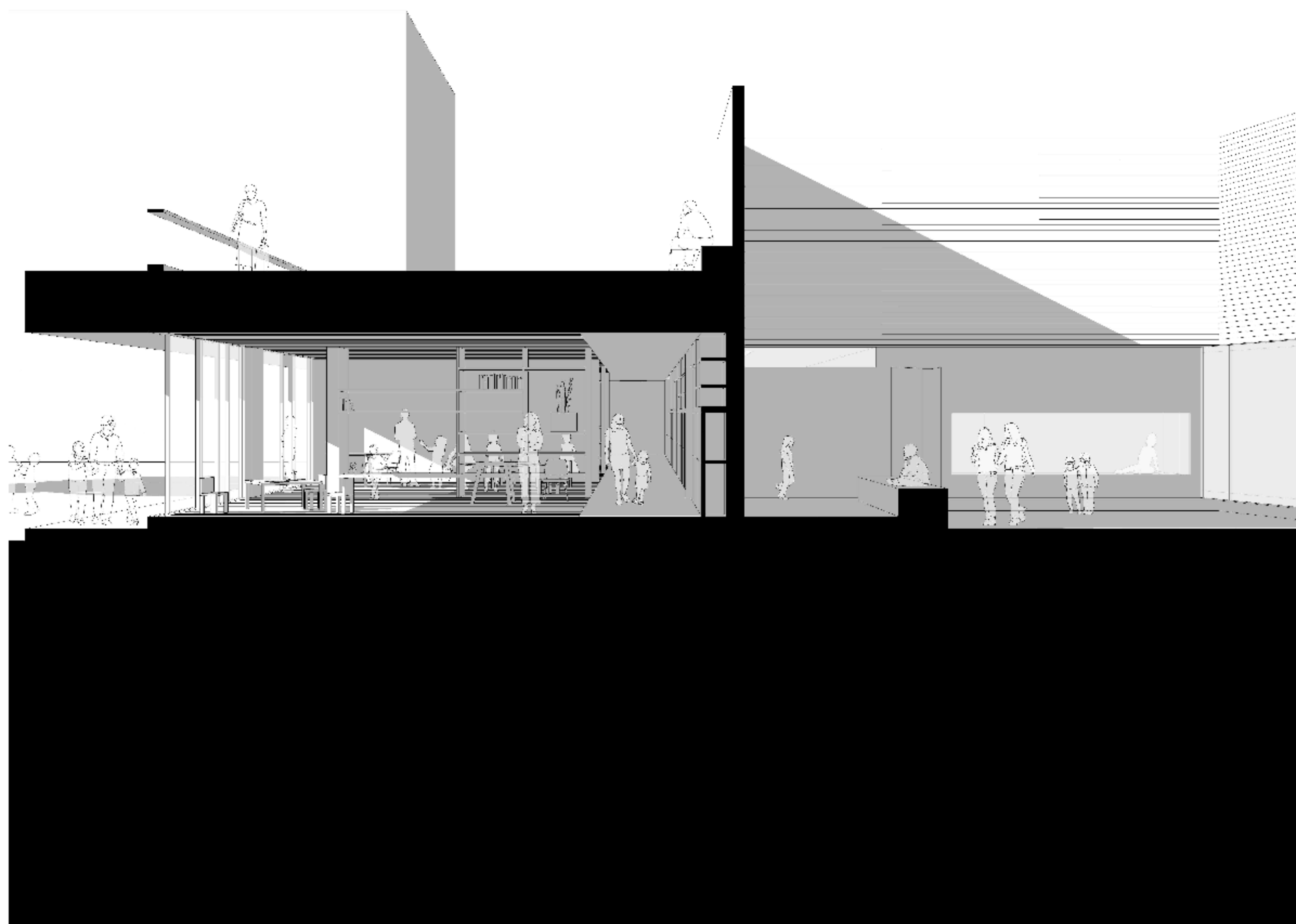
SECÇÃO PARCELAR 1/50
